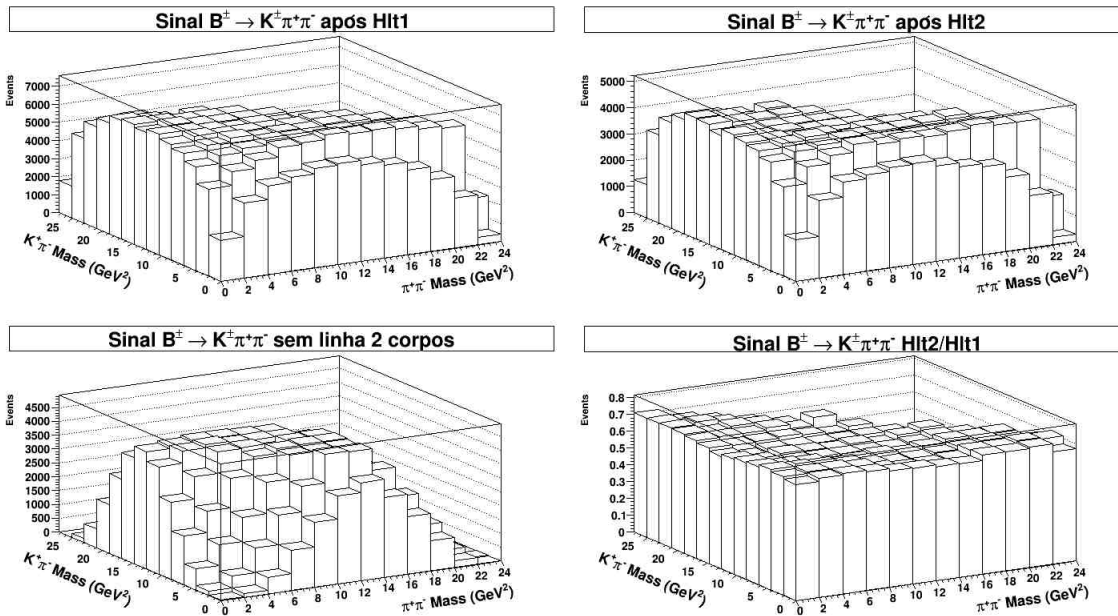
Figura 7.6: Dalitz Plot para o sinal de B^\pm \rightarrow K^\pm \pi^+ \pi^- . Alto Esquerda: Candidatos selecionados pelo Hlt1. Alto Direita: Candidatos selecionados pelo Hlt2. Baixo Esquerda: Candidatos selecionados apenas pela linha de três corpos do hádron topológico. Baixo Direita: Razão entre Hlt2 e Hlt1.
