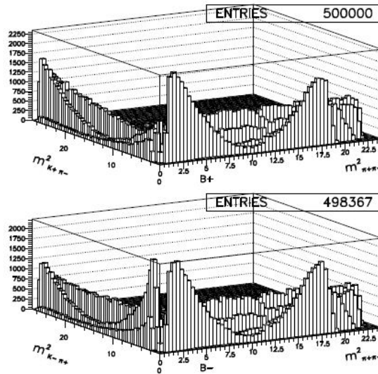
Figura 3.2: Dalitz Plot para B^+ e B^- gerados com assimetria de CP (próxima da origem).
