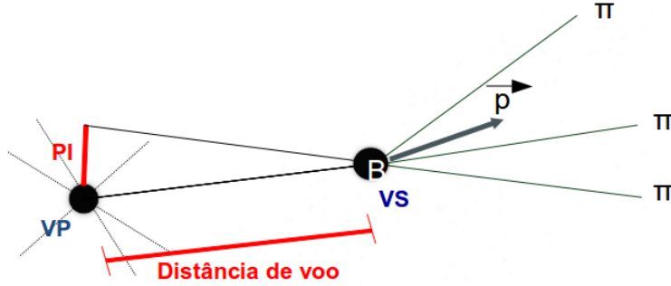
Figura 7.1: Topologia de um decaimento do méson B em três píons, onde as variáveis de parâmetro de impacto e de distância de voo estão ilustradas.
