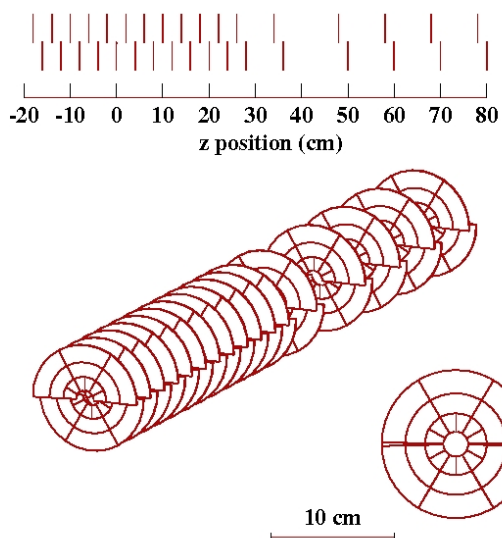
Figura 4.4: Geometria do VeLo. Ao todo são 34 semidiscos instalados ao redor da região de colisão para garantir que as partículas atravessassem pelo menos 3 deles.
