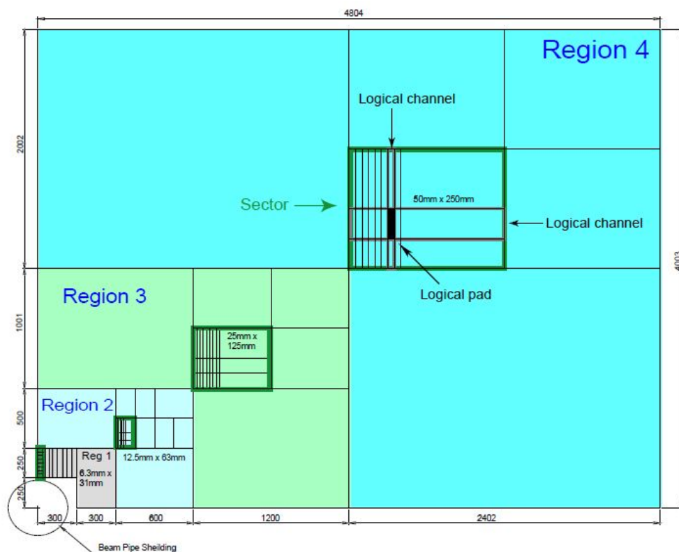
Figura 4.10: Visão frontal da estação M2 , mostrando a dimensão das regiões e das células que compõem cada câmara.
