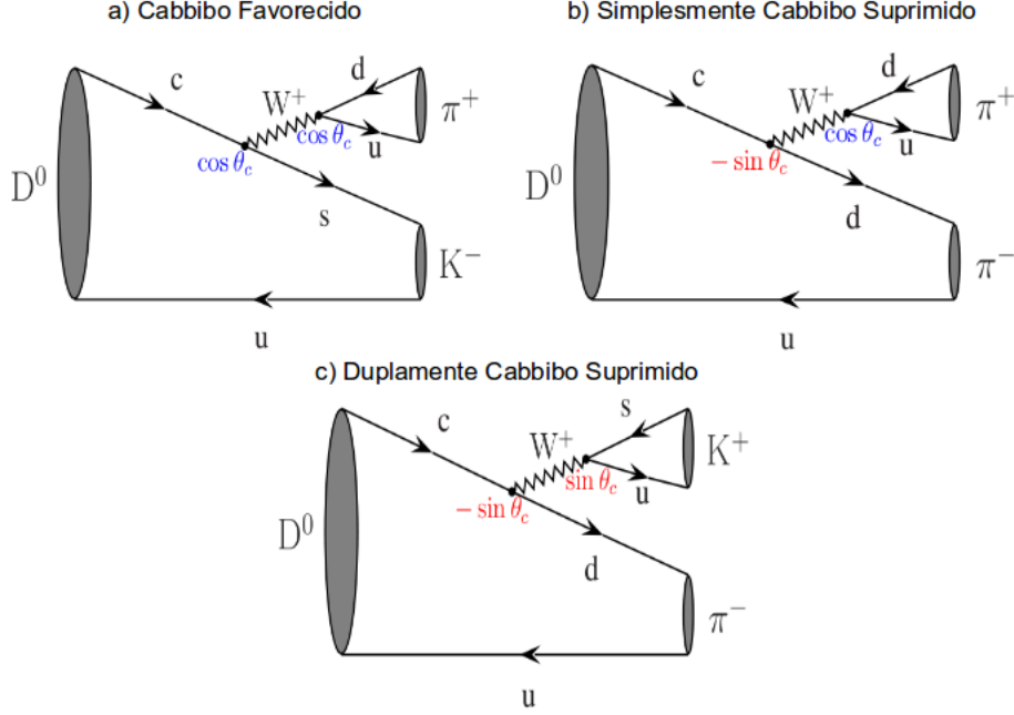
Figura 2.4: Diagramas representando três diferentes decaimentos do méson D^0 . Cada transição dos quarks envolvidos no processo dependem de \sin \theta_c ou \cos \theta_c , definindo o quão provável é tal decaimento.
