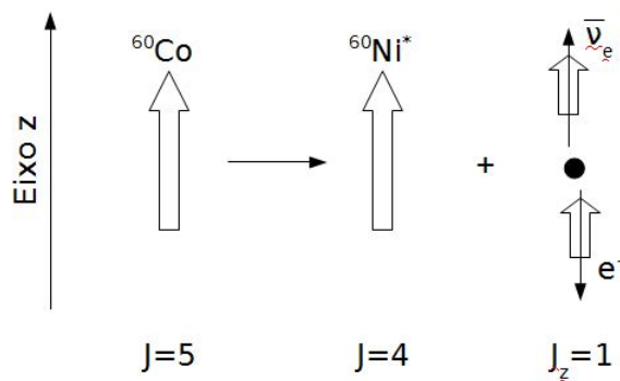
Figura 2.1: Experimento de decaimento do {}^{60}\text{Co} . O elétron emitido sempre está com momentum linear na direção oposta ao momentum angular revelando a violação de paridade para a interação fraca.
