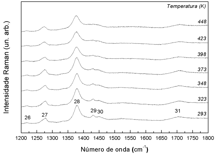
Figura 35: Espectro Raman não polarizado do KHT para o intervalo de temperatura 292–448 K, região espectral: 1200 a 1800 \text{cm}^{-1}
