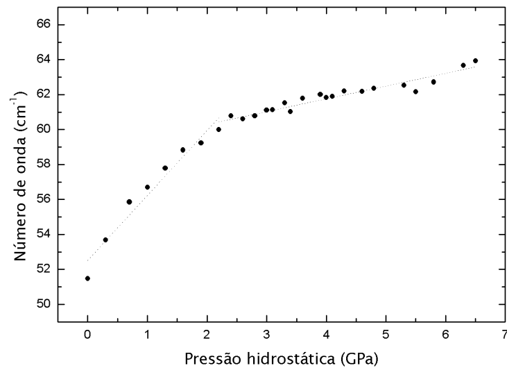
Figura 41: Número de onda do modo 1 (51 \text{cm}^{-1} ) em função da pressão hidrostática, intervalo de 0,0 a 6,5 GPa .
