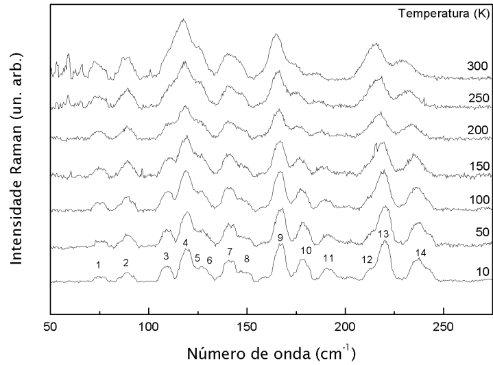
Figura 18: Espectro Raman não polarizado do KHT para o intervalo de temperatura 10–300 K, região espectral: 50 a 275 \text{cm}^{-1}
