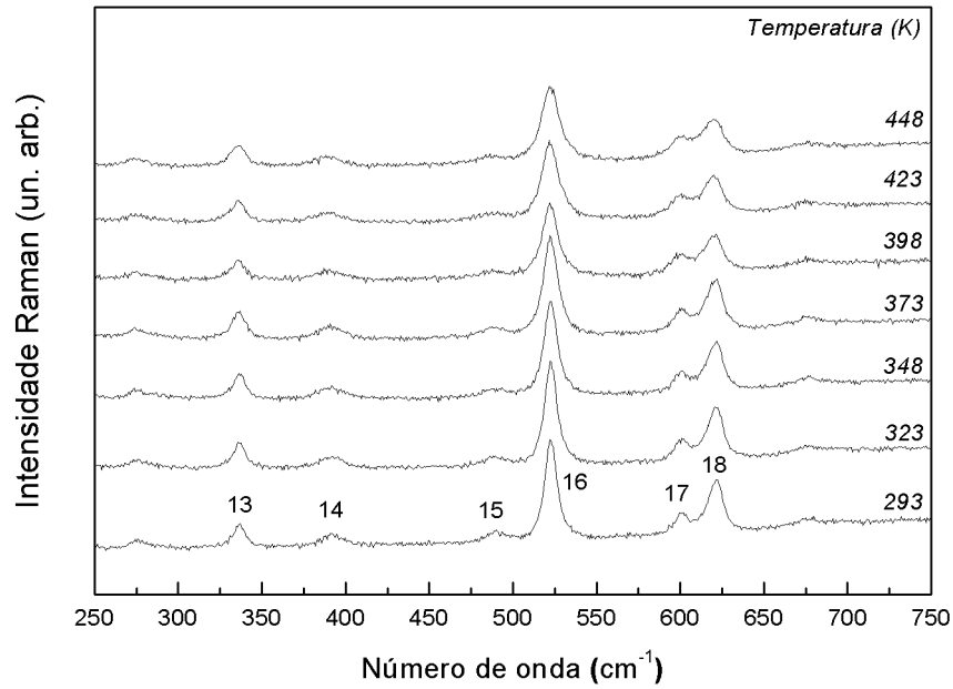
Figura 31: Espectro Raman não polarizado do KHT para o intervalo de temperatura 292–448 K, região espectral: 250 a 750 \text{cm}^{-1}
