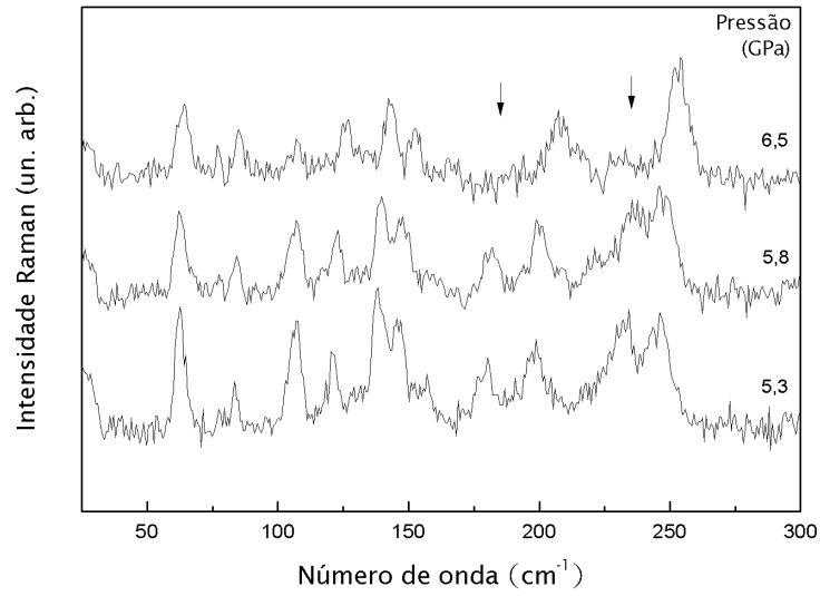
Figura 40: Espectro Raman não polarizado do KHT para o intervalo de pressão 5,3 GPa –6,5 GPa , região espectral: 25 a 275 \text{cm}^{-1}
