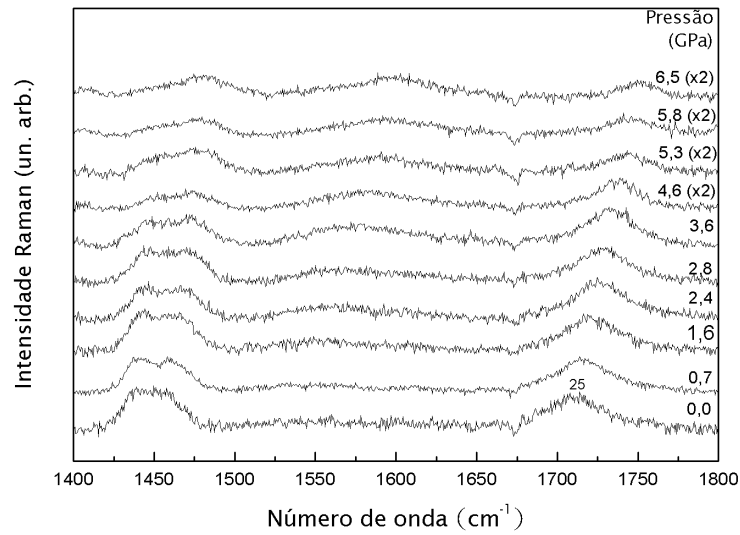
Figura 51: Espectro Raman não polarizado do KHT para o intervalo de pressão 0,0–6,5 GPa, região espectral: 1400 a 1800 \text{cm}^{-1}
