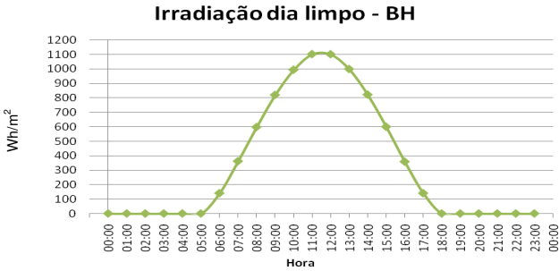
Figura 24 - Gráfico de um dia limpo para a cidade de Belo Horizonte. Fonte: Radiasol , 2009.
