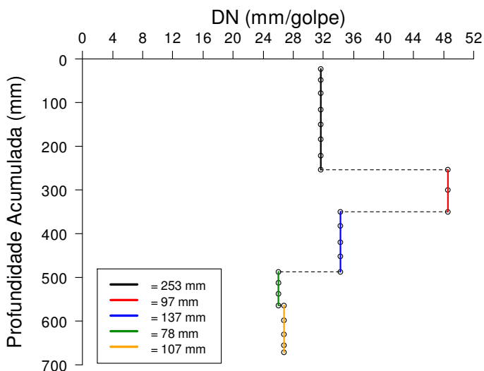
FIGURA 4.98 – Diagrama Estrutural do EX – Vala 8.
