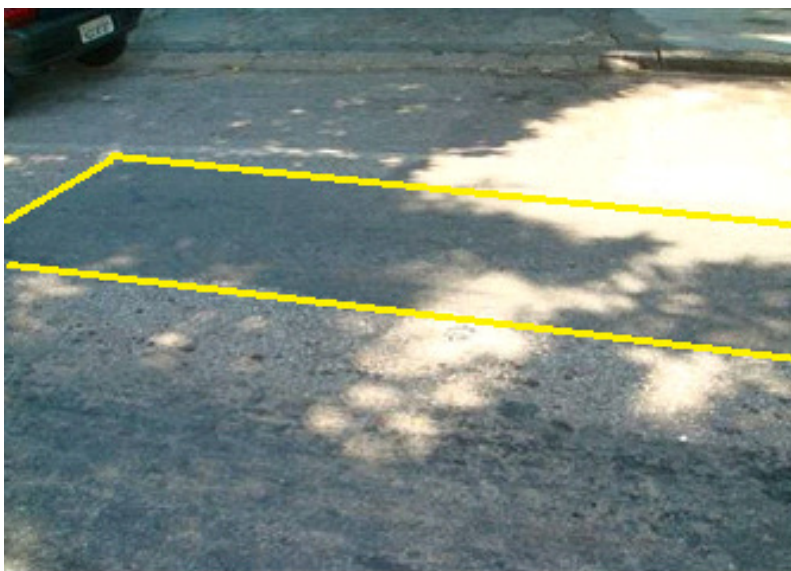
FIGURA 5.36 – Situação atual da vala 6 após dez meses de tráfego.
