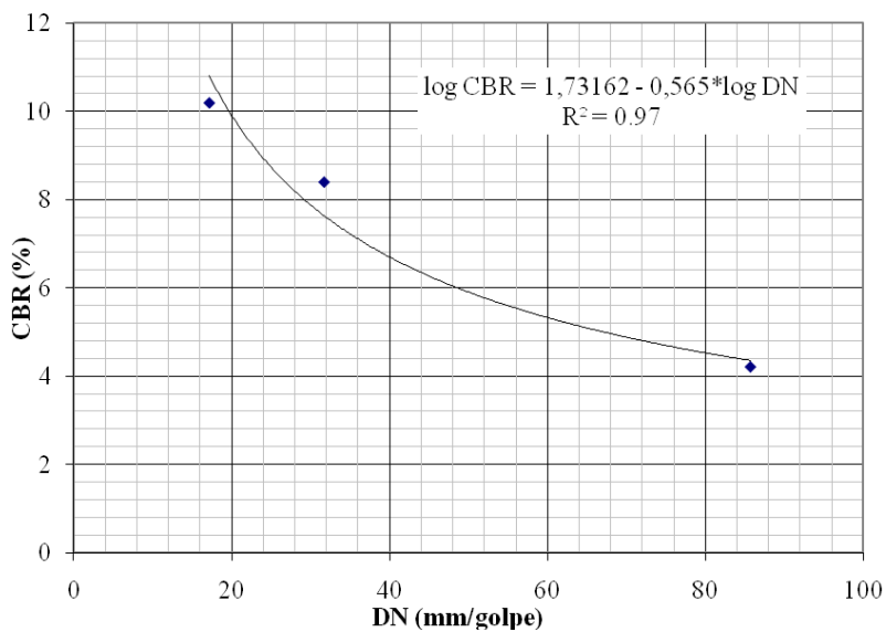
FIGURA 4.12 – Correlação CBR x DN - vala 2.
