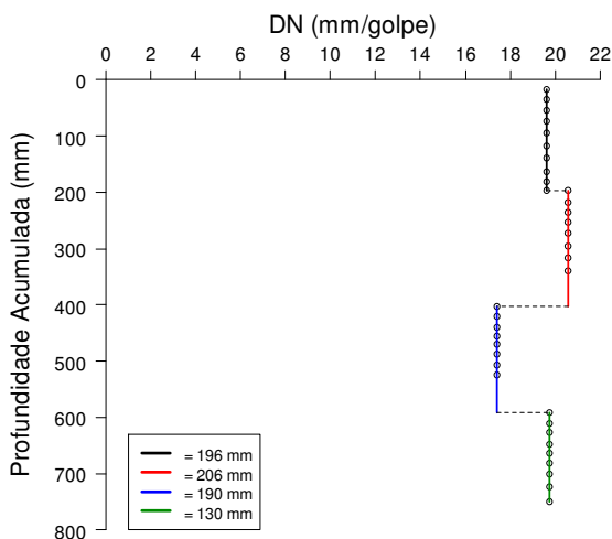
FIGURA 5.13 – Diagrama Estrutural por camada do EX – Vala Experimental 1
