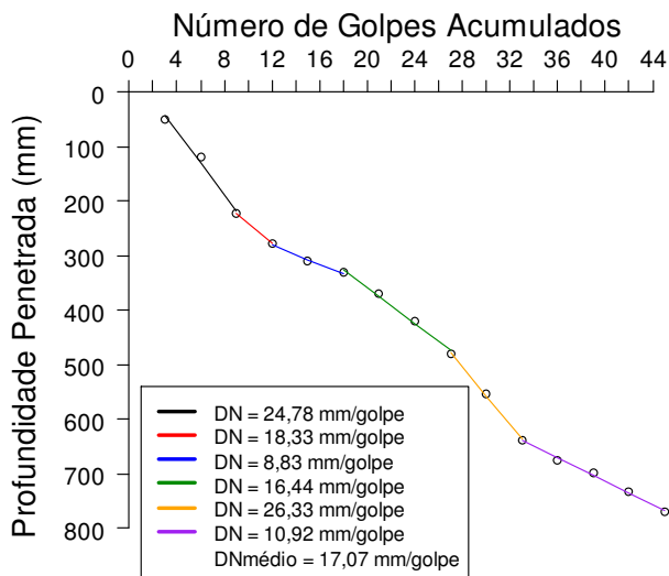
FIGURA 4.78 – Curva DCP do BD – Vala 6
