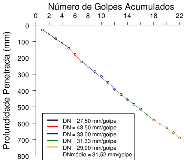
FIGURA 4.69 – Curva DCP do BD – Vala 5
