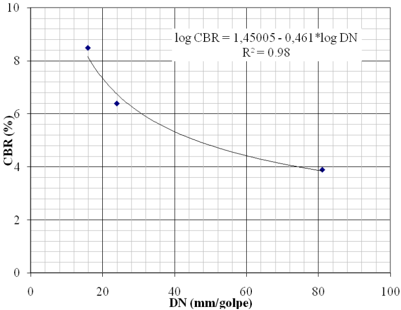
FIGURA 4.24 – Correlação CBR x DN - vala 8.
