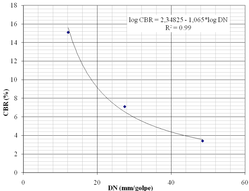
FIGURA 4.14 – Correlação CBR x DN - vala 3.
