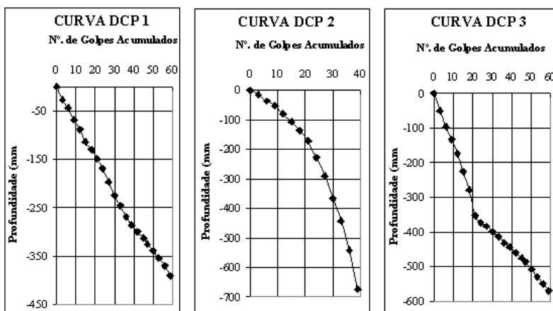
FIGURA 2.3 – Formato típico das Curvas DCP (Trichês e Cardoso, 2001).
