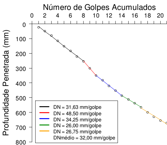
FIGURA 4.94 – Curva DCP do EX – Vala 8
