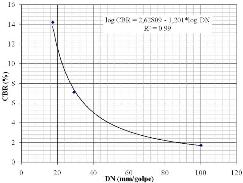
FIGURA 4.10 – Correlação CBR x DN - vala 1.
