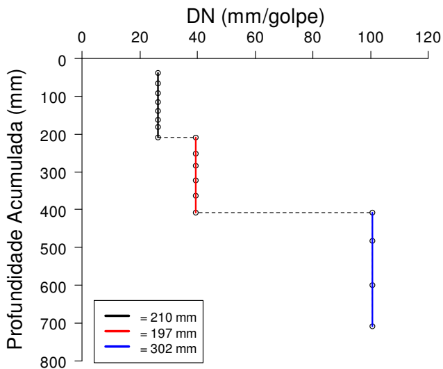
FIGURA 4.89 – Diagrama Estrutural do BE – Vala 7.
