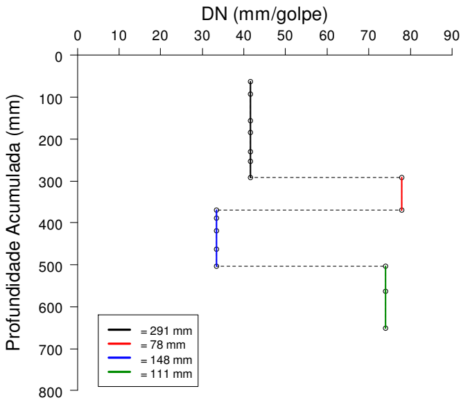
FIGURA 4.51 – Diagrama Estrutural do EX – Vala 3.
