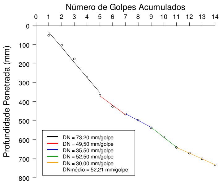
FIGURA 4.37 – Curva DCP do BE – Vala 2
