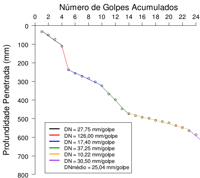
FIGURA 4.38 – Curva DCP do EX – Vala 2
