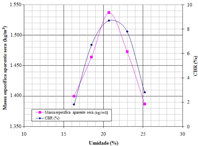
FIGURA 4.19 – Curvas de compactação e CBR - vala 6.
