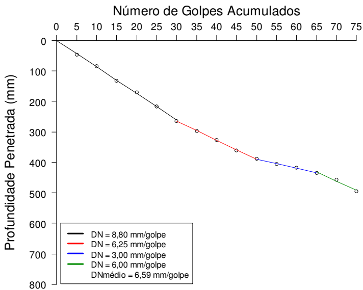
FIGURA 5.31 – Curva DCP do BD - Vala Exp. 2.
