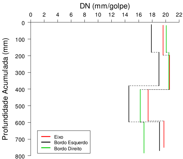
FIGURA 5.15 – Diagrama Estrutural por camada do BE, EX e BD – Vala Experimental 1.
