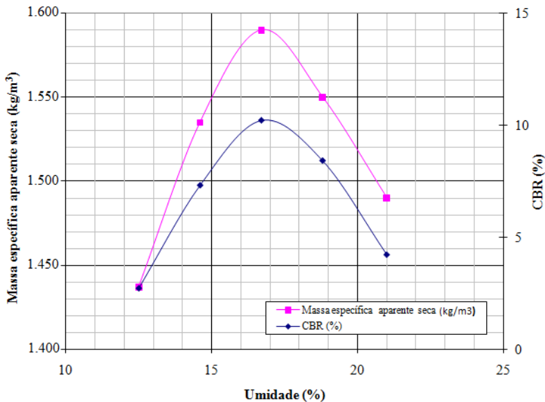
FIGURA 4.11 – Curvas de compactação e CBR - vala 2.
