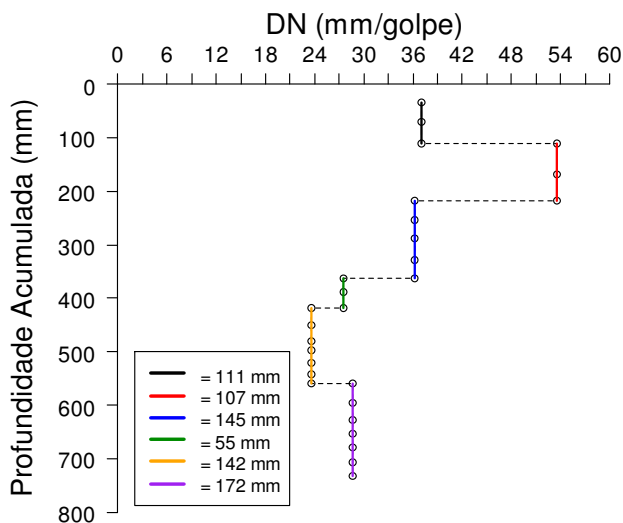
FIGURA 4.97 – Diagrama Estrutural do BE – Vala 8.
