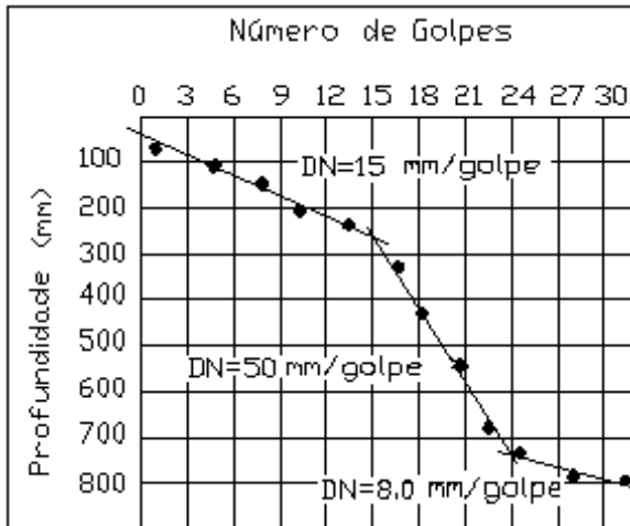
FIGURA 2.2 – Curva DCP, (Cardoso e Trichês, 1998).
