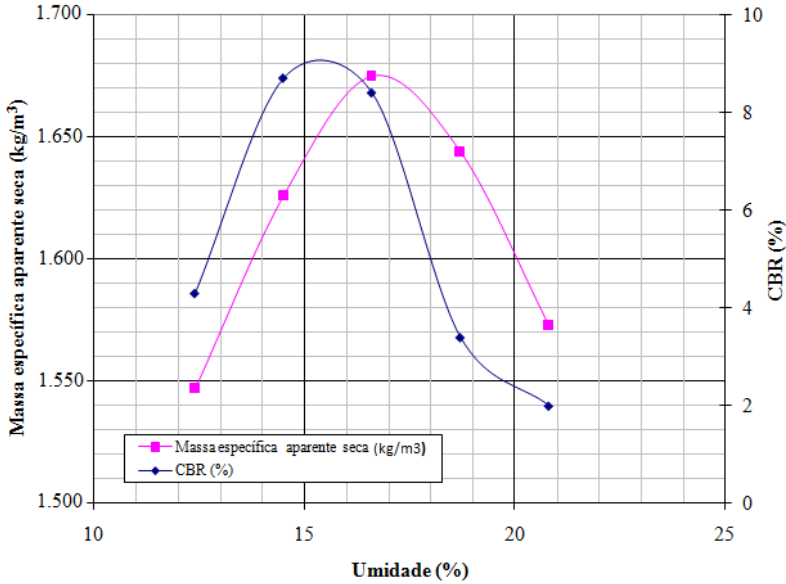
FIGURA 4.15 – Curvas de compactação e CBR - vala 4.
