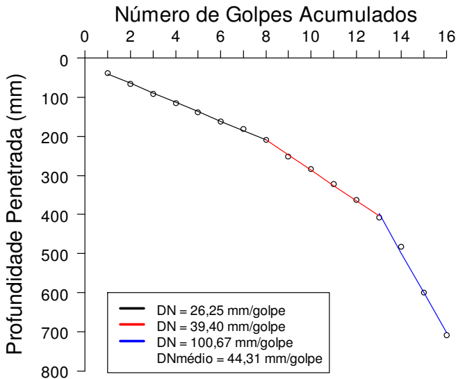
FIGURA 4.85 – Curva DCP do BE – Vala 7
