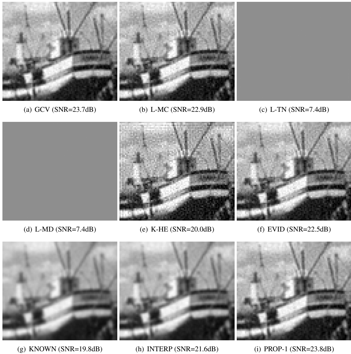
Figura 6.4: Exemplo visual mostrando a imagem 2 da seqüência Barco em outra realização, com alto ruído.
