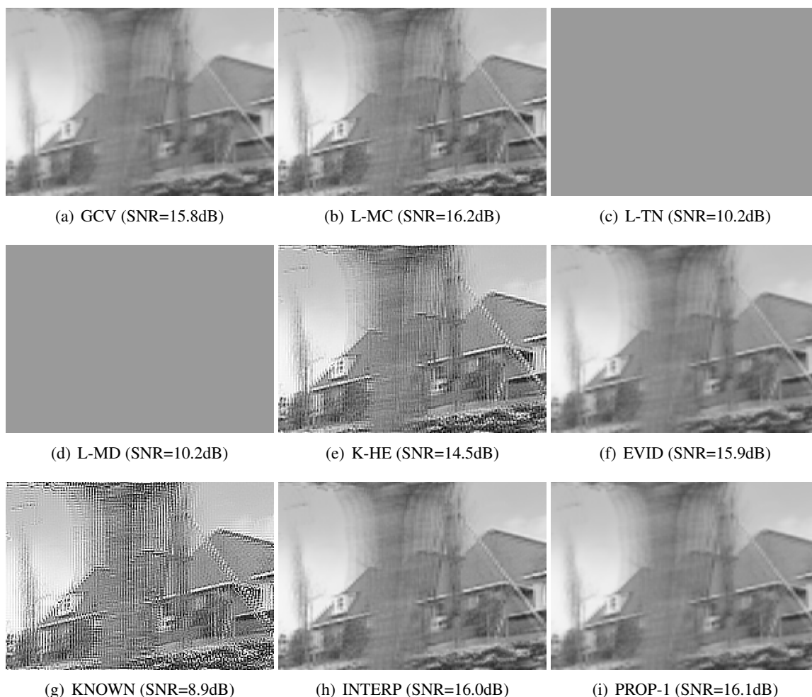
Figura 6.5: Exemplo visual mostrando a imagem 2 da seqüência Jardim, com baixo ruído.
