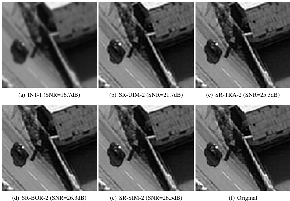
Figura 4.9: Exemplo visual mostrando a imagem 2 da seqüência Estrada, usando norma \ell_2 ao quadrado, modelos de segunda ordem e com detecção de outliers ativada .
