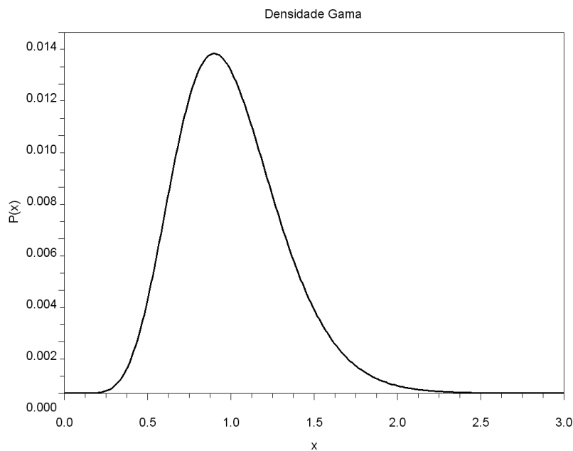
Figura 5.5: Densidade Gama, sugerida para os hiperparâmetros, com média 1 e variância 0.1.
