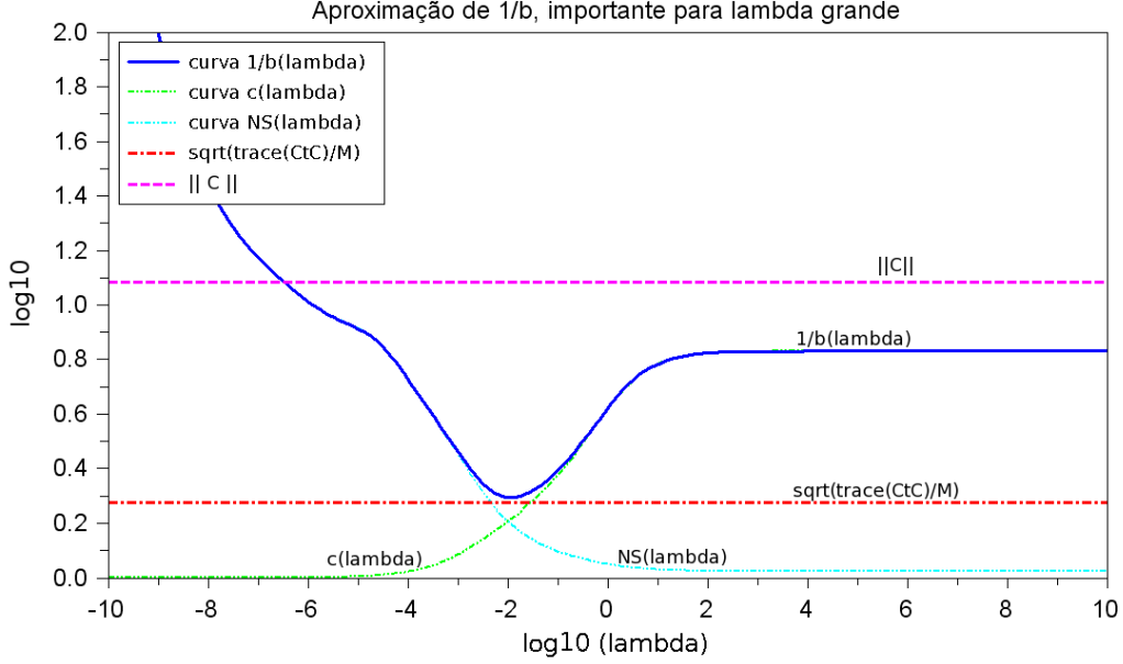
Figura C.1: Comportamento das curvas \frac{1}{b(\lambda)} , c(\lambda) e NS(\lambda) .
