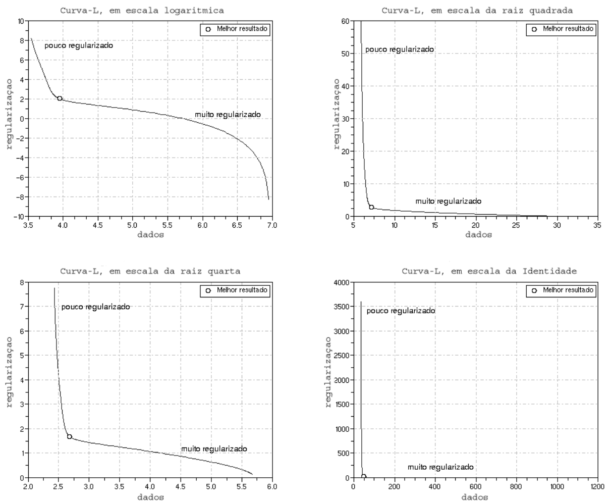
Figura 5.3: Curva-L em diversas escalas.
