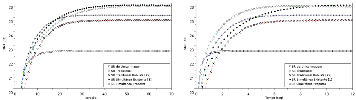
(a) Evolução do ganho em qualidade, através da SNR (dB), ao longo das iterações (b) Evolução do ganho em qualidade, através da SNR (dB), ao longo do tempo, em segundos
