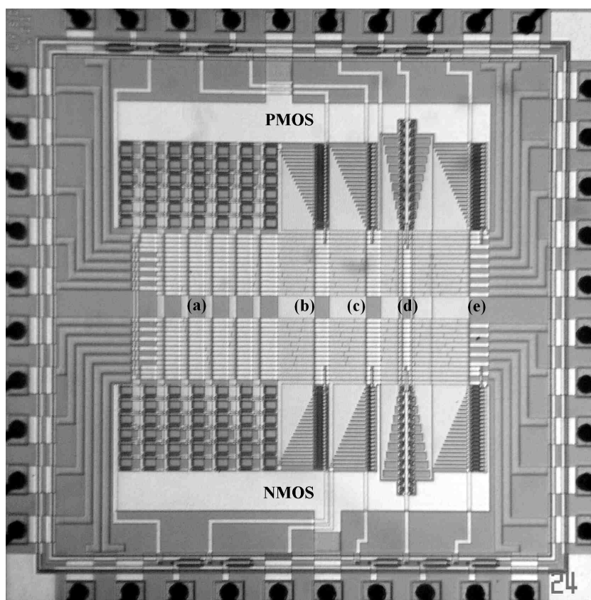
Figura 4.5: Microfotografia da primeira versão do circuito de teste, implementado na tecnologia AMIS 1,5 \mu\text{m} . É formado por cinco arranjos de geometrias diferentes: (a) grande, (b) curto, (c) pequeno, (d) médio e (e) estreito. Os arranjos são replicados em transistores NMOS e PMOS .
