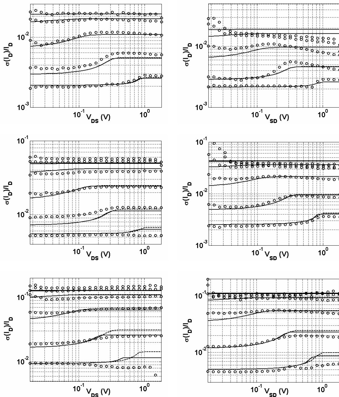
Figura 4.23: Descasamento dos grupos 16x16 (4,8 \mu\text{m} / 3,2 \mu\text{m} - cima), 16x04 (4,8 \mu\text{m} / 0,8 \mu\text{m} - centro) e 16x01 (4,8 \mu\text{m} / 0,2 \mu\text{m} - baixo), NMOS (esq.) e PMOS (dir.) na tecnologia TSMC 0.18 . Círculos (o): medidas; linhas sólidas (—): modelo com ESVP; linhas segmentadas (---): modelo sem ESVP. As curvas representam respectivamente, de cima para baixo, os níveis de inversão: 0,01; 0,1; 1; 10; 100 e 1000. No grupo 16x16 o nível de inversão 0,01 não está representado.
