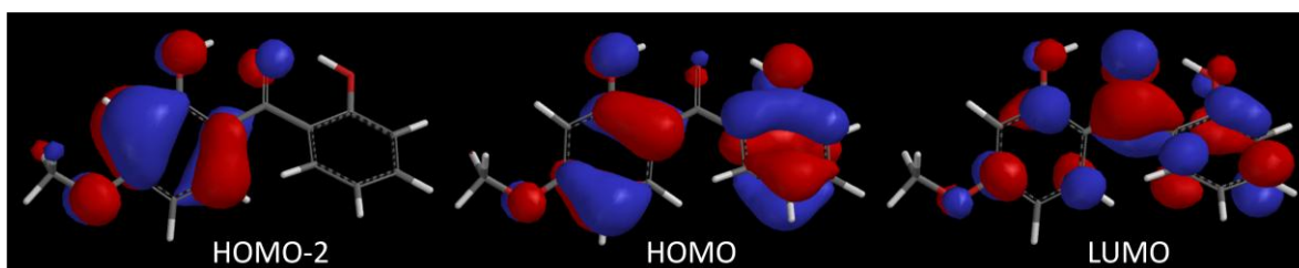
Figura 45. Coeficientes do orbitais de HOMO-2, HOMO e LUMO do derivado 14 .
