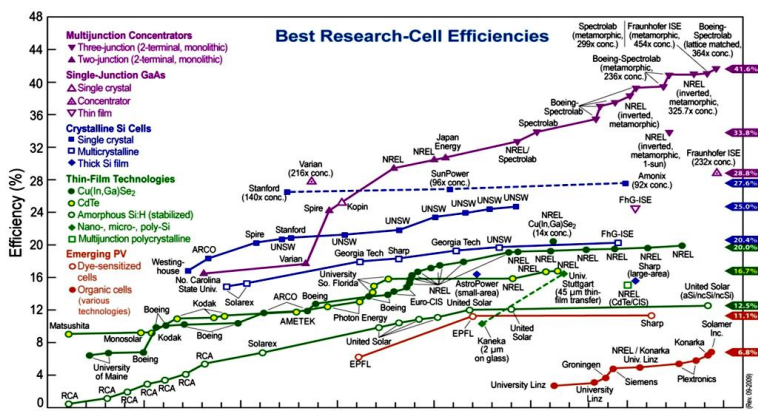
Figura 2.21 - Evolução da eficiência de conversão de células fotovoltaicas.
