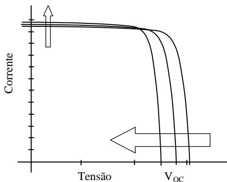
Figura 2.26 – Efeitos (indicados pelo sentido das setas) do aumento da temperatura de uma célula: grande diminuição na tensão de circuito aberto e ligeiro aumento na corrente.
