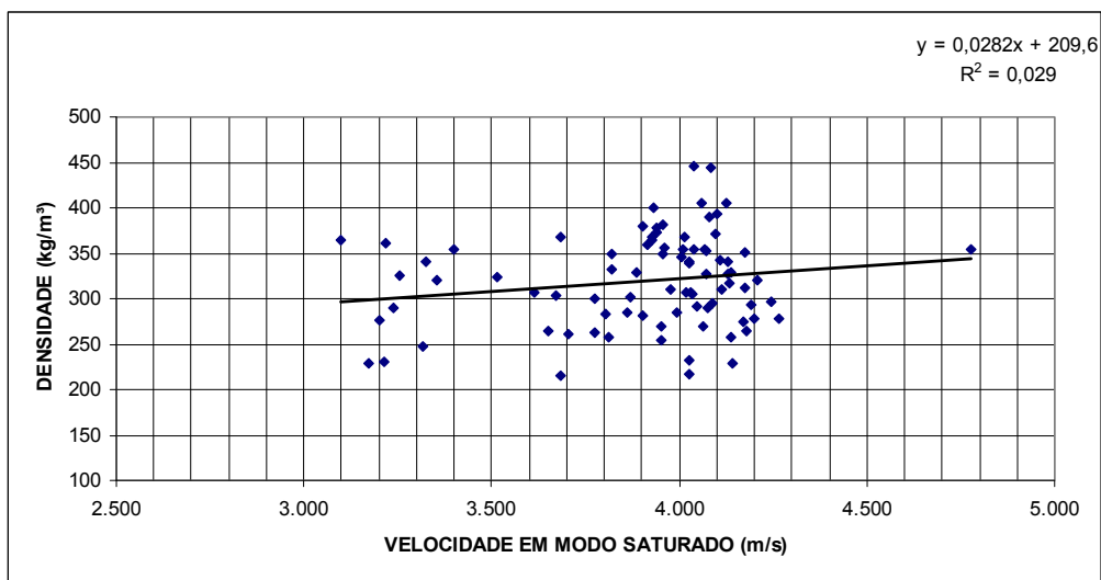
Figura 76 - Correlação entre densidade e velocidade de propagação longitudinal no modo saturado para todos os lotes.
