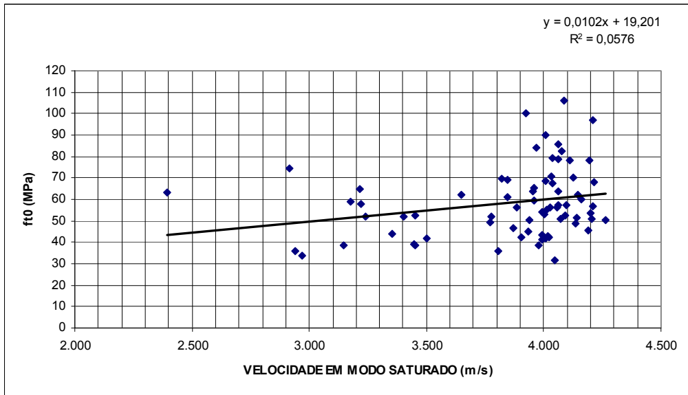
Figura 82 - Correlação entre tração paralela às fibras e velocidade de propagação longitudinal no modo saturado para todos os lotes.
