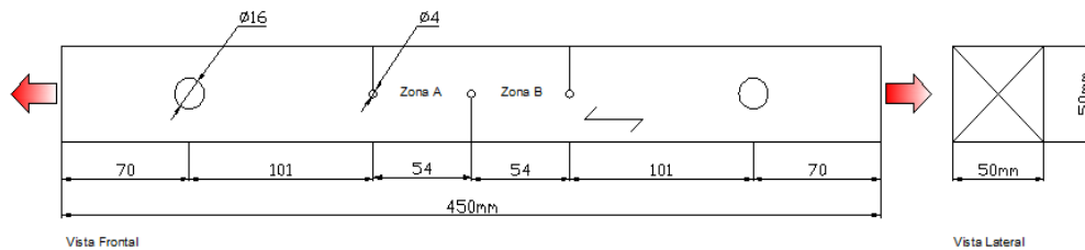
Figura 35 - Sistema de forças e dimensões do corpo de prova para o teste de cisalhamento adaptado.
