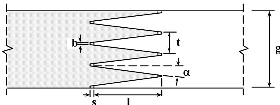
Figura 4 – Emenda por entalhes múltiplos: b – espessura da extremidade de um dente; g – largura total da emenda; l – comprimento dos entalhes; s – folga do fundo da emenda; t – passo dos dentes; e \alpha – inclinação da fase do dente. Adaptado de Szücs (1992).
