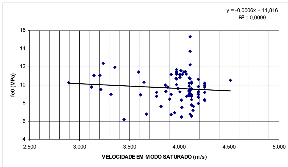
Figura 86 - Correlação entre embutimento paralelo às fibras e velocidade de propagação longitudinal no modo saturado para todos os lotes.
