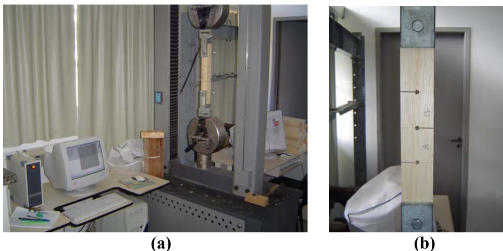
Figura 38 - Máquina Universal de Ensaio Kratos®: (a) ensaio de cisalhamento; e (b) detalhe do corpo de prova de cisalhamento.
