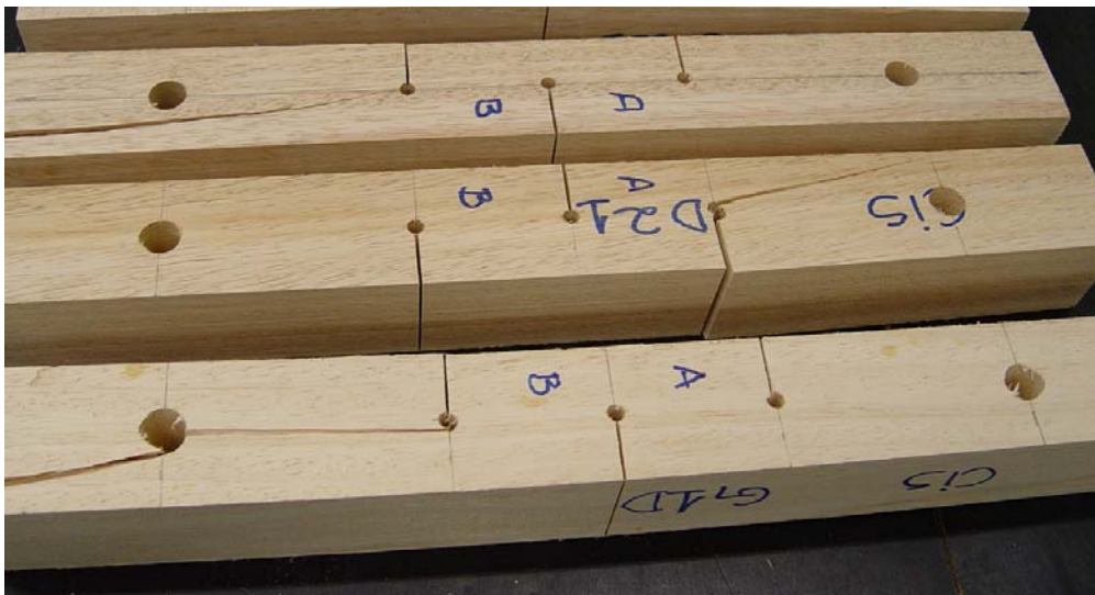
Figura 36 - Modos de ruptura não desejada em corpos de prova de cisalhamento adaptados da NF B 5-32.
