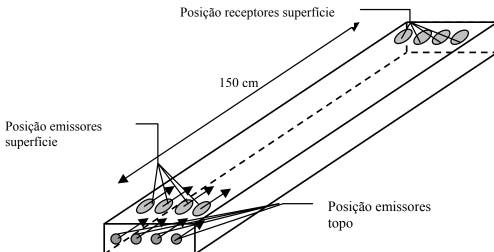
Figura 27 – Esquema do posicionamento dos transdutores emissores e receptores de ultrassom.
