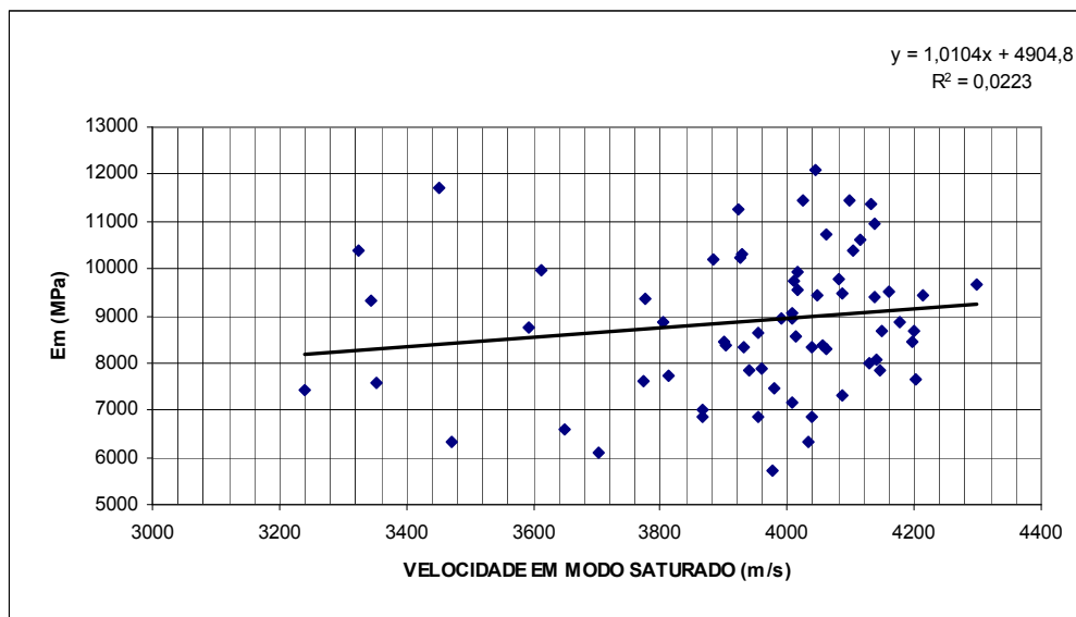
Figura 80 - Correlação entre módulo de elasticidade à flexão e velocidade de propagação longitudinal no modo saturado para todos os lotes.
