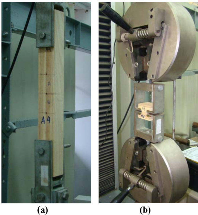
Figura 47 – Testes de resistência da linha de cola (a) teste de cisalhamento e (b) teste de tração normal.
