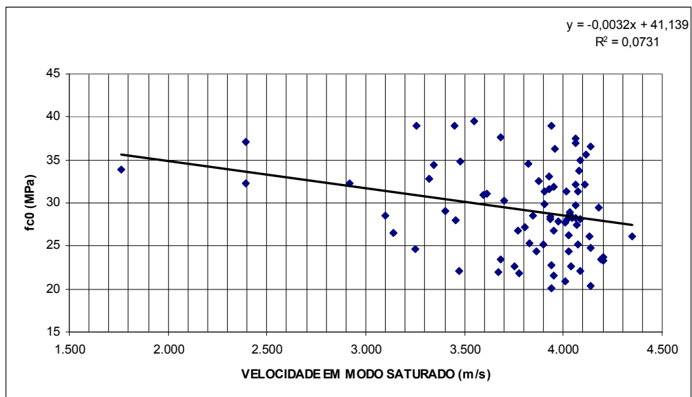
Figura 77 - Correlação entre compressão paralela às fibras e velocidade de propagação longitudinal no modo saturado para todos os lotes.
