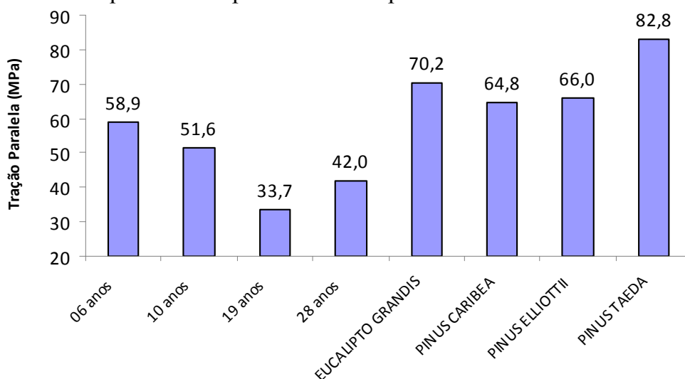
Figura 58 - Valores de resistência à tração paralela às fibras.
