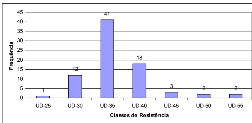
Figura 68 - Frequência da velocidade de propagação no topo das peças de paricá do lote de 19 anos.
