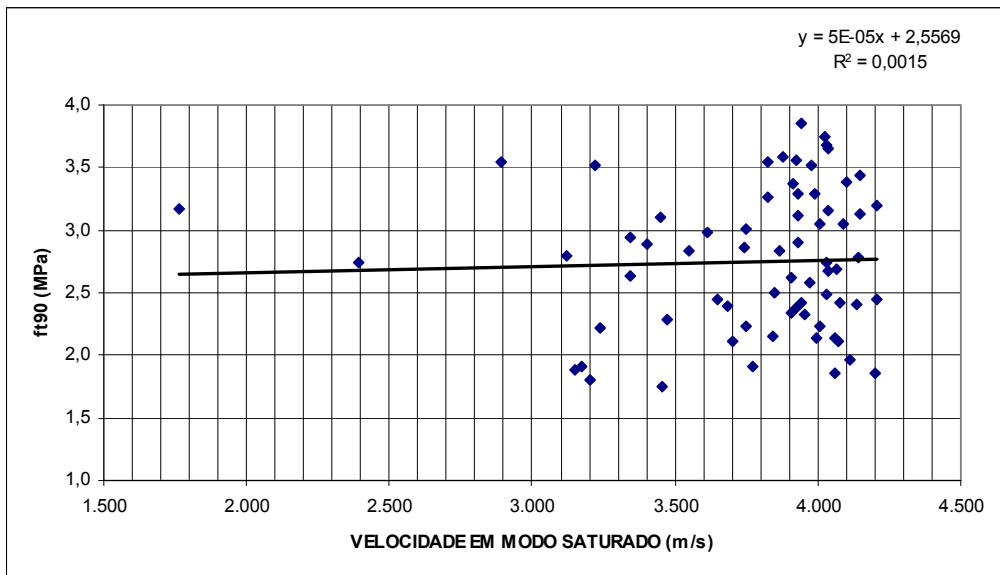
Figura 83 - Correlação entre tração normal às fibras e velocidade de propagação longitudinal no modo saturado para todos os lotes.
