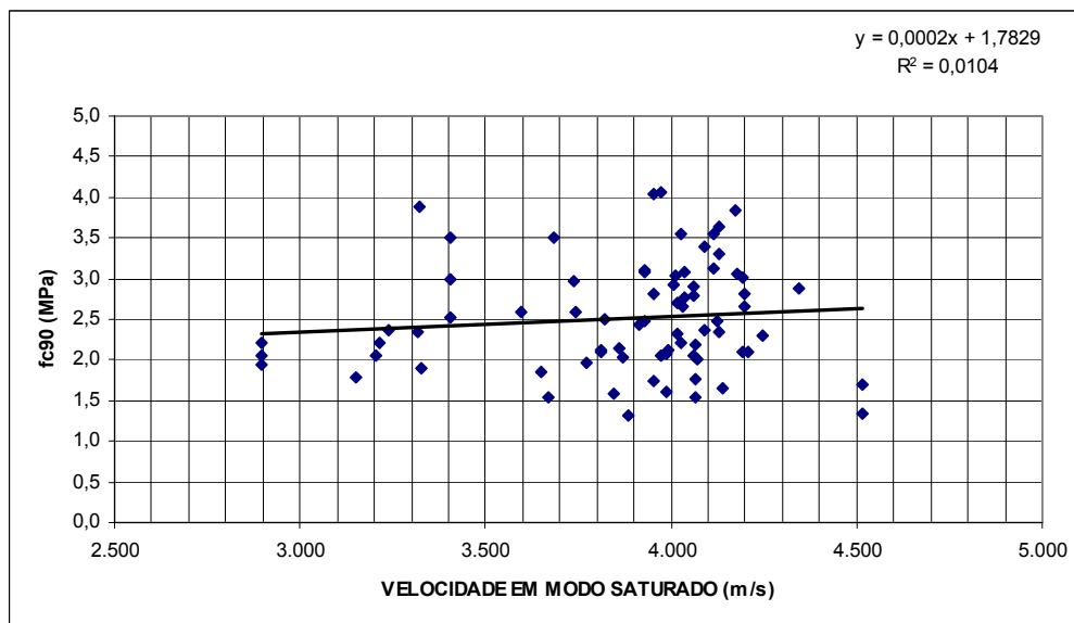
Figura 81 - Correlação entre compressão normal às fibras e velocidade de propagação longitudinal no modo saturado para todos os lotes.
