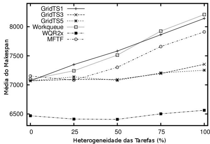
Figura 5.8: Média do makespan variando a heterogeneidade de tarefas
