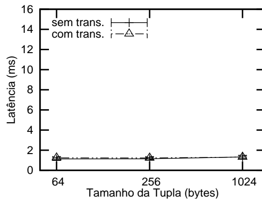
Figura 6.5: Custo da adição do suporte a transações no DEPSpace - Operação rdp
