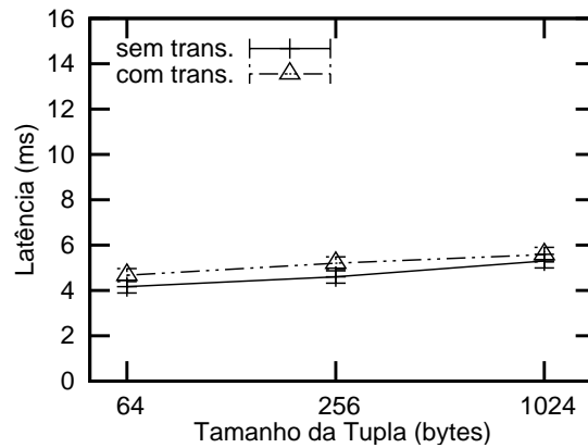
Figura 6.4: Custo da adição do suporte a transações no DEPSpace - Operação out
