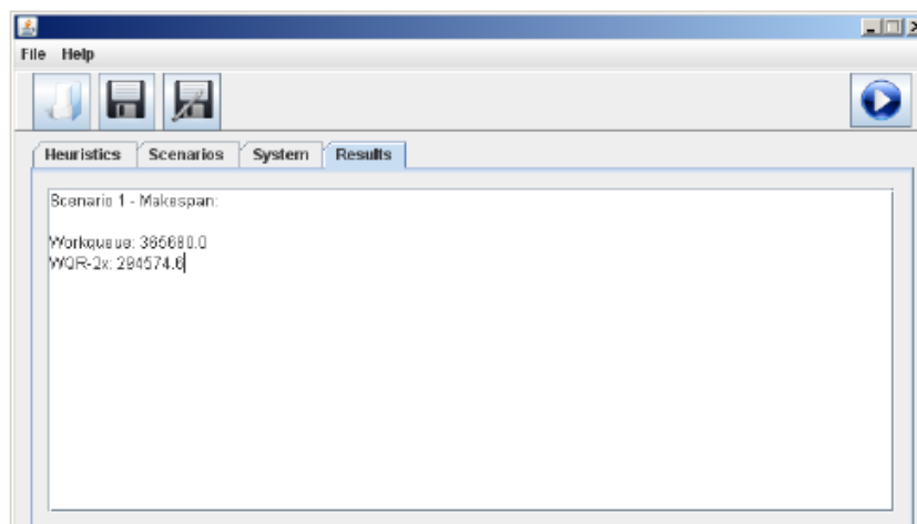
Figura 5.6: Interface Gráfica do AGRIS - Aba Results
