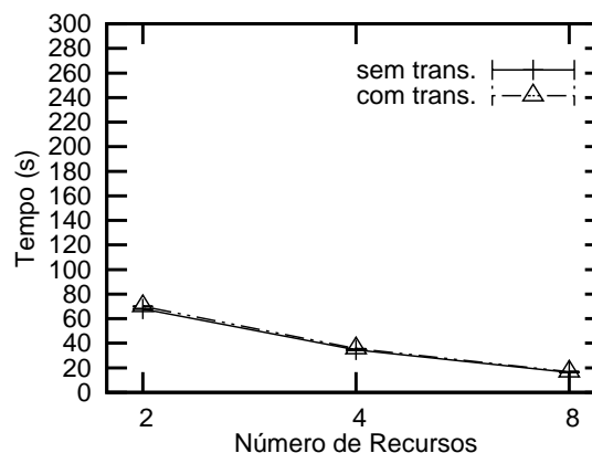
Figura 6.7: Tempo médio de execução para encontrar a chave RC5 - 8.000.000 chaves em cada tarefa
