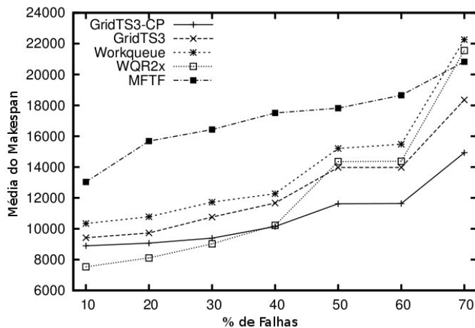
Figura 5.12: Média do makespan considerando falha dos recursos e tarefas com granularidade 2500
