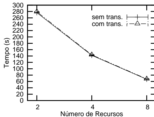
Figura 6.9: Tempo médio de execução para encontrar a chave RC5 - 32.000.000 chaves em cada tarefa
