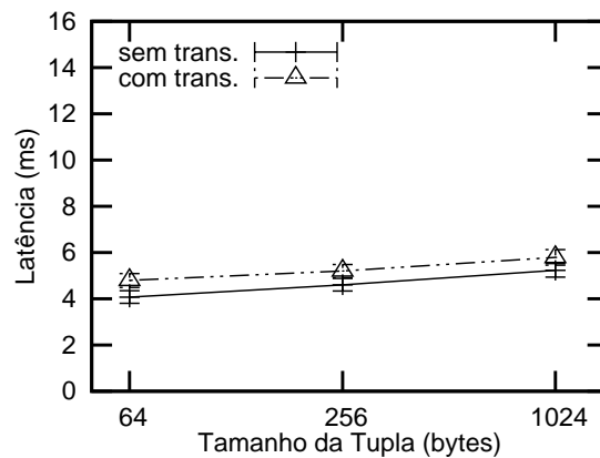
Figura 6.6: Custo da adição do suporte a transações no DEPSpace - Operação inp
