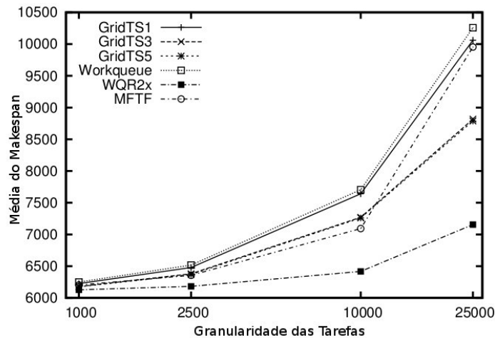
Figura 5.7: Média do makespan variando a granularidade de tarefas
