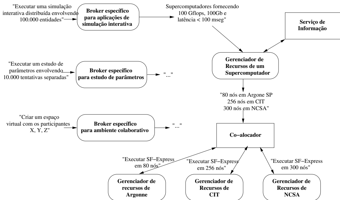
Figura 3.6: Exemplo mostrando diferentes brokers participando de uma única requisição [38]
