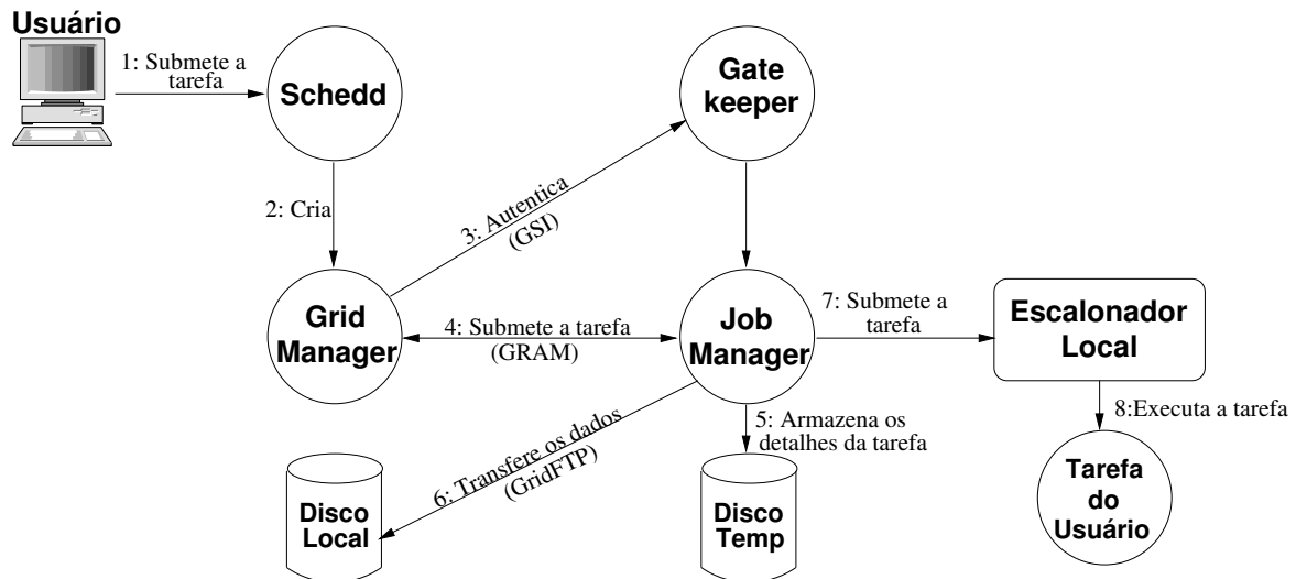
Figura 3.9: Condor-G (Adaptado de [57])
