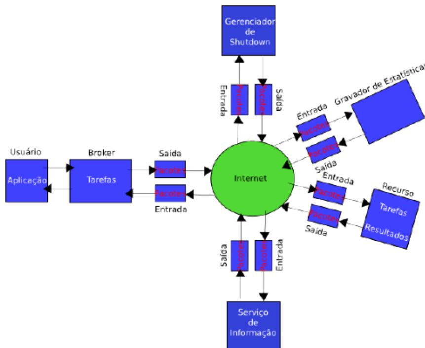
Figura 5.2: Interação das Entidades no GridSim (Adaptada de [24]).
