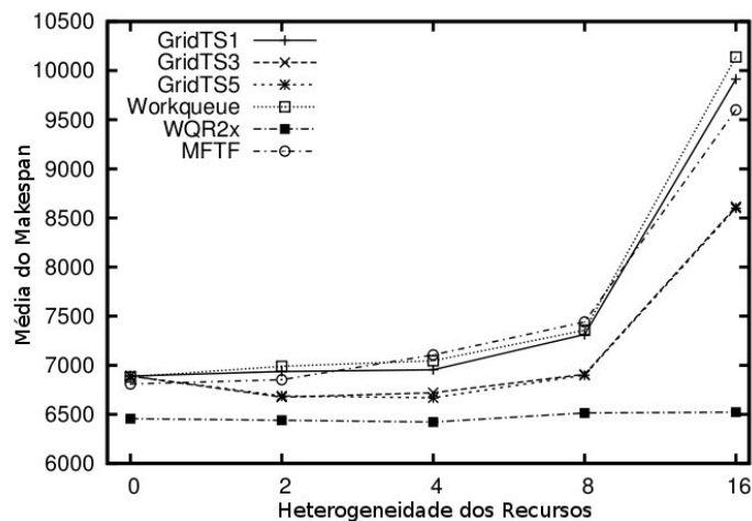
Figura 5.9: Média do makespan variando a heterogeneidade de recursos
