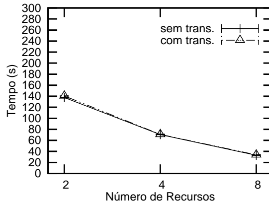
Figura 6.8: Tempo médio de execução para encontrar a chave RC5 - 16.000.000 chaves em cada tarefa
