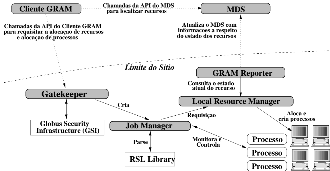
Figura 3.5: Arquitetura do GRAM [38]
