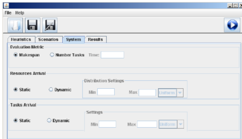
Figura 5.5: Interface Gráfica do AGRIS - Aba System
