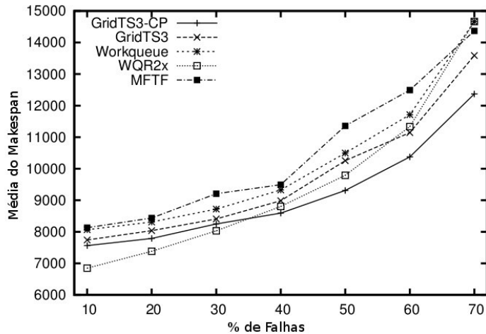
Figura 5.11: Média do makespan considerando falha dos recursos e tarefas com granularidade 10000
