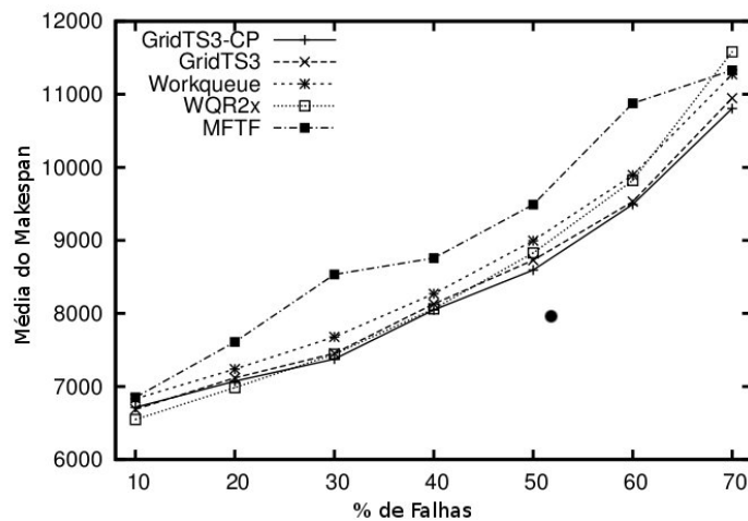
Figura 5.10: Média do makespan considerando falha dos recursos e tarefas com granularidade 2500
