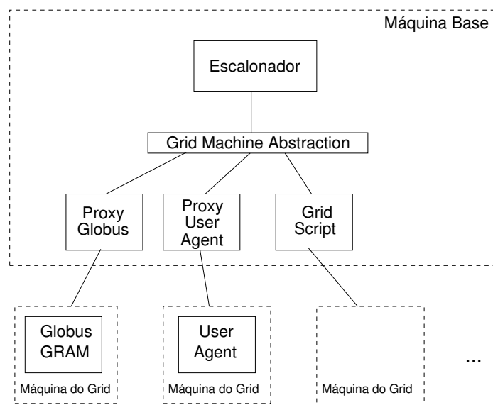
Figura 3.10: Arquitetura do MyGrid [34]
