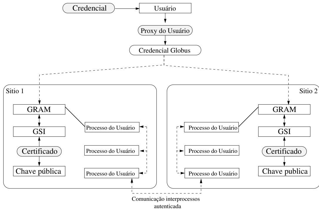
Figura 3.7: Infra-estrutura de Segurança do Globus [56]
