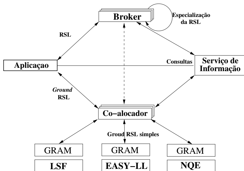
Figura 3.4: Estrutura do Gerenciamento de Recursos no Globus [38]
