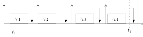
Figura 4.7: Ativações de \tau_i
