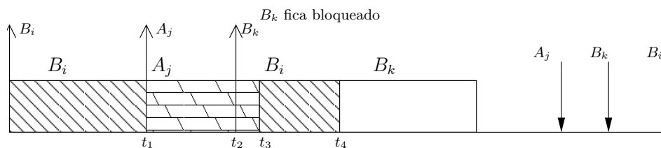
Figura 3.11: Acesso exige bloqueio.
