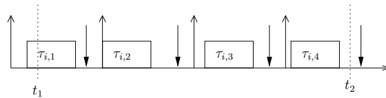
Figura 4.2: Exemplo de ativações de \tau_i , computados por \eta_i
