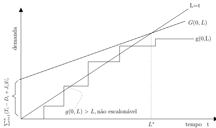
Figura 4.3: Demanda de processador para g(0, L) e G(0, L) .
