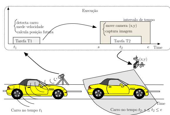
Figura 1.2: Execução com máximo benefício.
