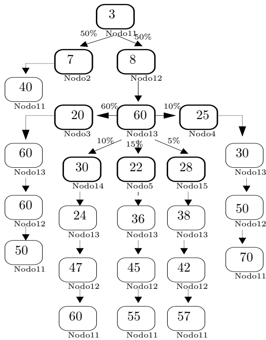
Figura D.25: Thread Distribuída NB25.
