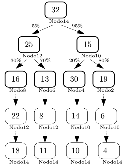
Figura C.4: Thread Distribuída B4.
