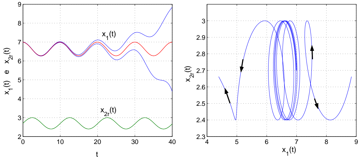
FIGURA 3.20: Dinâmica interna do boost controlado a partir da imposição de x_{2r} . (a) Evoluções de 3 sinais de x_1(t) com condições iniciais ligeiramente diferentes, (b) evolução da trajetória dos estados no espaço de estados (x_1, x_2) .
