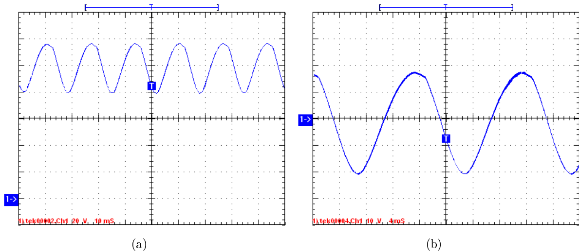
FIGURA 4.21: Formas de onda da tensão de saída (a) Medição DC com 20V/div vertical e 10ms/div horizontal; (b) Medição AC com 10V/div vertical e 4ms/div horizontal.
