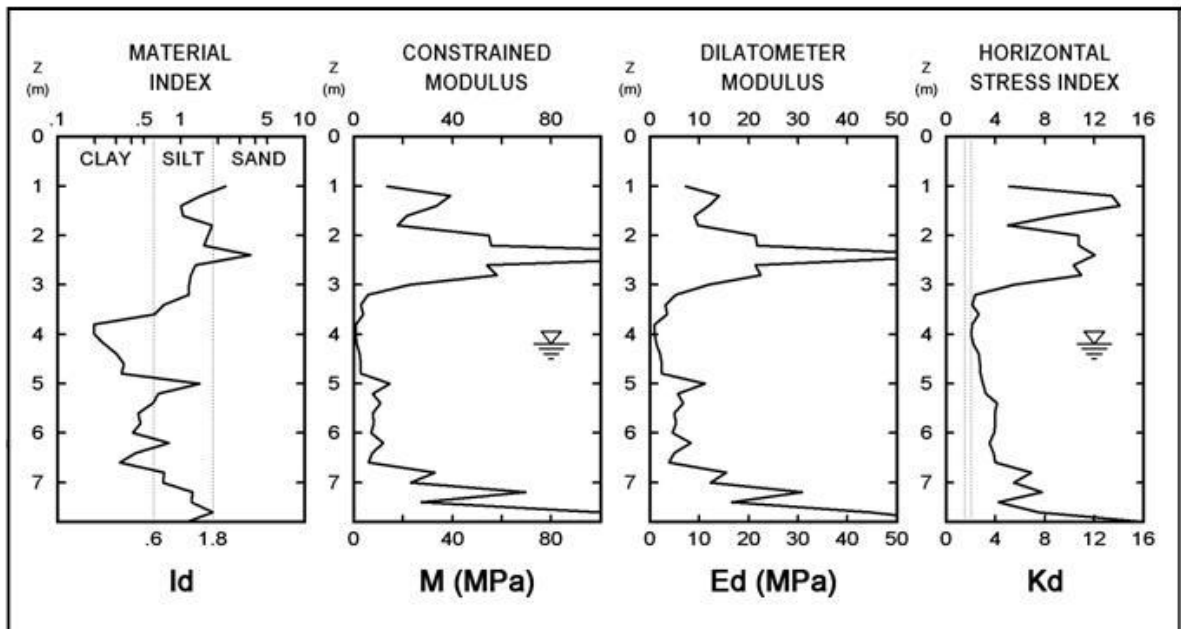
FIGURA 34 – Resultados do ensaio 1: CPT-01 , DMT-01 , SPT-12 FONTE: Autor
