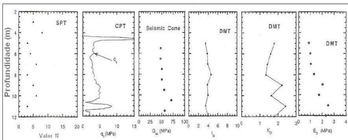
FIGURA 7 - Resultados de testes em Ohgishima
