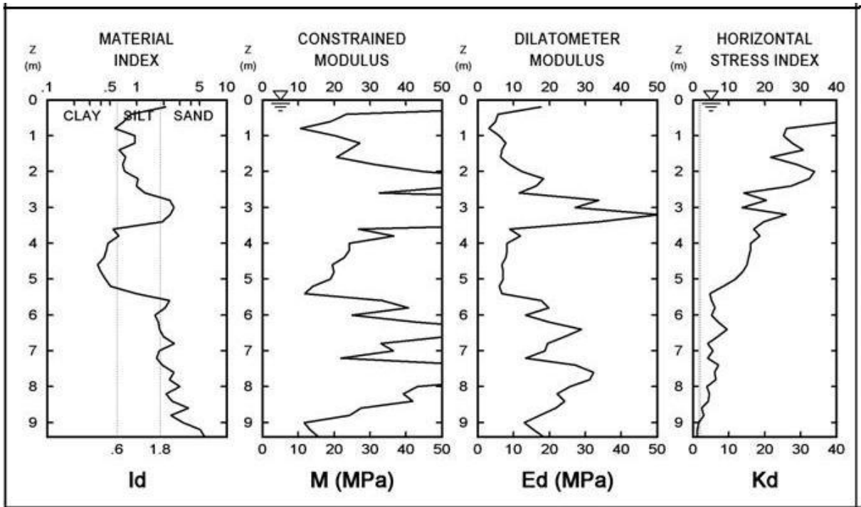
FIGURA 67 – Resultados do ensaio 3: CPT-03 , DMT-03 , SPT-15 FONTE: Autor
