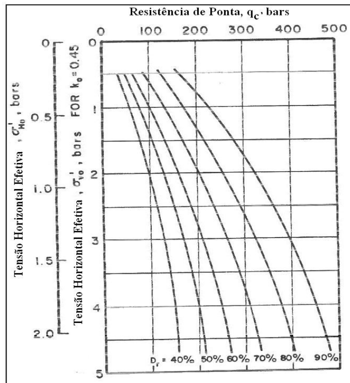
FIGURA 24 - Densidade relativa para areias de quartzo não cimentadas e não envelhecidas Fonte: Baldi et al. (1982)
