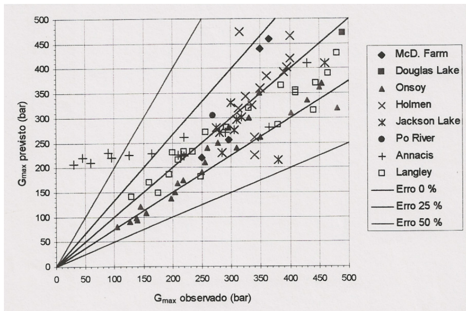
FIGURA 15 - Comparação entre G_{max} previsto e G_{max} observado – Hryciw, 1990 (adaptado por Jardim em 1998)
