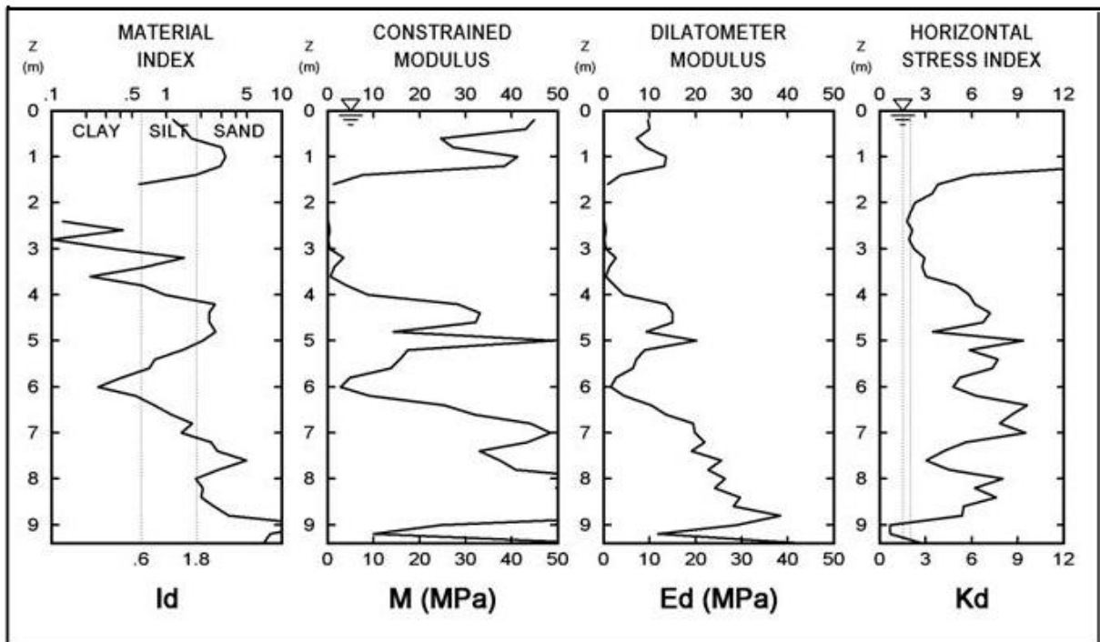
FIGURA 64 – Resultados do ensaio 3: CPT-02, DMT-02, SPT-14 FONTE: Autor
