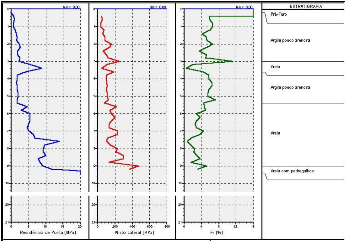
FIGURA 66 – Resultados do ensaio 3: CPT-03 , DMT-03 , SPT-15 FONTE: Solo Sondagem
