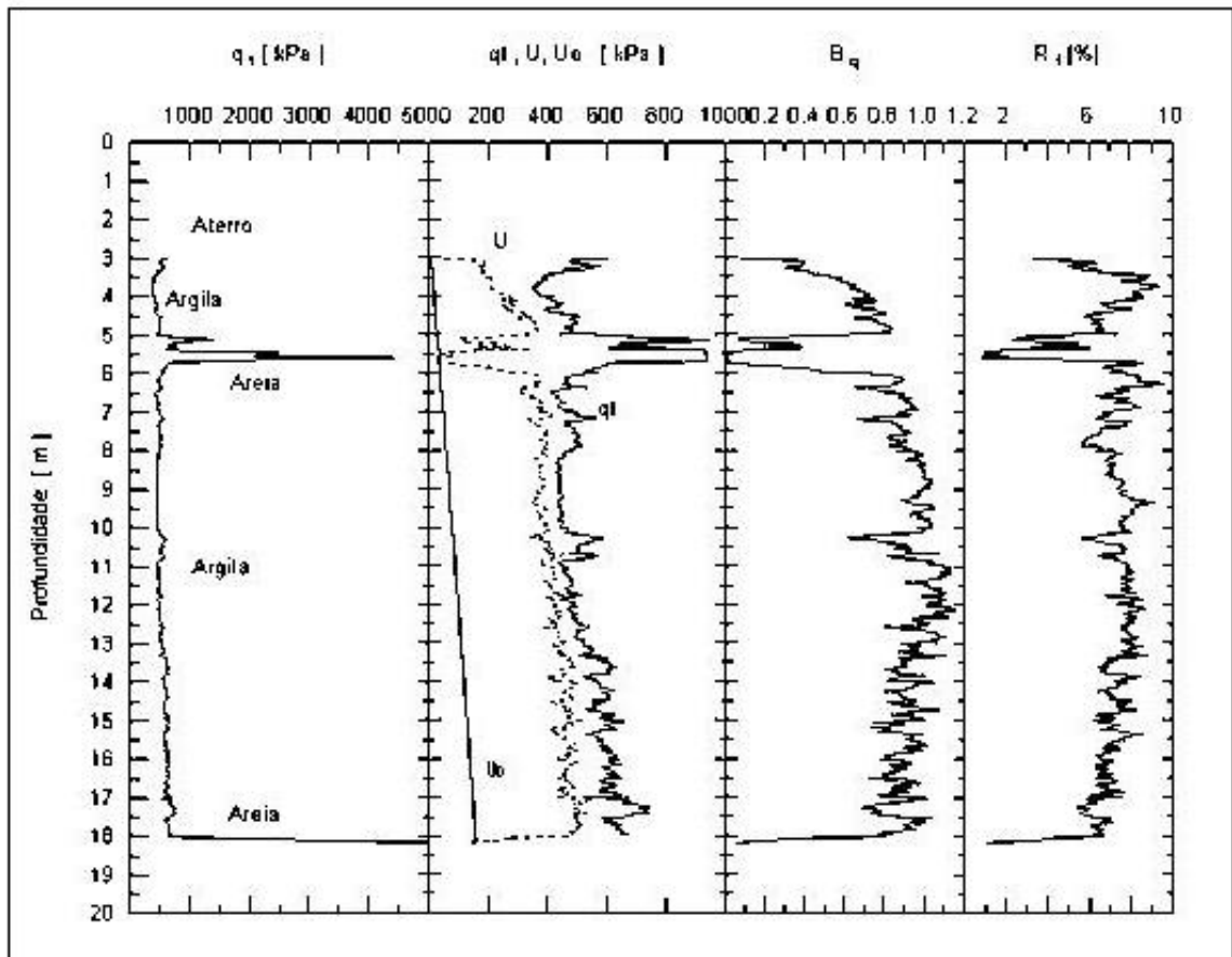
FIGURA 20 - Resultado de um ensaio Piezocone na BR 101 em SC
