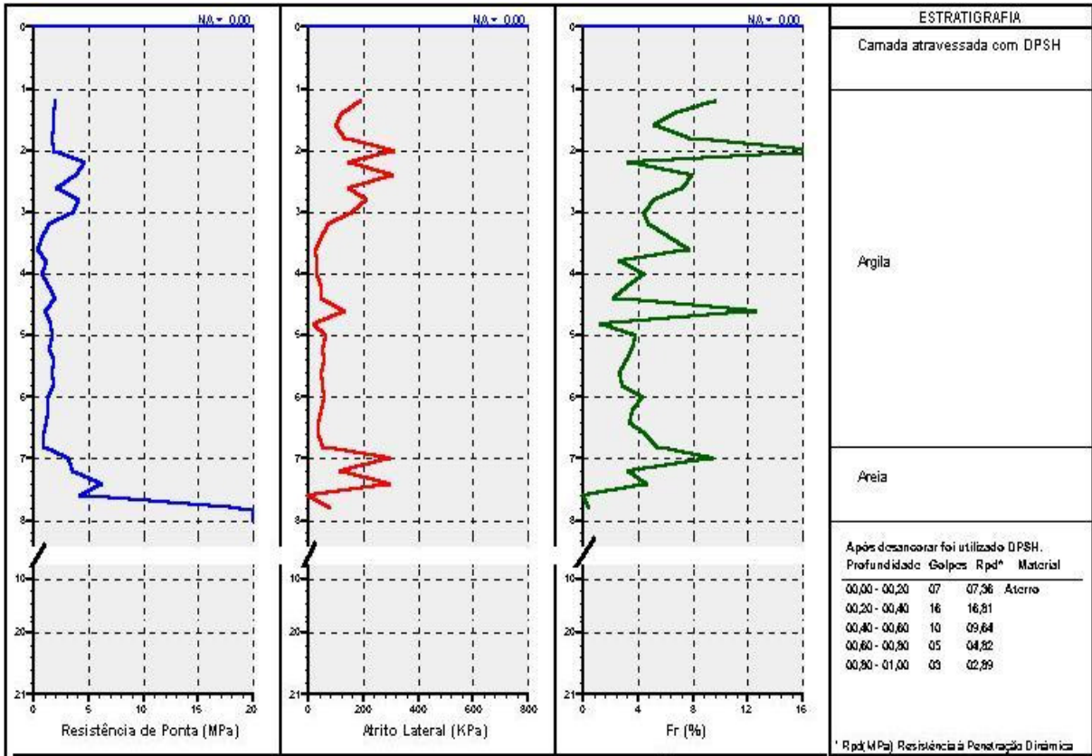
FIGURA 33 – Resultados do ensaio 1: CPT-01 , DMT-01 , SPT-12 FONTE: Solo Sondagem
