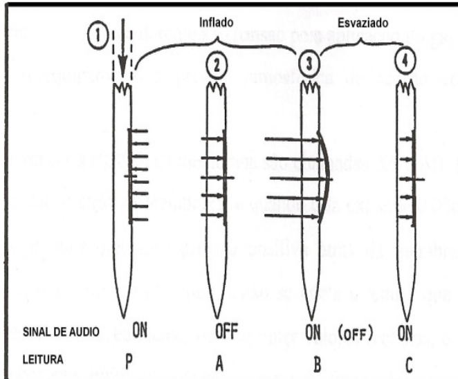
SEQÜÊNCIA DE TESTE DO DILATÔMETRO
