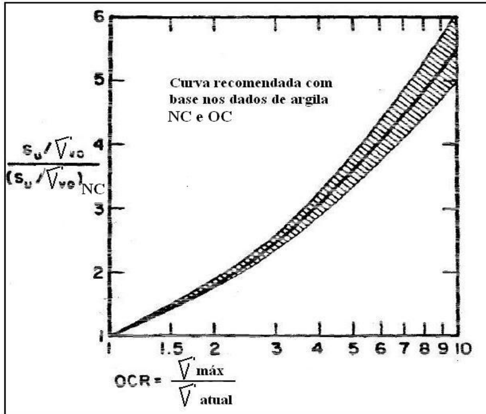
FIGURA 21 - Estimativa de OCR a partir da relação normalizada ( S_u/\sigma_{vo} ) Fonte: Schmertamm(1978)
