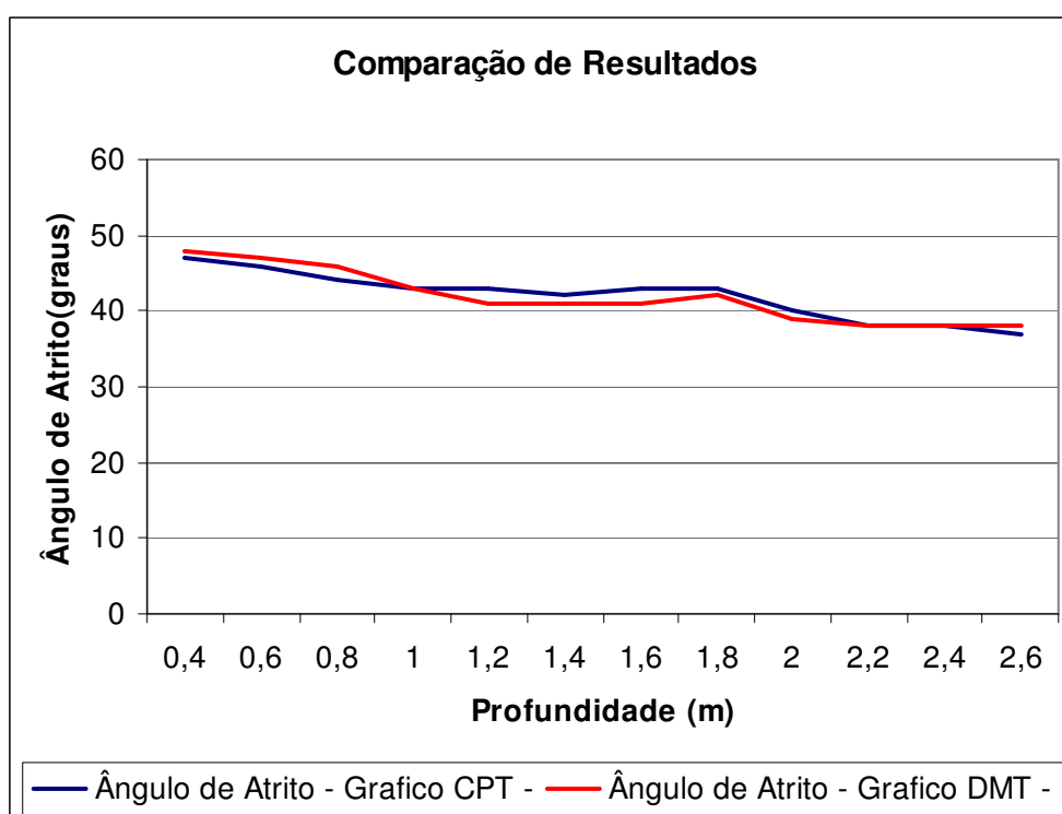
FIGURA 105 – Gráfico do ângulo de atrito – Ensaio 5
