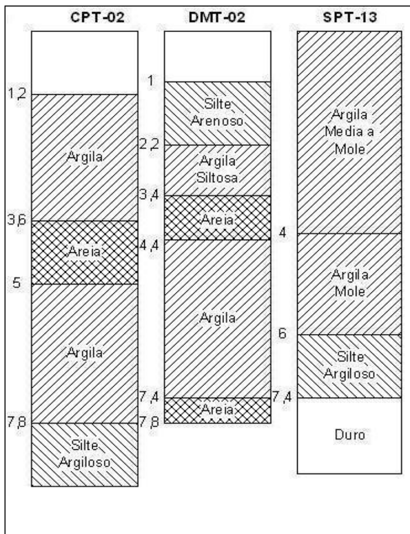
FIGURA 85 - Perfis estratigráficos ensaio 1 CPT-02, DMT-02, SPT-13
