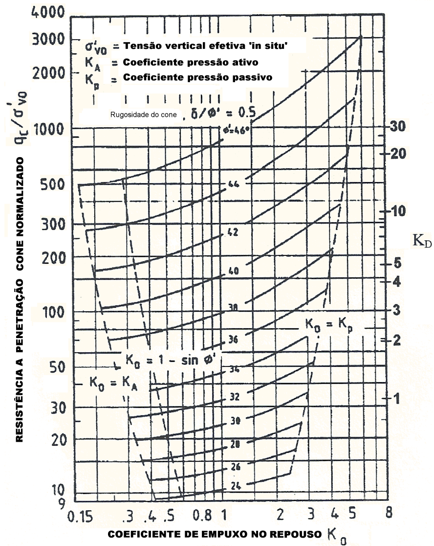
FIGURA 14 - Ábaco proposto por Campanella e Robertson (1991) para avaliação de K_D através de \phi e K_0 em areias não cimentadas.
