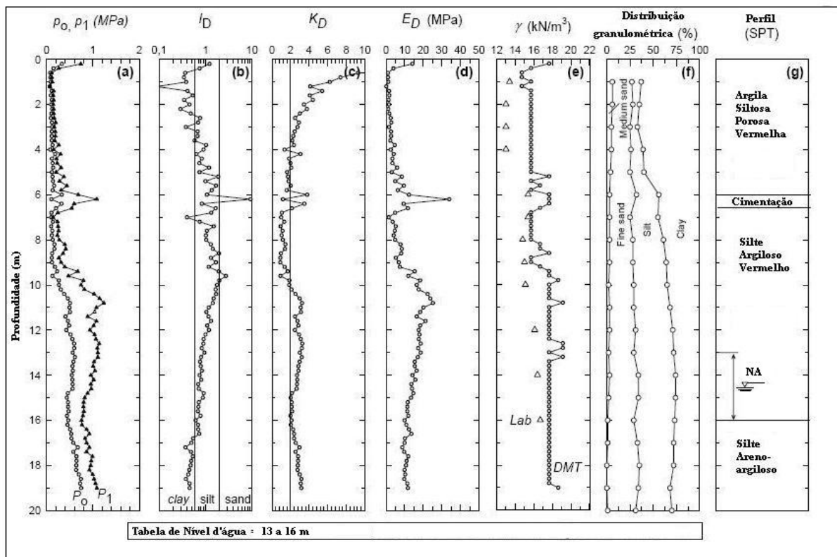
FIGURA 3 - Resultados de ensaios DMT, peso específico total, distribuição granulométrica e perfil SPT para a região de Campinas.
