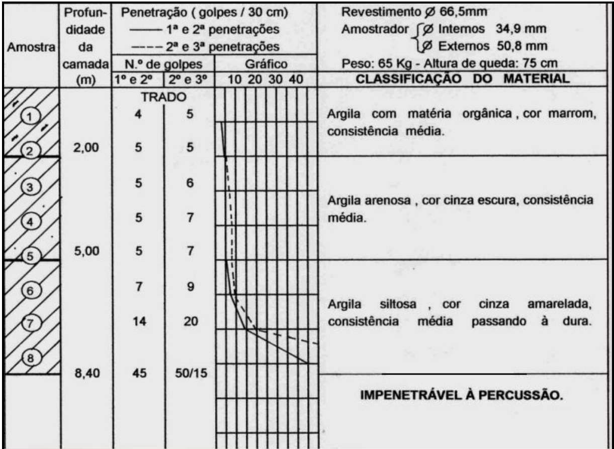
FIGURA 47 – Resultados do ensaio 1: CPT-05, DMT-05, SPT-17 (N.A. = 0,3m)
