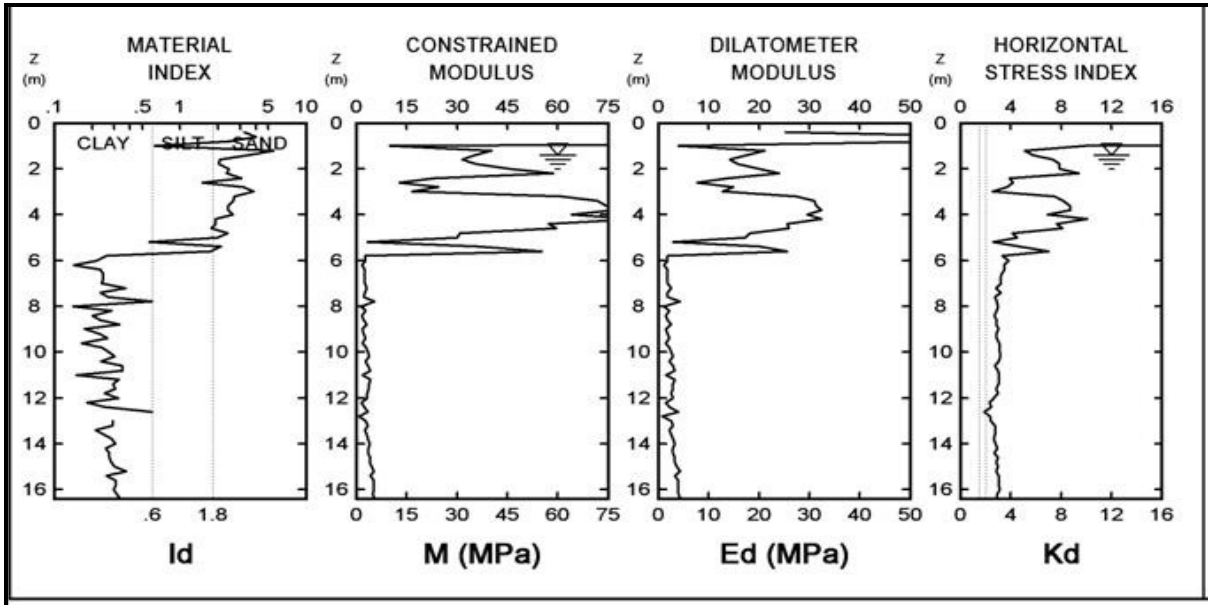
FIGURA 57 – Resultados do ensaio 2: CPT-01, DMT-01, SPT-01
