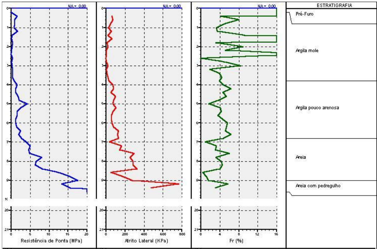
FIGURA 63 – Resultados do ensaio 3: CPT-02, DMT-02, SPT-14 FONTE: Solo Sondagem
