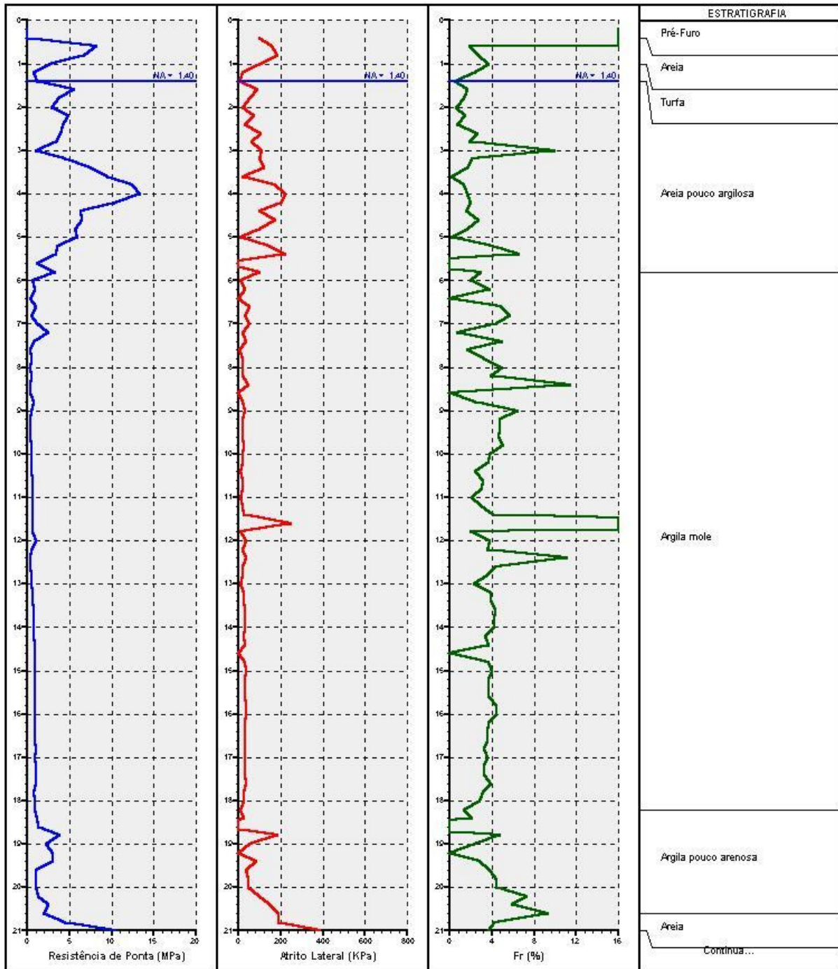
FIGURA 56 – Resultados do ensaio 2: CPT-01, DMT-01, SPT-01 FONTE: Solo Sondagem
