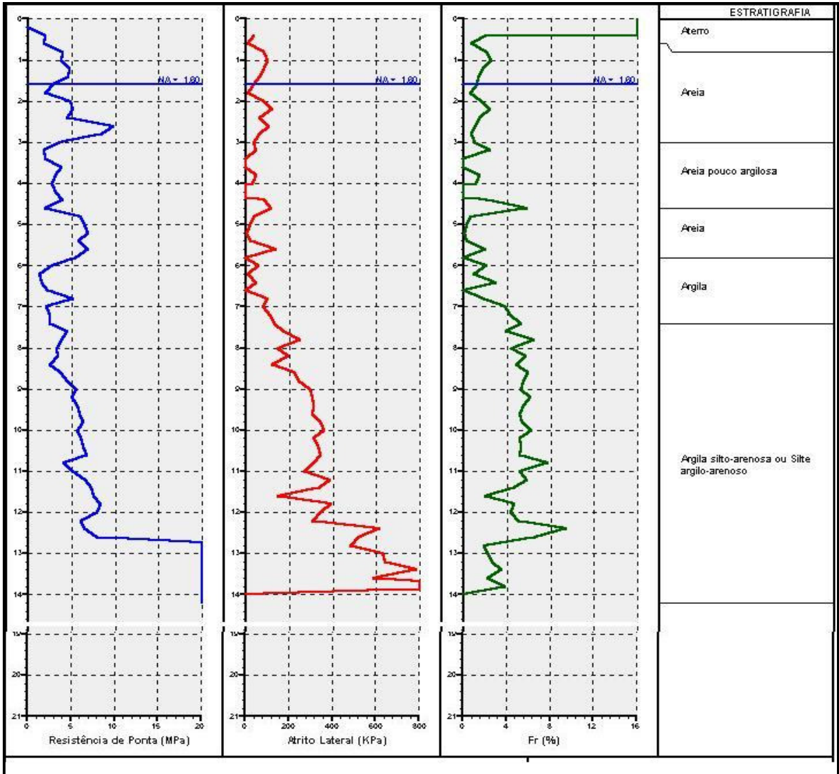
FIGURA 76 – Resultados do ensaio 4: CPT-04, DMT-04, SM-02 FONTE: Solo Sondagem
