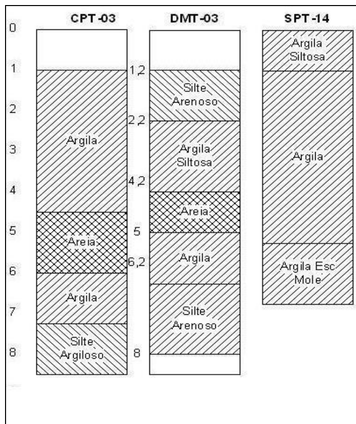
FIGURA 86 - Perfis estratigráficos ensaio 1 CPT-03, DMT-03, SPT-14
