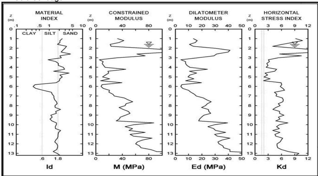
FIGURA 77 – Resultados do ensaio 4: CPT-04, DMT-04, SM-02 FONTE: Autor
