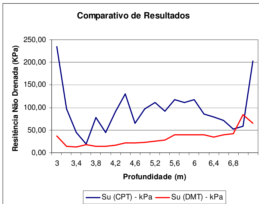
FIGURA 91 – Gráfico resistência não drenada Ensaio 1
