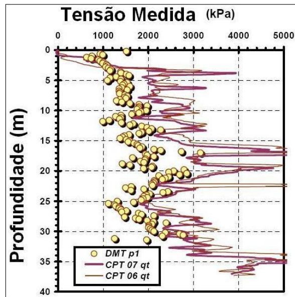
FIGURA 6 - Comparação de p_1 com o perfil q_t em argilas OC em Baton Rouge, LA. FONTE: Mayne (2006)
