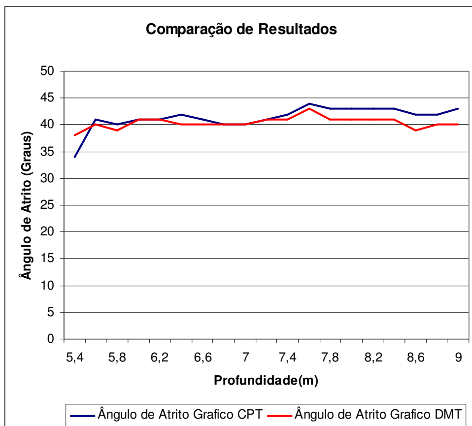
FIGURA 99 – Gráfico do ângulo de atrito – Ensaio 3
