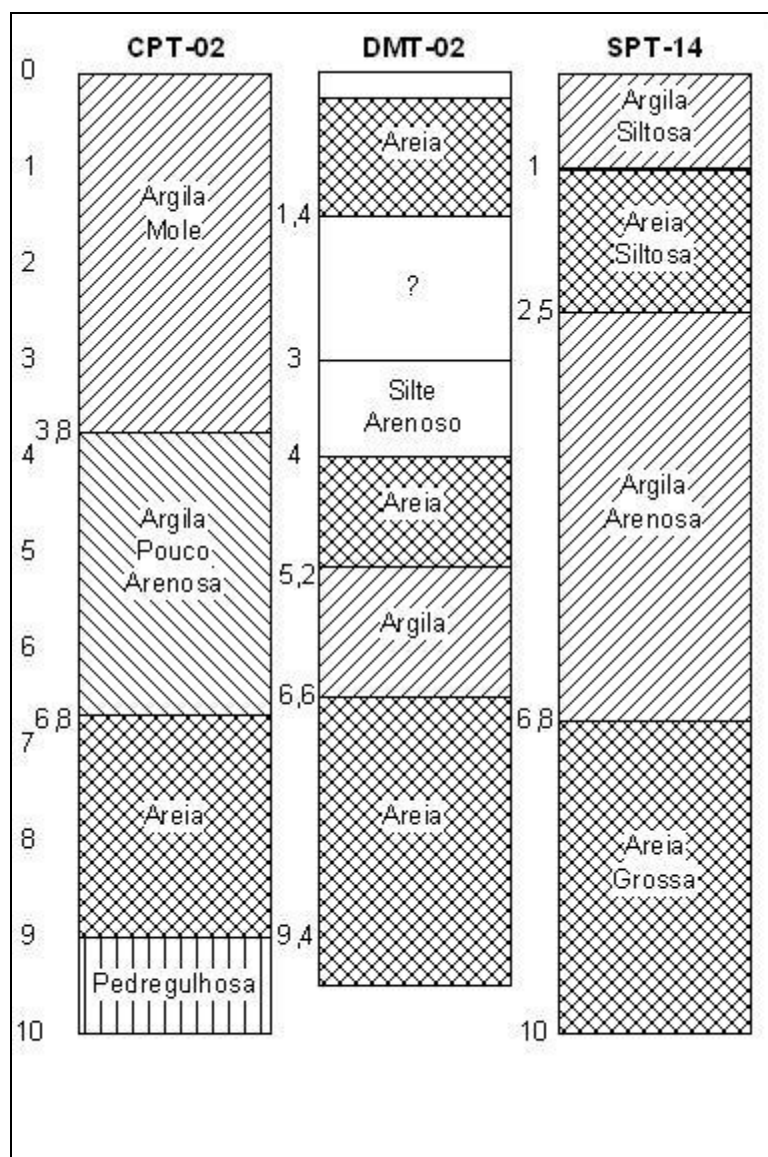
FIGURA 97 - Perfis estratigráficos ensaio 3 CPT-02, DMT-02 e SPT-14
