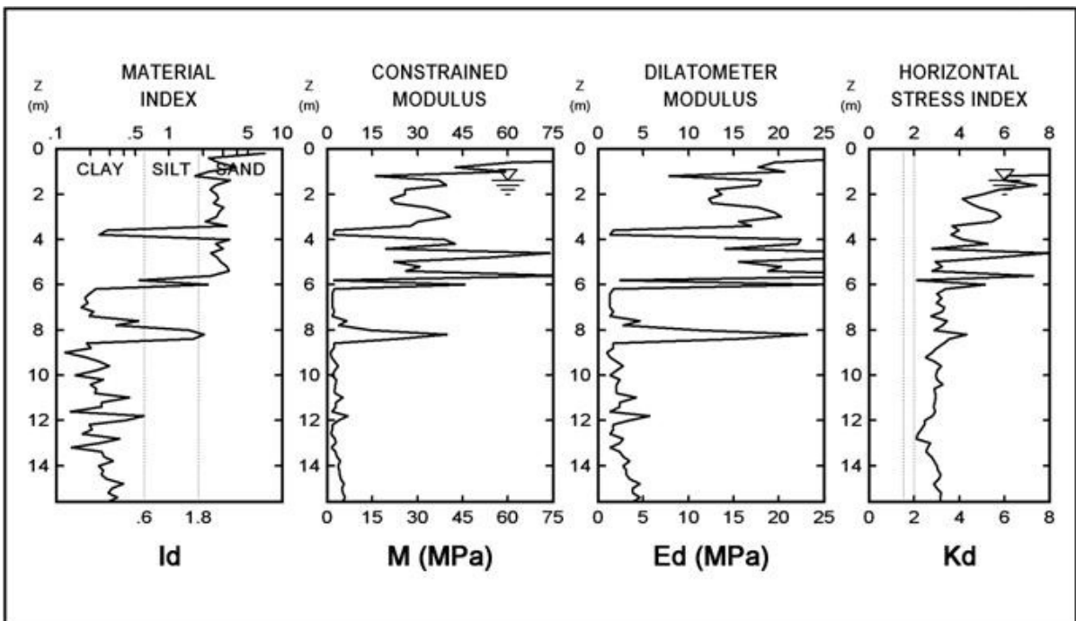
FIGURA 58 – Resultados do ensaio 2: CPT-02, DMT-02, SPT-01
