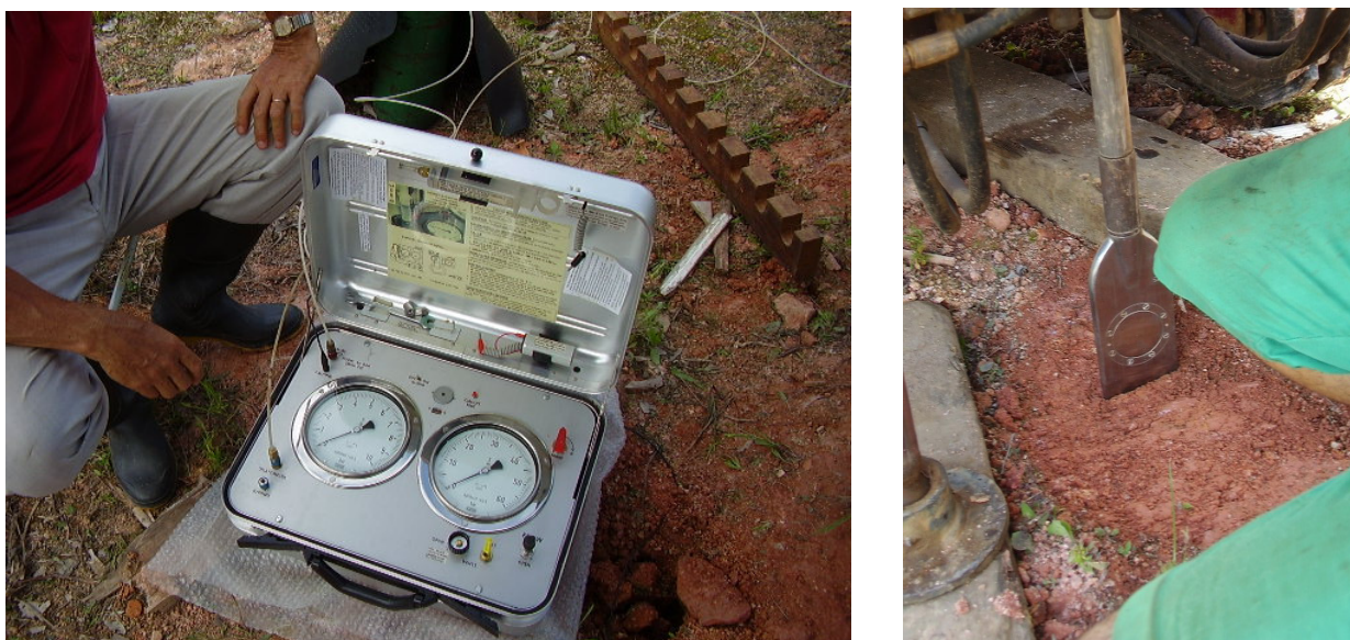
FIGURA 9 – Fotos da unidade de controle (esquerda) e da lâmina penetrando no solo (direita) FONTE: Ensaio realizado em dez/2006, no local do ensaio 4
