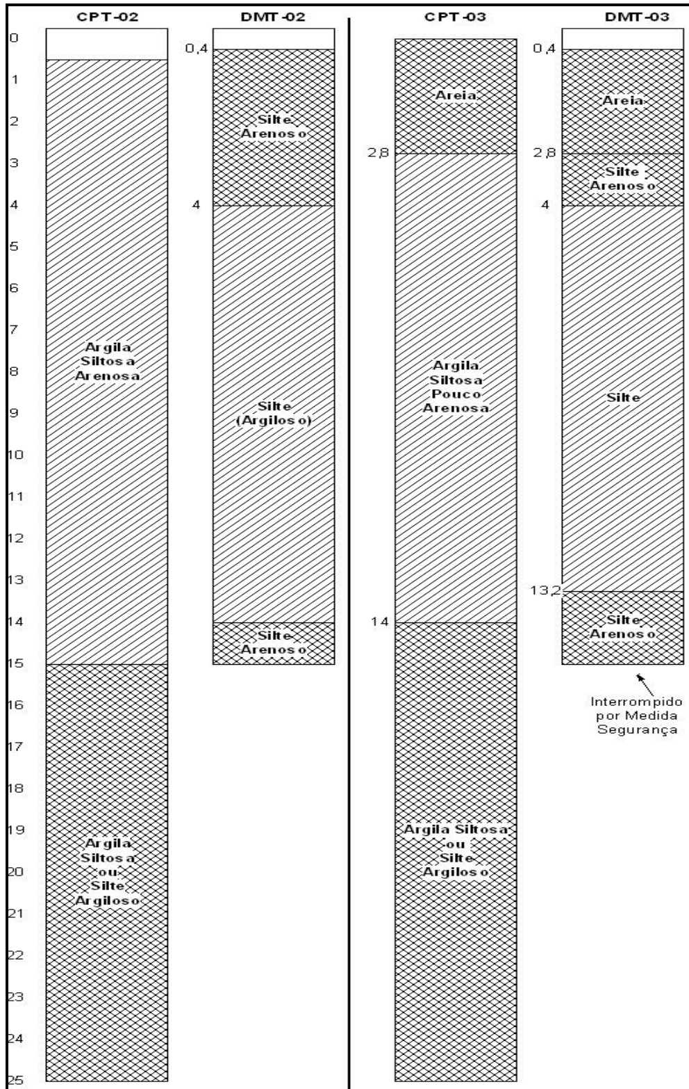
FIGURA 104 – Perfis estratigráficos ensaio 5 CPT-02/DMT-02 e CPT-03/DMT-03
