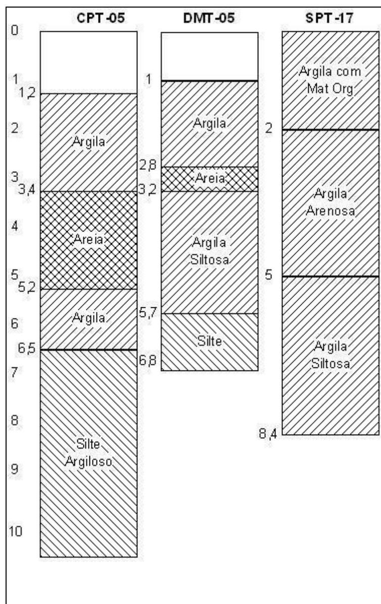
FIGURA 88 - Perfis estratigráficos ensaio 1 CPT-05, DMT-05, SPT-17
