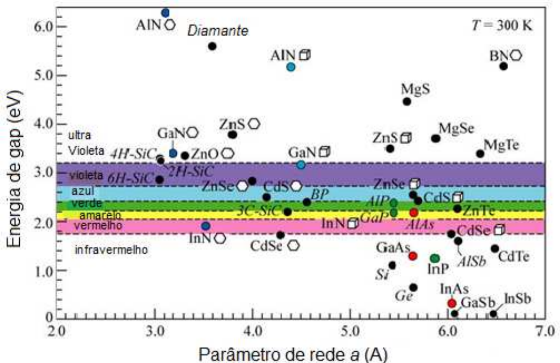
Figura 3. Energia de gap em função do parâmetro de rede a temperatura ambiente de elementos comuns e sistemas binários. Adaptada de 37 .
