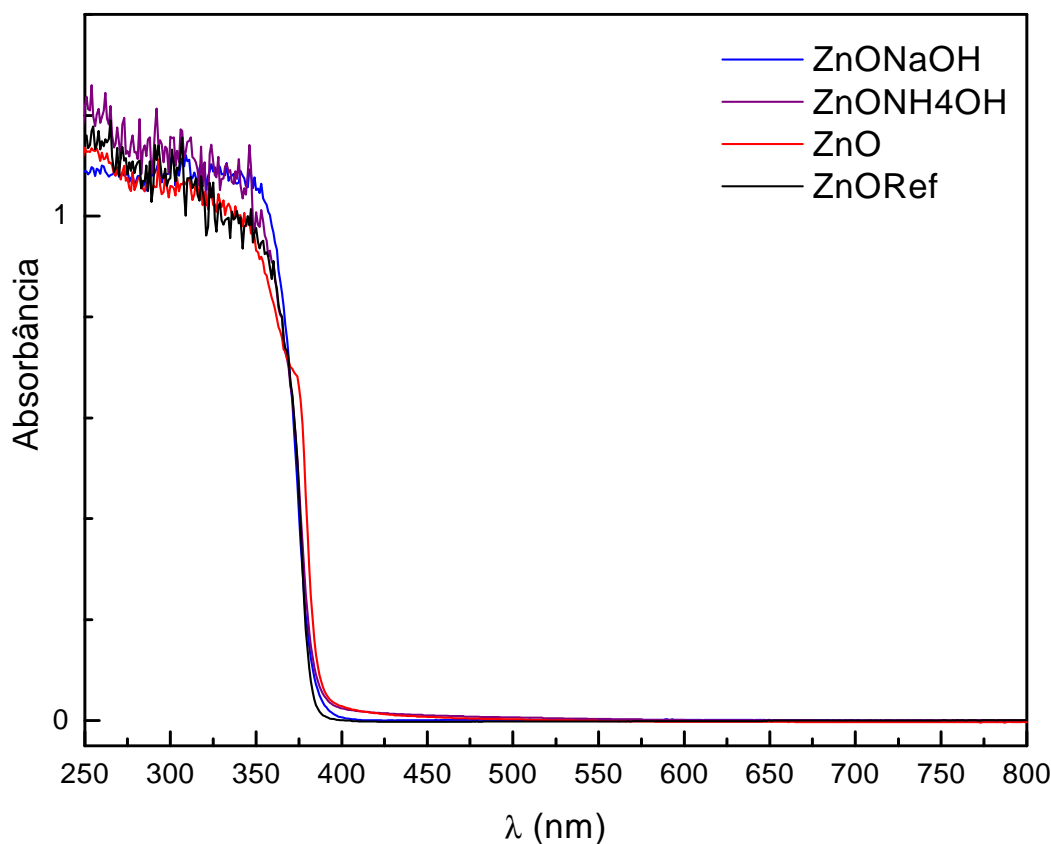
Figura 20. Espectro de UV-Vis das amostras sintetizadas em comparação com ZnOref.
