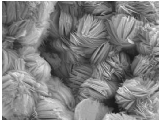
Figura 6 – Micrografia do gel produto da reação álcali-silica ampliado 4000 vezes (BEKTAS et al. , 2008).
