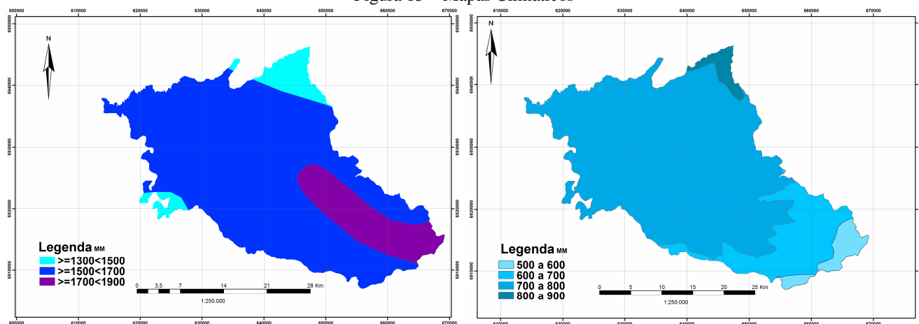
Figura 13 – Mapas Climáticos
