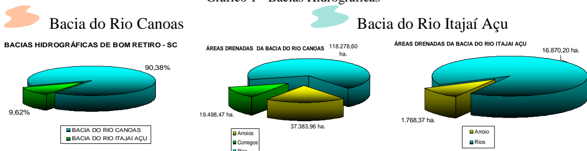
Gráfico 1 - Bacias Hidrográficas
