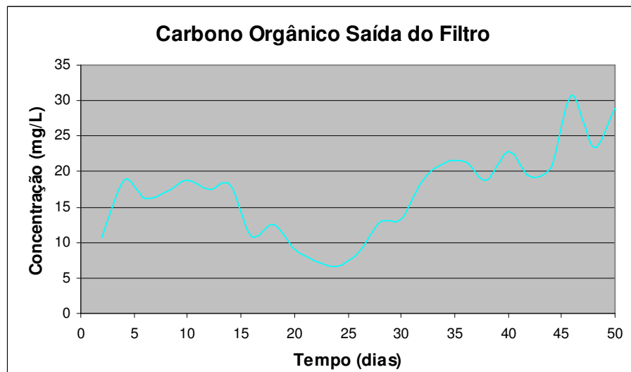
Figura 5.21: Variação ao longo do tempo do Carbono Orgânico Total na saída do filtro biológico do sistema com recirculação.
