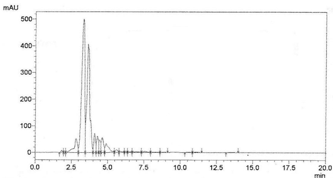
Figura 7 - Cromatograma do extrato branco de esgoto sintético.
