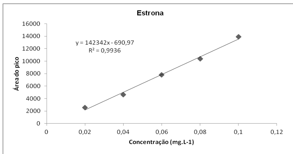
Figura 9 - Curva de calibração para o hormônio natural estrona (E1)
