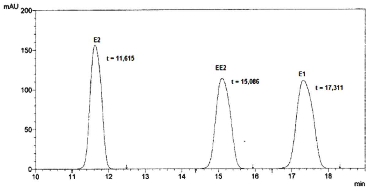
Figura 6 - Cromatograma de uma mistura de padrões, com concentração igual a 20 mg.L -1 de estrona (E1), 17 \beta -estradiol (E2) e 17 \alpha -etinilestradiol (EE2).
