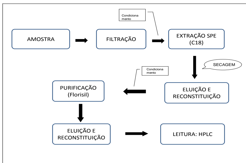
Figura 4 - Fluxograma do procedimento de extração em fase sólida (SPE)
