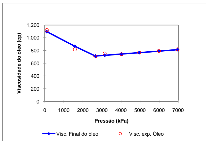
Figura 5-4– Viscosidade do óleo em função da pressão.
