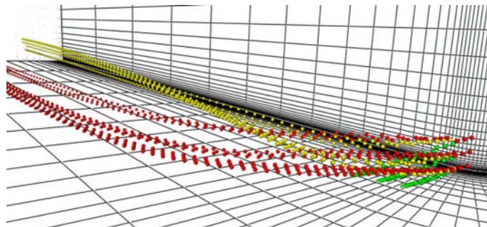
Figura 2.10 – As streak balls mostram o fluxo em um conjunto de dados de uma aleta. As bolas vermelhas são computadas num grid curvilíneo esperso de nível 4, as amarelas em nível 3 e as verdes em nível 2. (fonte: Teitzel e Ertl, 1999)
