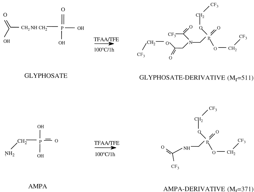
Figura XII: Reação de derivatização do glifosato e do AMPA com TFAA e TFE
