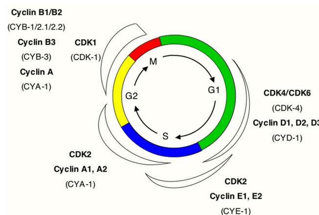
Figura X: Representação do ciclo celular, com suas fases bem definidas e com suas durações e transições mediadas pelas ciclinas.
