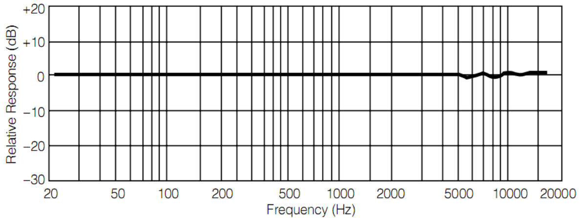
Figura 4.2: Curva de resposta de magnitude x frequência para o eletreto Panasonic WM-61A
