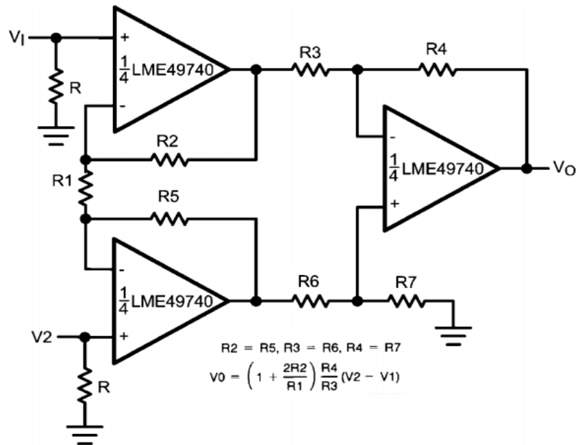
Figura 4.6: Diagrama esquemático do estágio de amplificação
