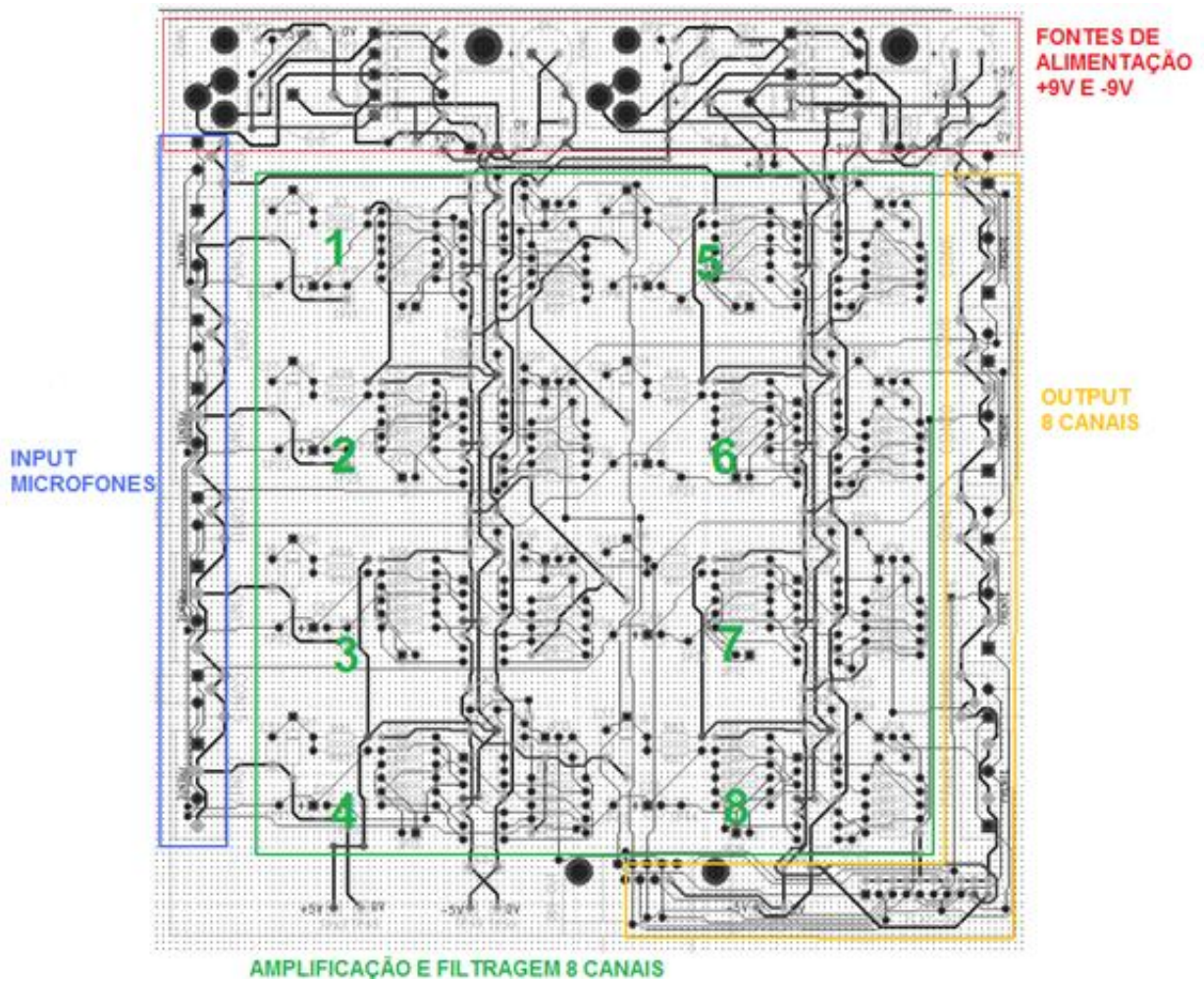
Figura 4.13: Placa de circuito impresso para amplificação e filtragem
