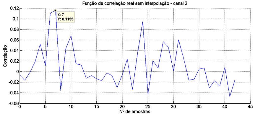
Figura 4.21: Correlação real obtida para um atraso de 6 amostras entre canais
