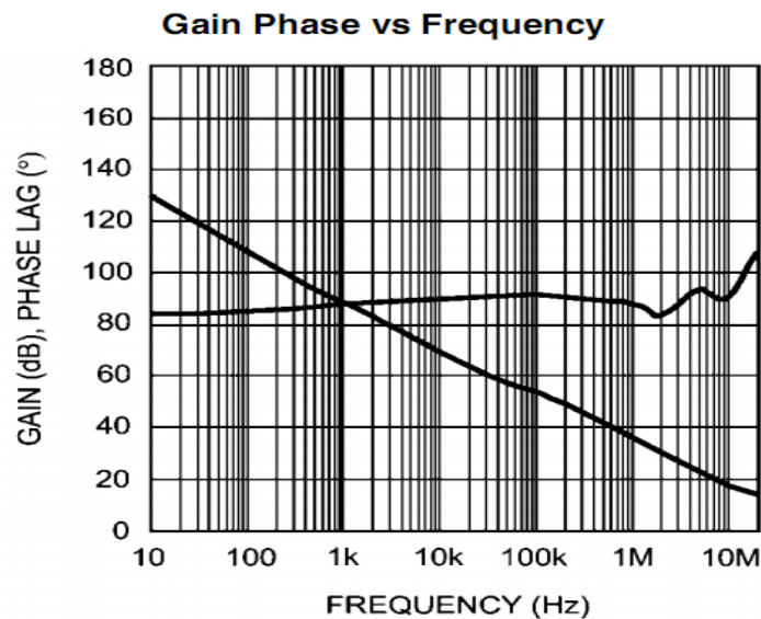
Figura 4.5: Curva de fase e atraso de grupo LME49740
