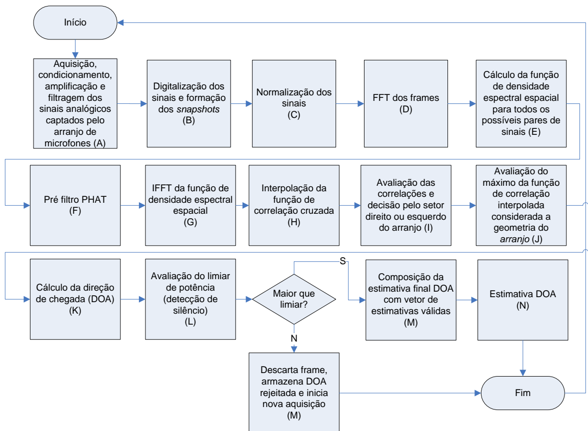
Figura 4.1: Visão geral do sistema de estimação DOA
