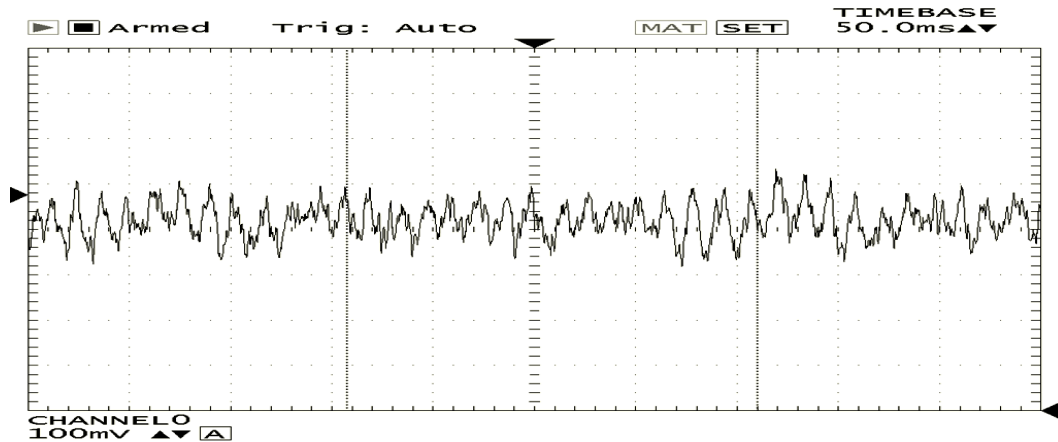
Figura 4.14: Ruído ambiente com escala de 100 mV
