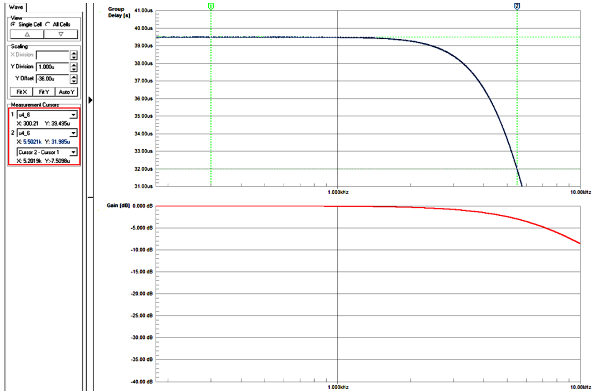
Figura 4.9: Simulação para o bloco de filtragem analógica
