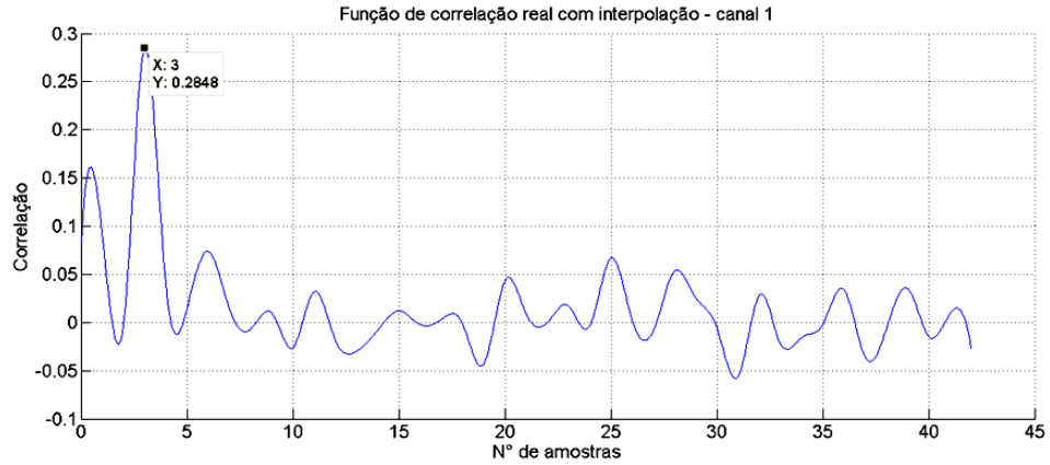
Figura 4.24: Correlação real com interpolação obtida para um atraso de três amostras entre canais
