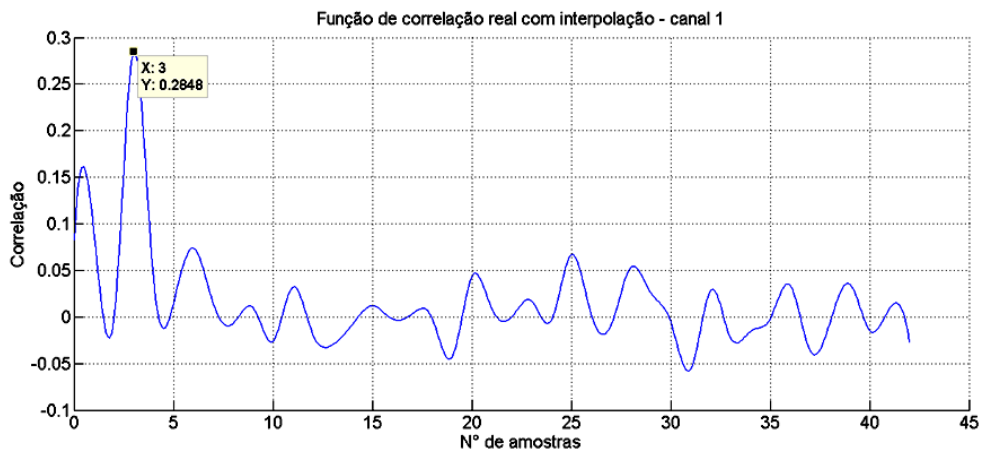
Figura 4.28: Correlação real com interpolação obtida para um atraso de três amostras entre canais
