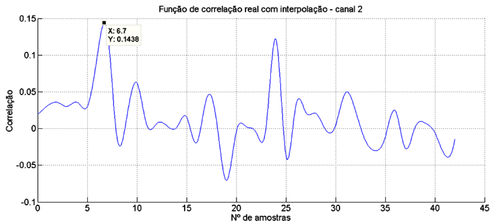
Figura 4.29: Correlação real com interpolação obtida para um atraso de 6 amostras entre canais
