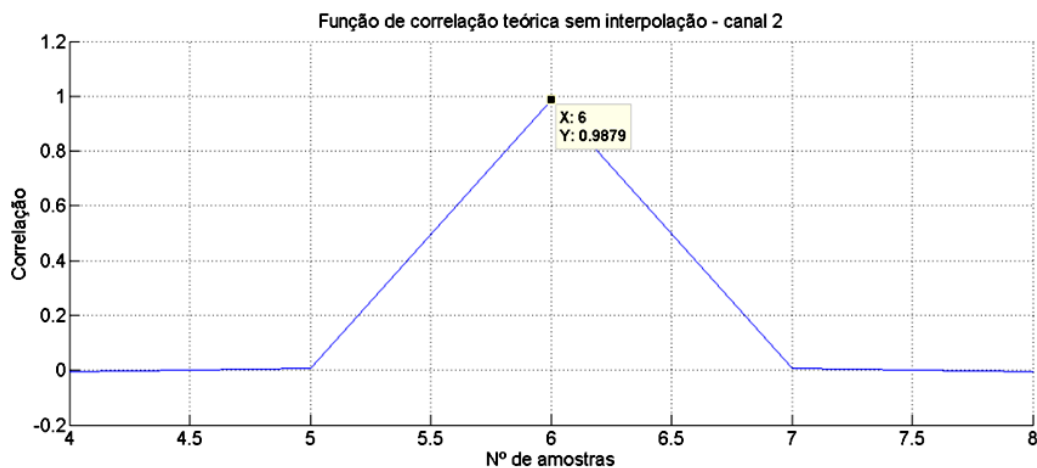
Figura 4.20: Correlação teórica simulada para um atraso de 6 amostras entre canais
