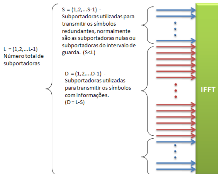
Figura 4.4: Diagrama da técnica de subportadoras virtuais
