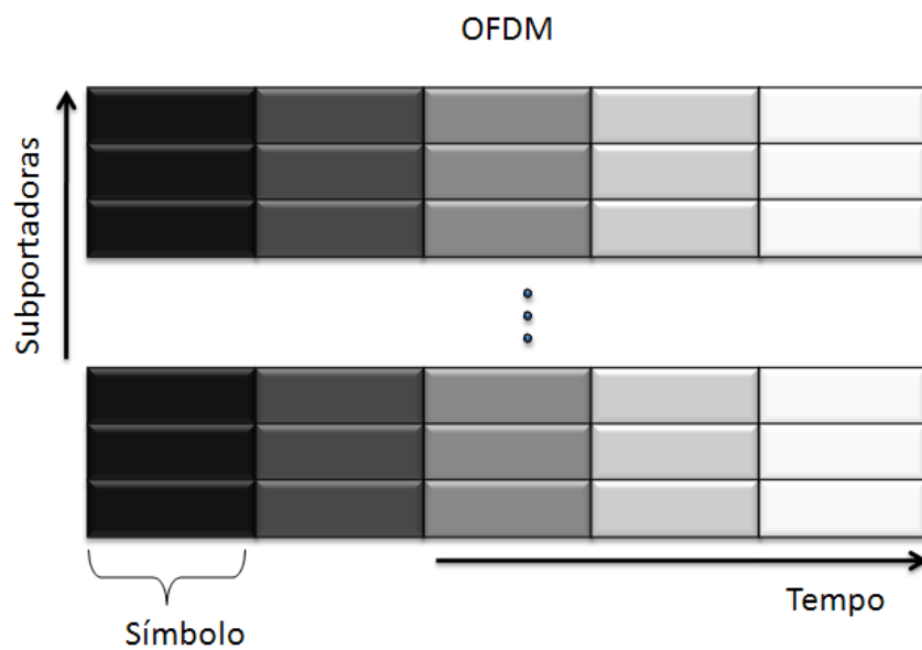
Figura 5.1: Sistema OFDM
