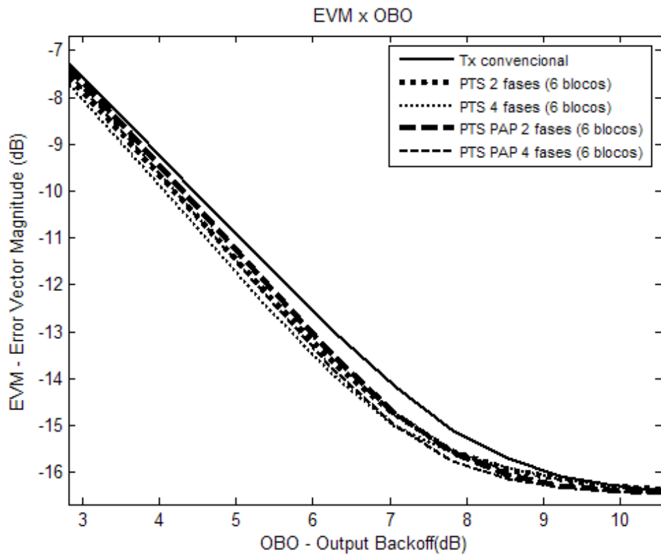
Figura 6.52: EVM do método de PTS com a utilização de 6 blocos
