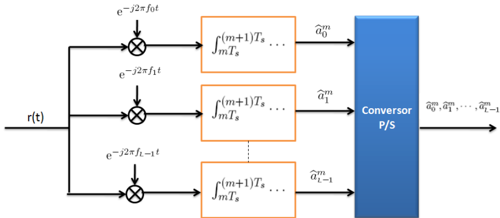
Figura 3.3: Demodulador OFDM
