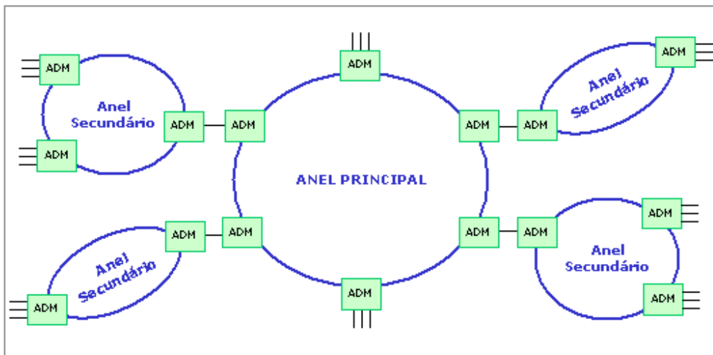
Figura 3-12 - Topologias Típicas
