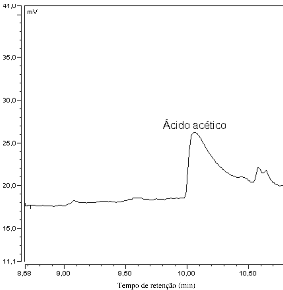
Figura 12 - Cromatograma representando os compostos produzidos pela cultura 55 ( Leuconostoc mesenteroides ) isolada do queijo Mussarela de búfala com 28 dias de estocagem.
