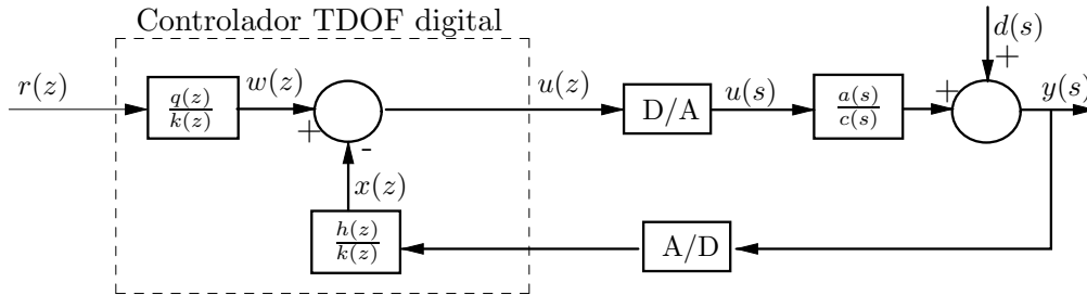
Figura D.1: Controlador TDOF digital
