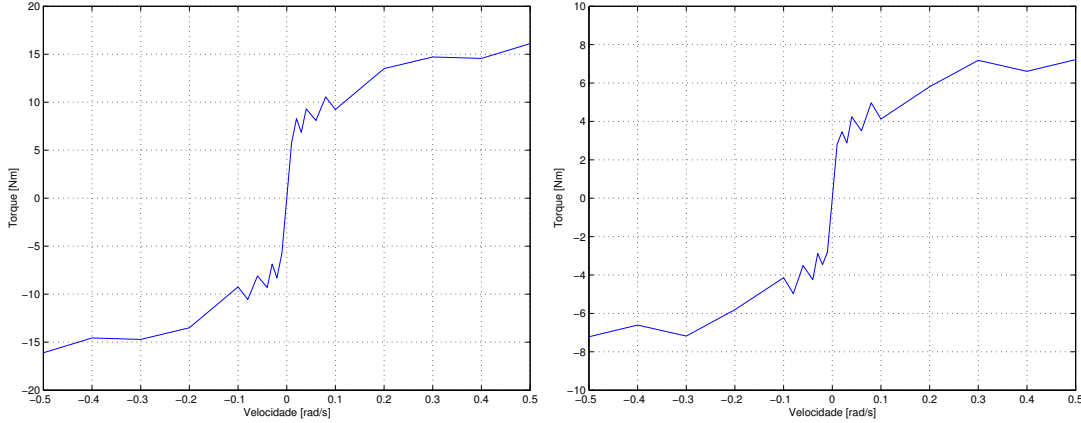
Figura 6.28: Atrito estático para as juntas 0 e 1
