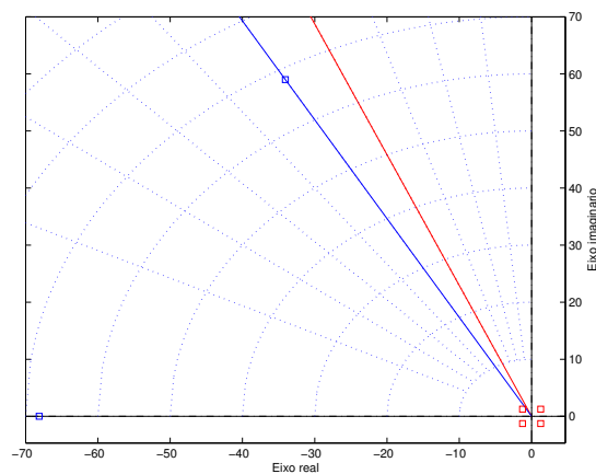
Figura 6.4: Pólos ótimos
