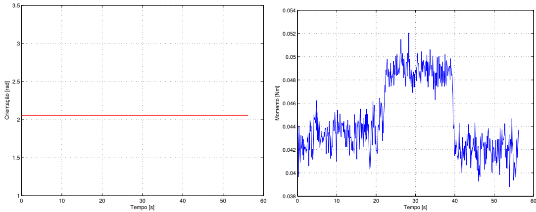
Figura 7.16: Posição angular e momento na direção \theta - controle PI
