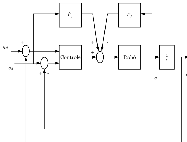
Figura 3.8: Observador de atrito baseado na velocidade desejada
