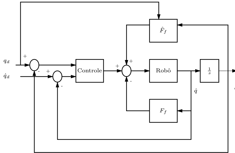
Figura 3.6: Observador de atrito baseado no erro de posição
