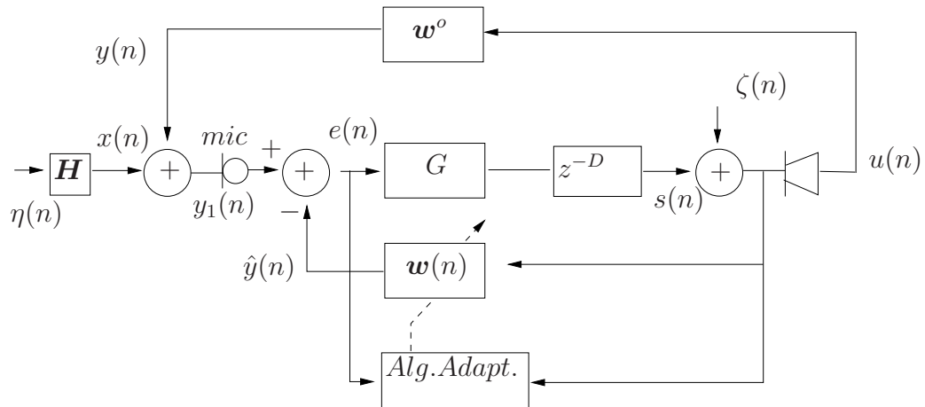
Figura 2.5: Diagrama em blocos de um sistema típico de cancelamento adaptativo de retroalimentação em aparelhos auditivos
