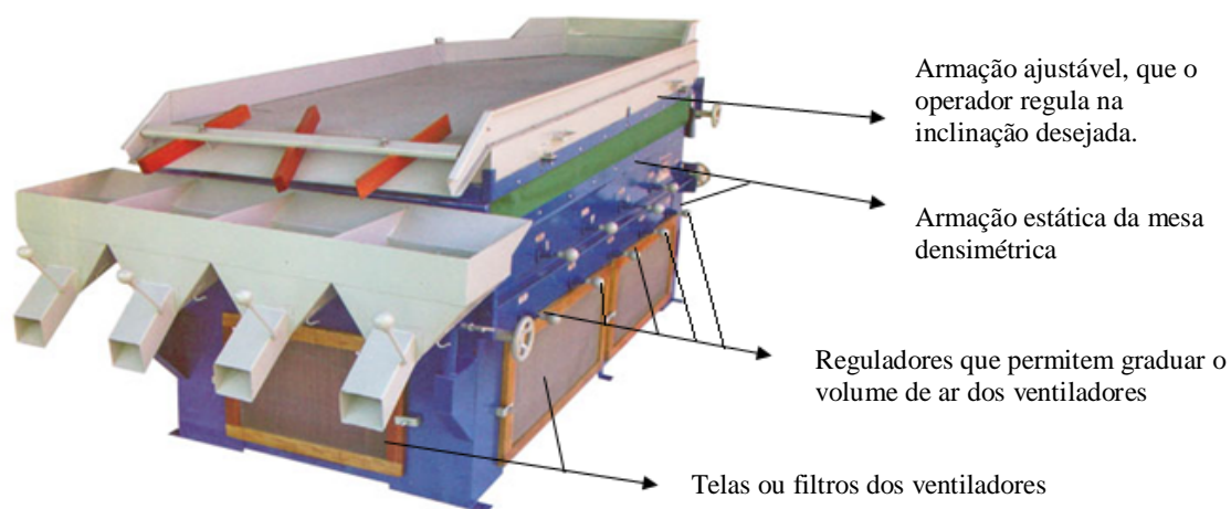
Figura 3: Mesa densimétrica.
