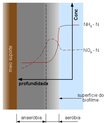
Figura 3.16. Perfil de nitrogênio no biofilme. Adaptado de Iwai e Kitao (1994) por Gebara (2006)
