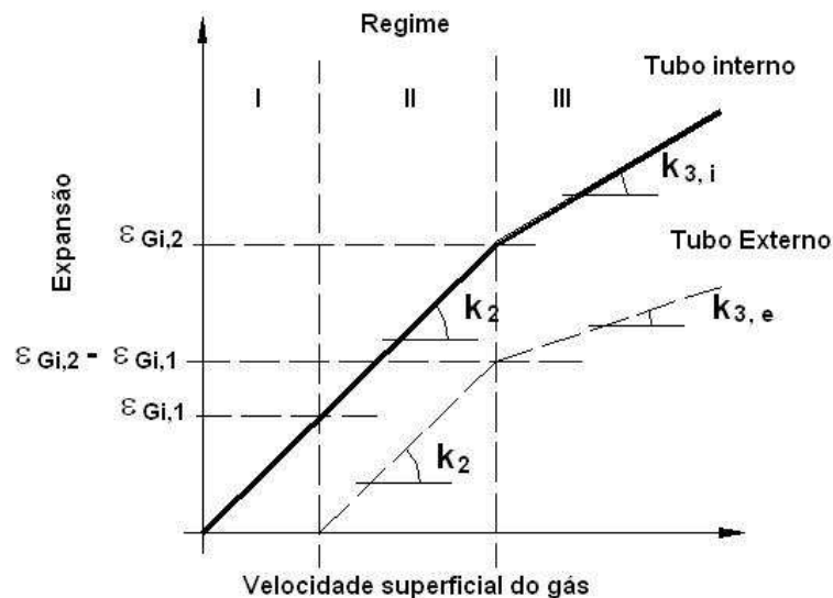
Figura 3.6. Representação esquemática da expansão no tubo interno e externo em função da velocidade superficial do gás. Adaptado de Van Benthum et al. (1999)
