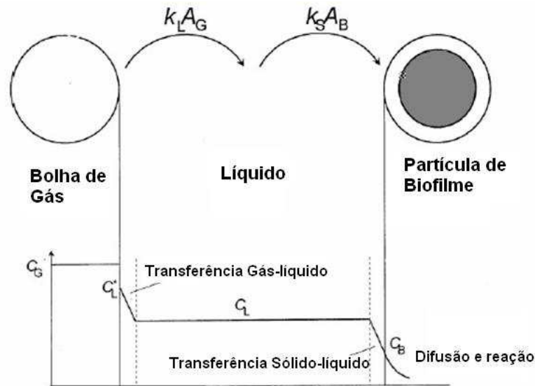
Figura 3.8. Transferência de massa em reatores trifásicos. Adaptado de Nicoletta et al. (1999)
