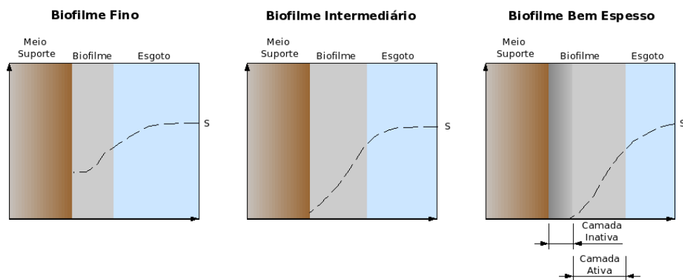
Figura 3.12. Gradientes de concentração de substrato (S) em biofilmes de diferentes espessuras. Adaptado de Von Sperling (1996) por Gebara (2006)
