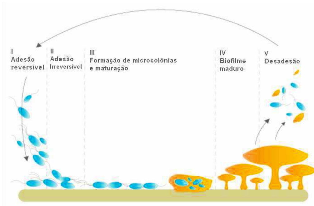
Figura 3.10. Representação esquemática das etapas de desenvolvimento de biofilme (modelo para Pseudomonas aeruginosa ). Adaptado de Ghigo et al. (2003) por Grupo de Ciências Biológicas – GCB (2008)
