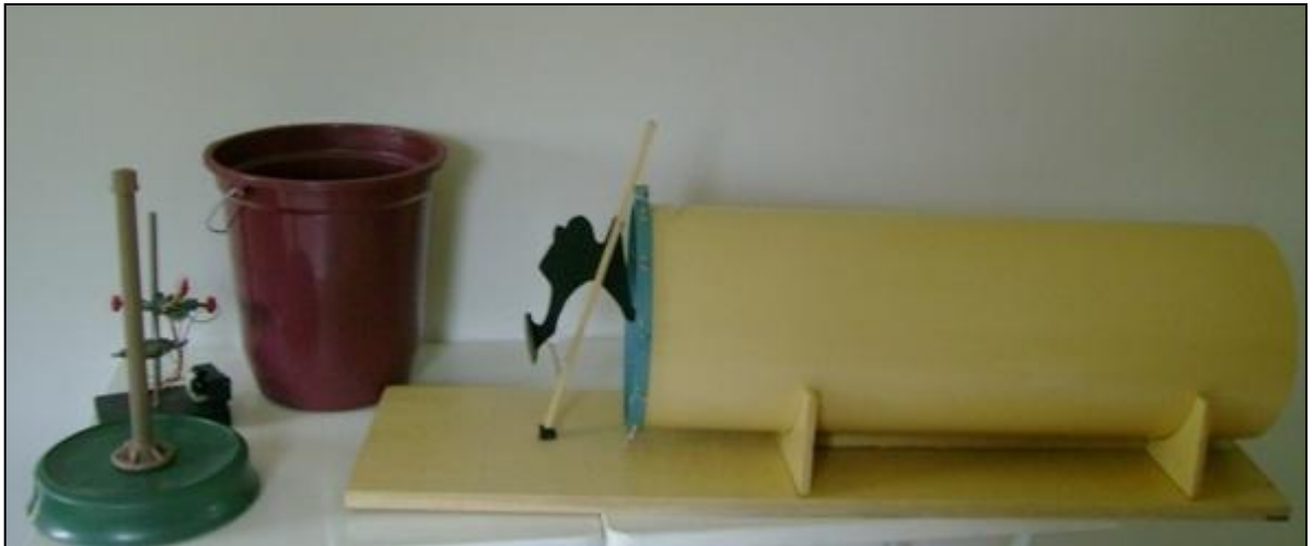
Figura 10 - Dispositivo ouvido mecânico - utilizado para representar o ouvido externo e o médio.
