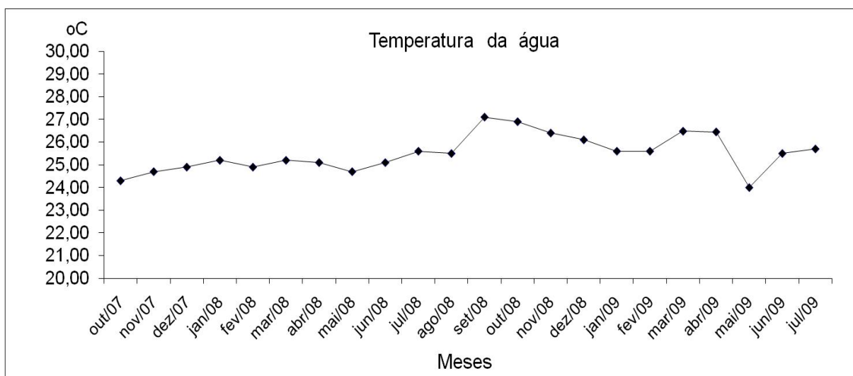
Figura 24 - Distribuição dos valores médios mensais da temperatura da água (°C) em todos os pontos amostrais, no período de outubro de 2007 a julho de 2009.
