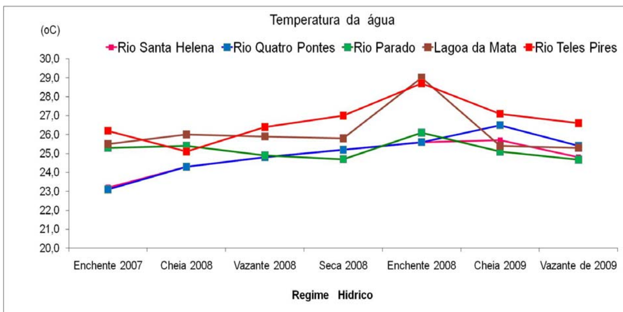
Figura 25 - Distribuição dos valores médios da temperatura da água (°C) em função das fases do regime hídrico nas áreas de coleta, no período de outubro de 2007 a julho de 2009
