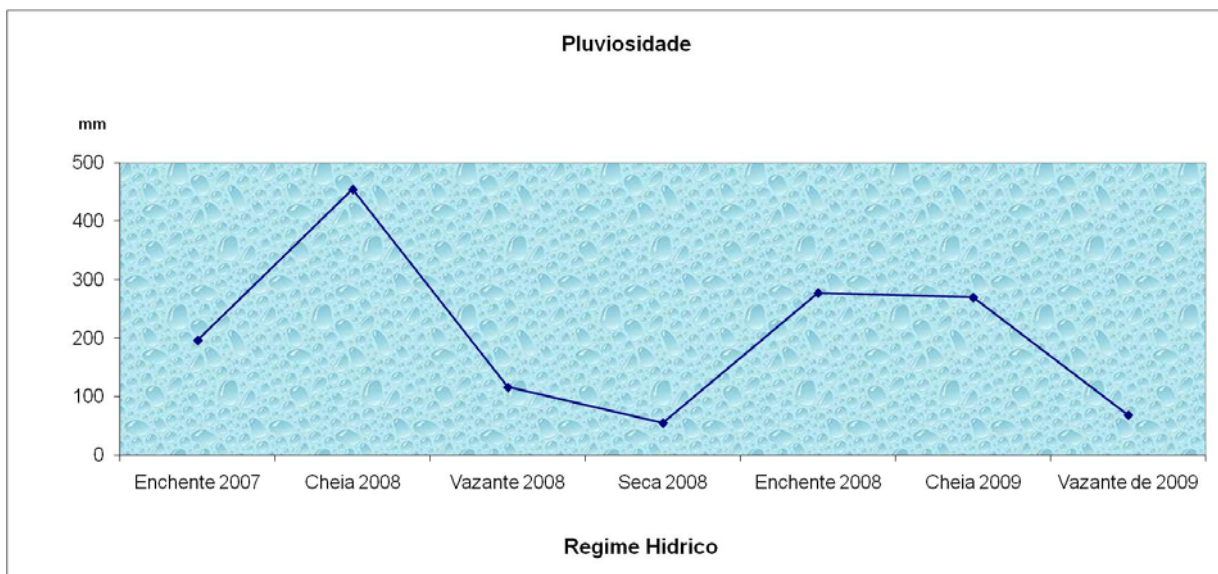
Figura 15 - Distribuição dos valores médios de pluviosidade (mm) em relação ao regime hídrico, no período de outubro de 2007 a julho de 2009, na região de Alta Floresta-MT. Fonte: INFRAERO-Aeroporto de Alta Floresta-MT (Estação Meteorológica de Superfície)
