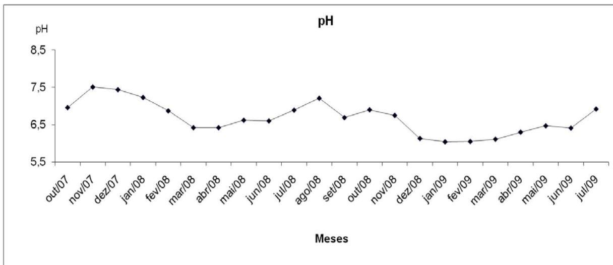
Figura 18 - Distribuição dos valores médios mensais do pH da água em todos os pontos amostrais, na região de Alta Floresta-MT, no período de outubro de 2007 a julho de 2009.
