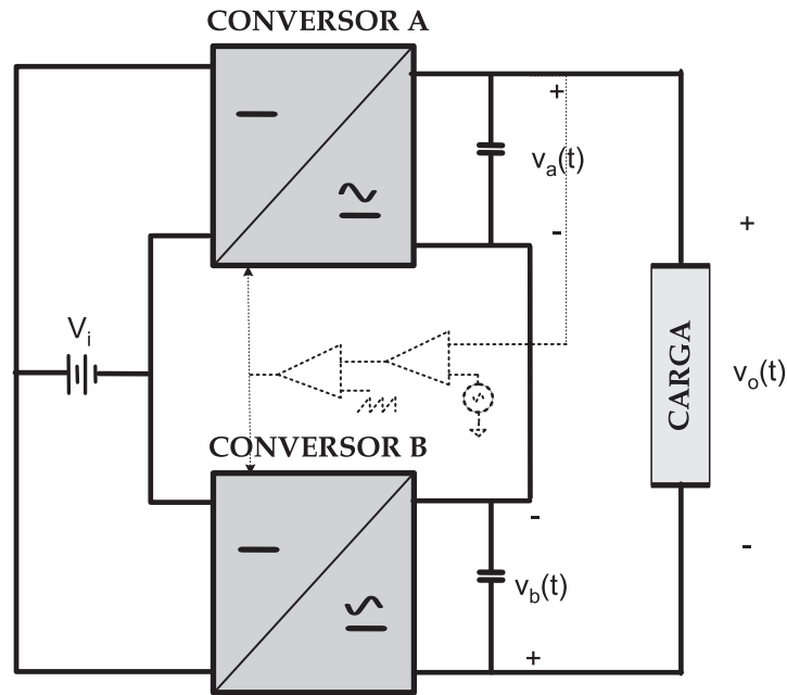
Figura 1.16: Diagrama de blocos ilustrando o princípio da geração da conexão diferencial de conversores CC-CC bidirecionais.
