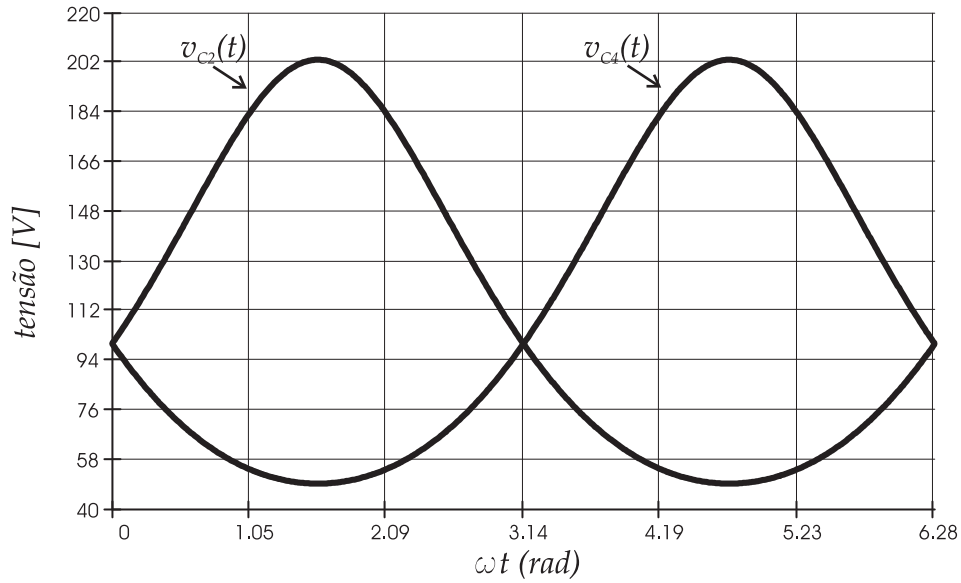
Figura 5.2: Tensão nos capacitores, v_{C2} e v_{C4}
