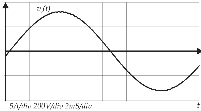
Figura 4.49: Tensão de saída v_o(t) obtida por simulação.
