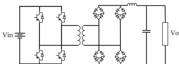
Figura 1.11: Esquemático do conversor CC-CA bidirecional baseado em conversor de frequência.
