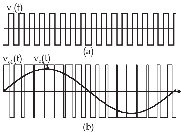
Figura 1.8: (a) Traçado da forma da onda da tensão aplicada ao primário do transformado, (b) Traçado das formas de onda da saída após o conversor de frequência.
