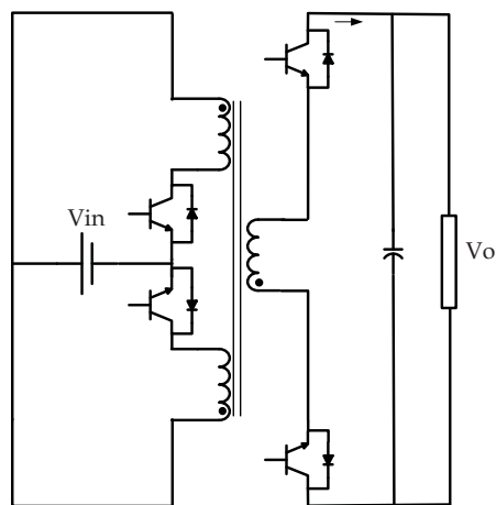
Figura 1.15: Conversor flyback CC-CA bidirecional proposto por Skinner.
