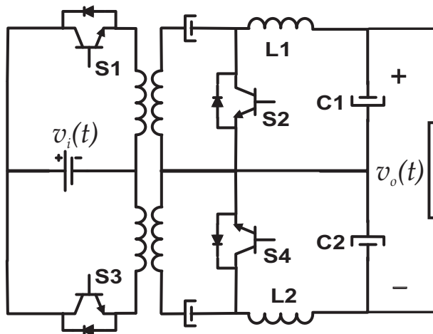
Figura 3.10: Conversor Zeta CC-CA bidirecional isolado.
