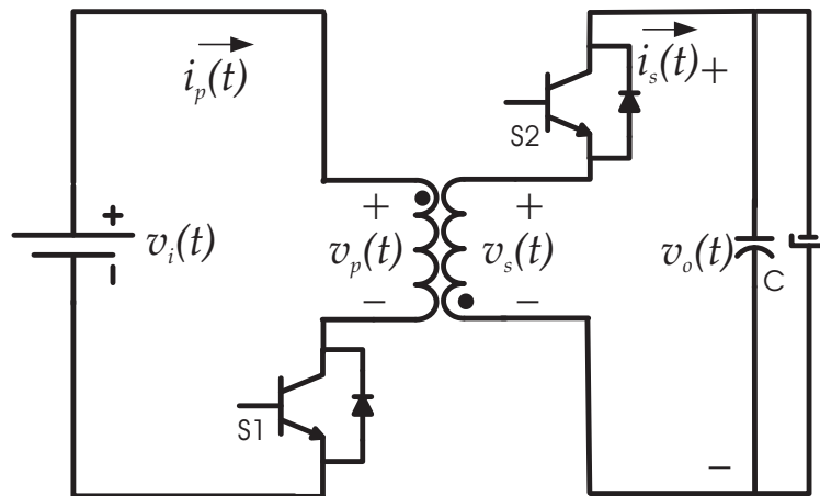
Figura 4.14: Conversor flyback CC-CC bidirecional com carga capacitiva.
