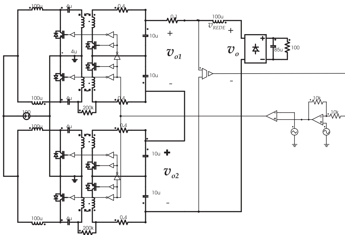
Figura 7.1: Associação de dois conversores SEPIC bidirecional isolados em alta freqüência.
