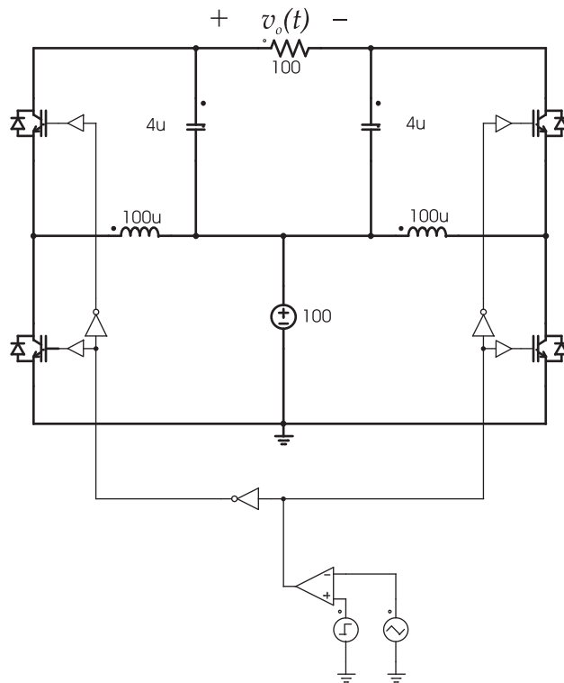
Figura 4.40: Inversor flyback simulado.
