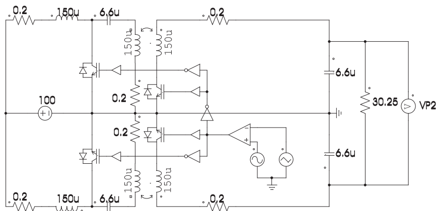
Figura 6.9: Inversor SEPIC com carga resistiva simulado em malha aberta.
