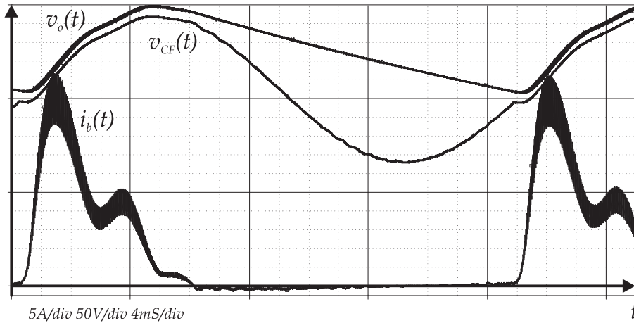
Figura 4.18: Tensões de saída v_o(t) , carga v_{CF}(t) e corrente da bateria, obtida por simulação.
