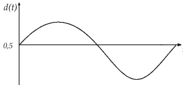
Figura 4.8: Razão cíclica para que seja obtida uma a tensão senoidal com nível CC na saída.
