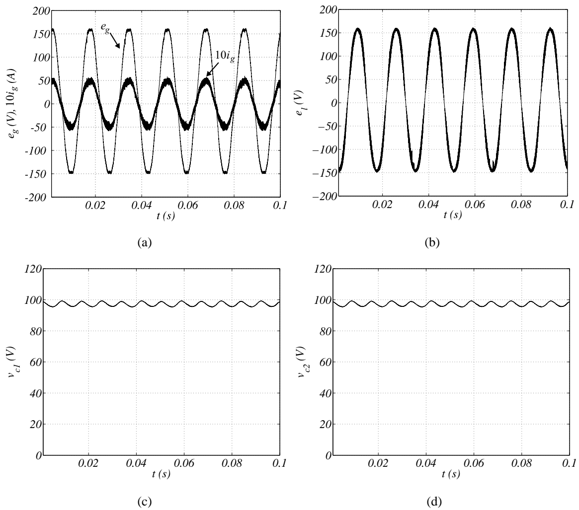
Figura 7.12: Resultados experimentais em regime permanente - 2P - \mu = 0,5 . (a) Tensão e corrente da rede monofásica. (b) Tensão da carga. (c) Tensão do barramento CC do conversor 1. (d) Tensão do barramento CC do conversor 2.
