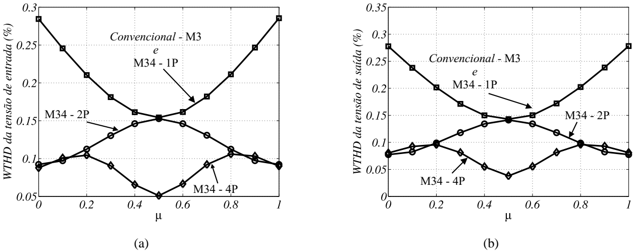
Figura 5.6: Curvas da WTHD das topologias M34 e convencional M3. (a) Tensão de entrada, v_g . (b) Tensão de saída, v_l .
