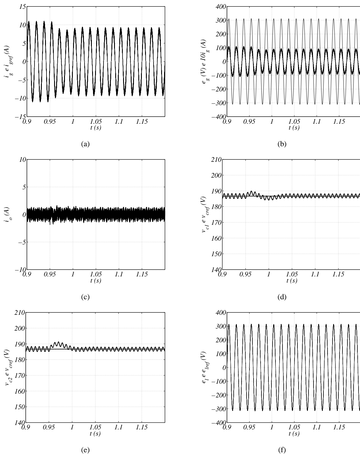
Figura 7.2: Resultados de simulação com transitório de carga da topologia série M34 (a) Corrente da rede monofásica. (b) Corrente da rede em fase com a tensão da rede. (c) Corrente de circulação i_o . (d) Controle da tensão do barramento CC do conversor 1. (e) Controle da tensão do barramento CC do conversor 2. (f) Tensão na carga, e_l .
