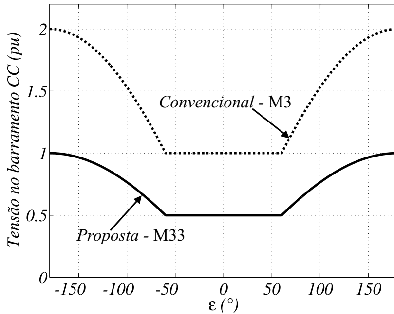
Figura 6.2: Tensão no barramento CC das topologias M33 e M3 em função da diferença entre o ângulo da tensão de entrada e o ângulo da tensão de saída.
