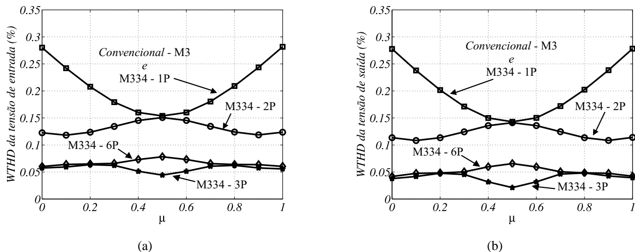
Figura 5.16: Curvas da WTHD das topologias M334 e convencional M3. (a) Tensão de entrada, v_g . (b) Tensão de saída, v_l .
