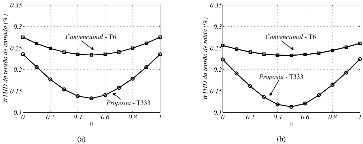
Figura 8.3: Curvas da WTHD das topologias T333 e convencional T6. (a) Tensão de entrada, v_{ak} , com k = 1, 2 e 3 . (b) Tensão de saída, v_{bk} , com k = 1, 2 e 3 .
