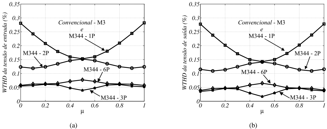
Figura 5.23: Curvas da WTHD das topologias M344 e convencional M3. (a) Tensão de entrada, v_g . (b) Tensão de saída, v_l .
