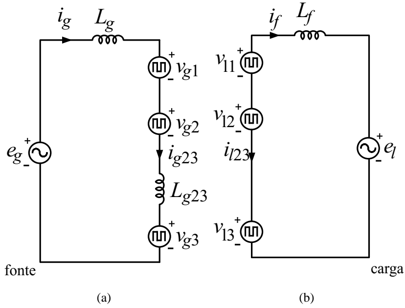
Figura 4.2: (a) Representação da entrada do sistema M334. (b) Representação da saída do sistema M334.
