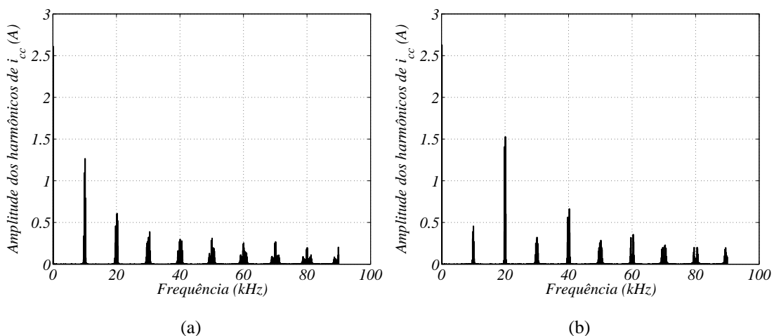
Figura 6.3: Espectro da corrente do barramento CC da topologia convencional M3. (a) \mu = 0 . (b) \mu = 0,5 .
