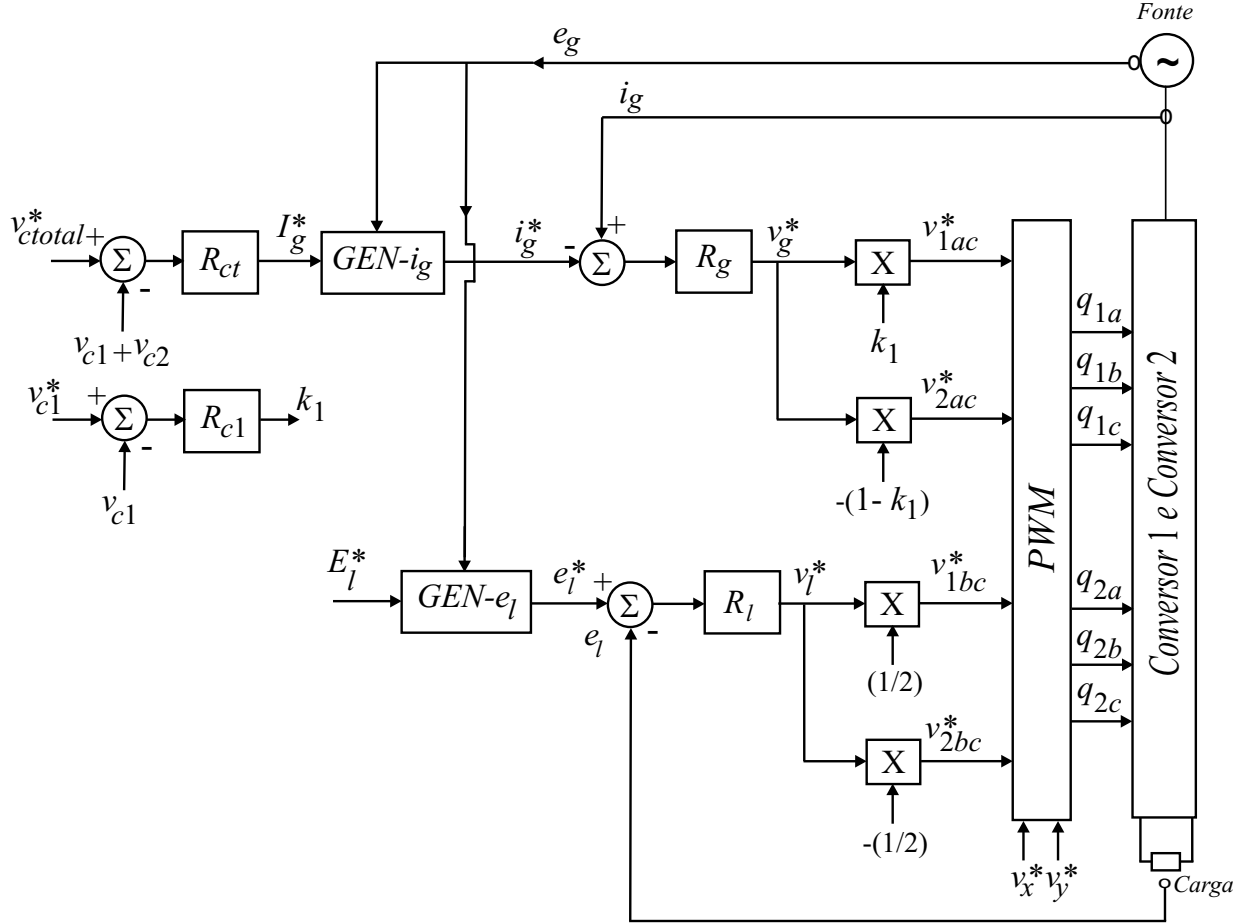
Figura 3.4: Diagrama de controle da topologia M33.
