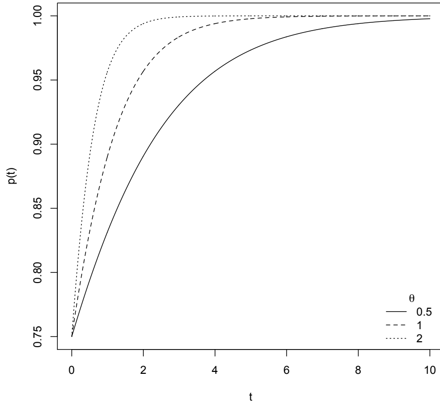
FIGURA 4.1: Função probabilidade de imunes do modelo exponencial para diferentes valores de \theta .
