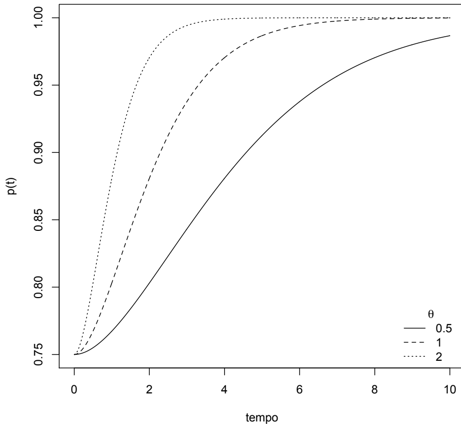
FIGURA 4.3: Função probabilidade de imunes do modelo exponencial length biased para diferentes valores de \theta .
