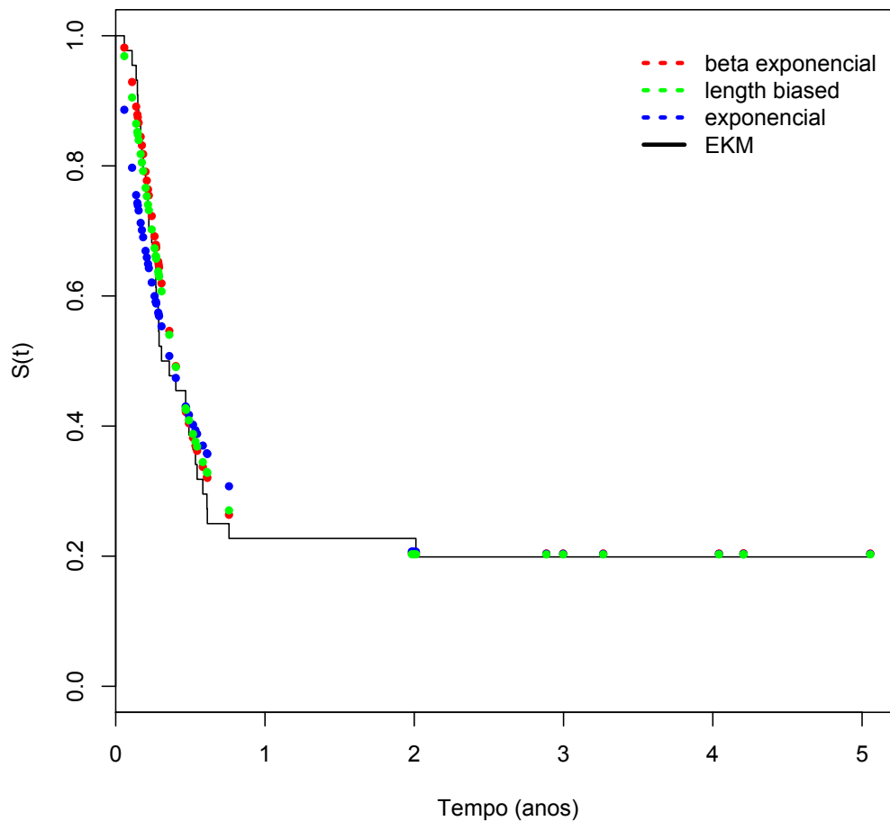
FIGURA 4.8: Curvas de sobrevivência previstas por cada um dos modelos para o grupo 2 e estimativa de Kaplan-Meier.
