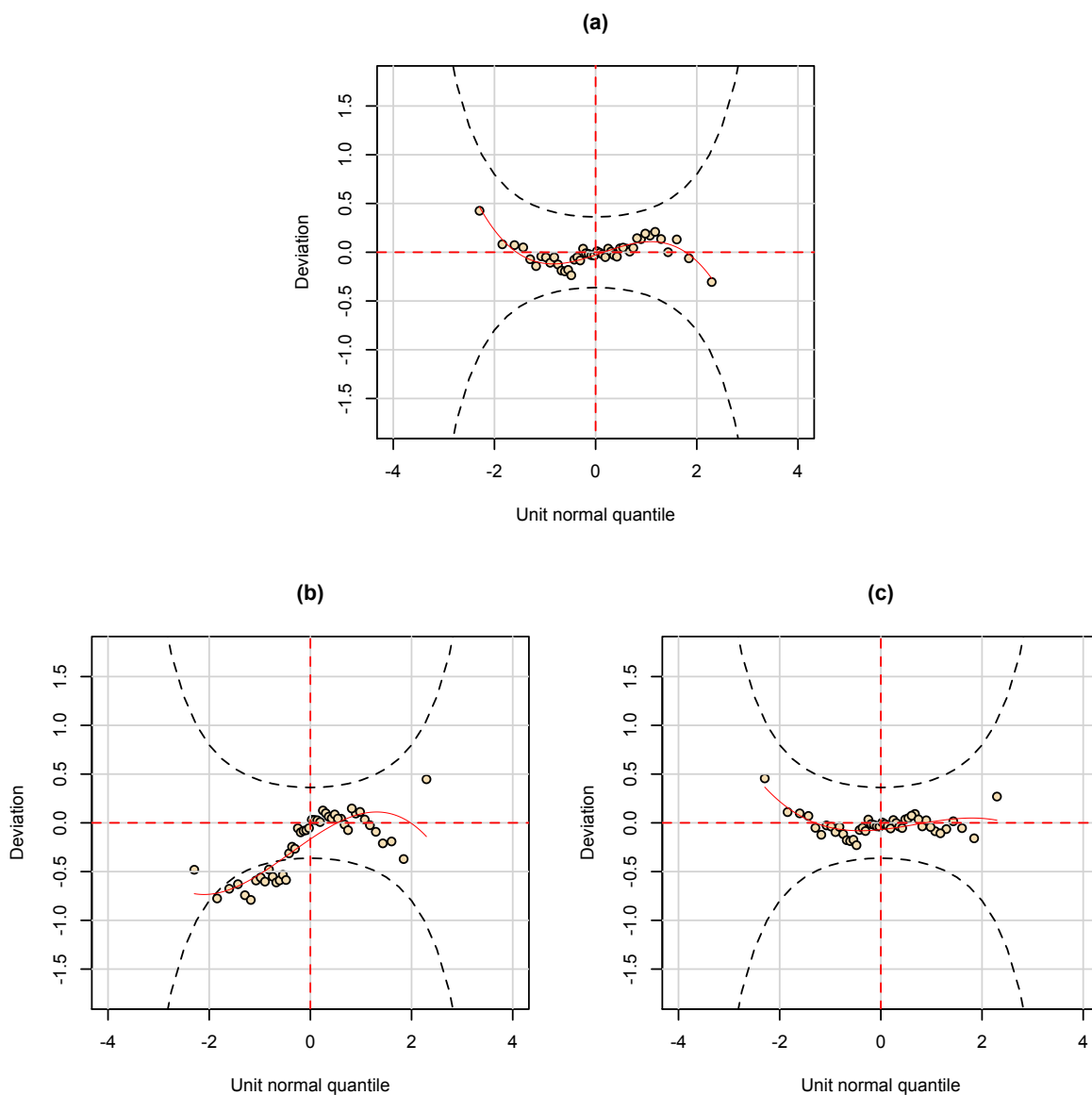
FIGURA 4.5: Gráficos wormplot : (a) exponencial (b) length biased e (c) beta exponencial.
