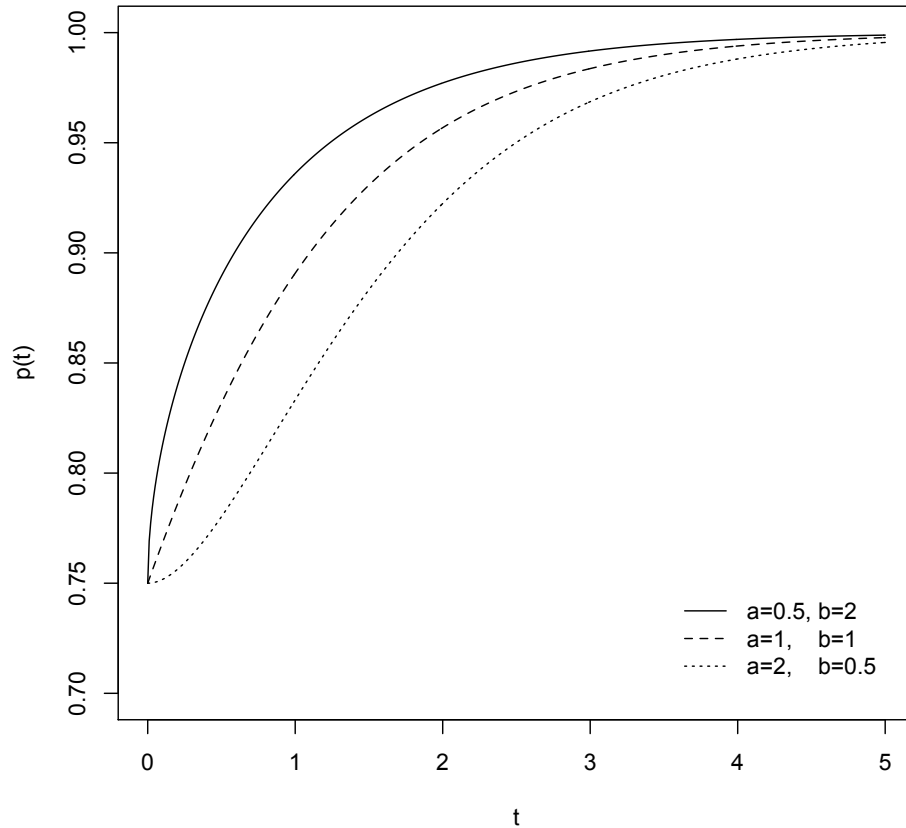
FIGURA 4.4: Função probabilidade de imunes do modelo beta exponencial para diferentes valores de (a, b) .
