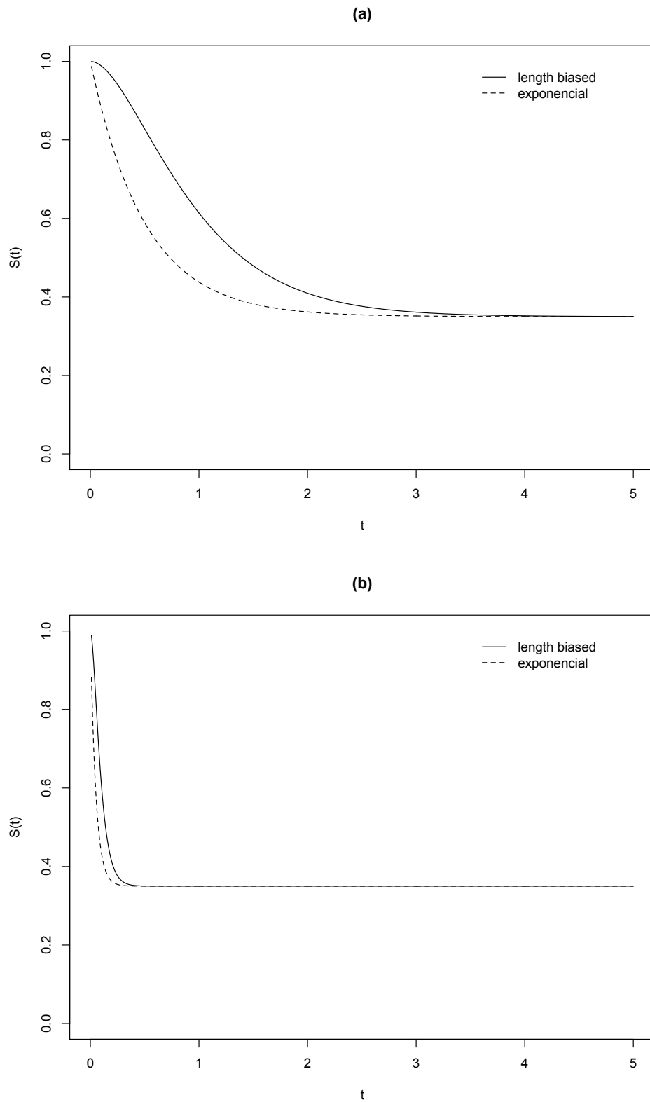
FIGURA 4.2: Funções de sobrevivência do modelo exponencial e exponencial length biased : (a) \theta = 2 e (b) \theta = 20
