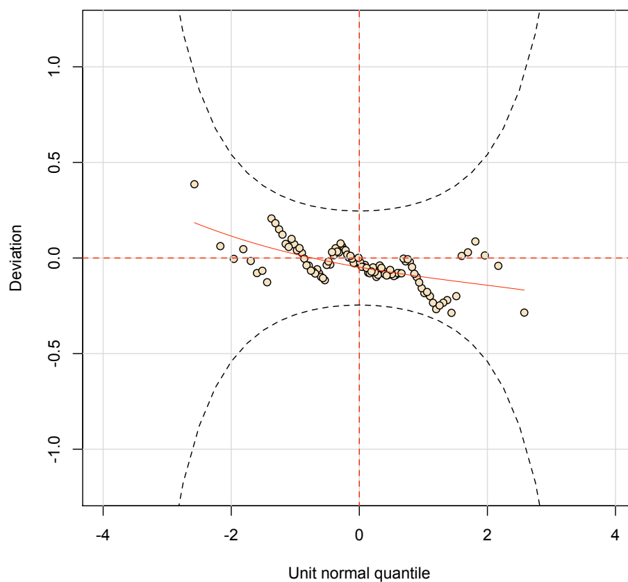
FIGURA A.2: Gráfico wormplot .
