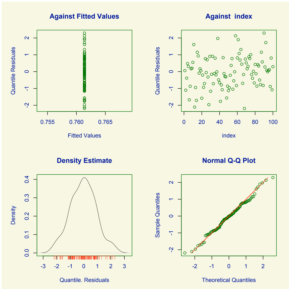
FIGURA A.1: Gráficos dos resíduos, densidade estimada e QQ-Plot.
