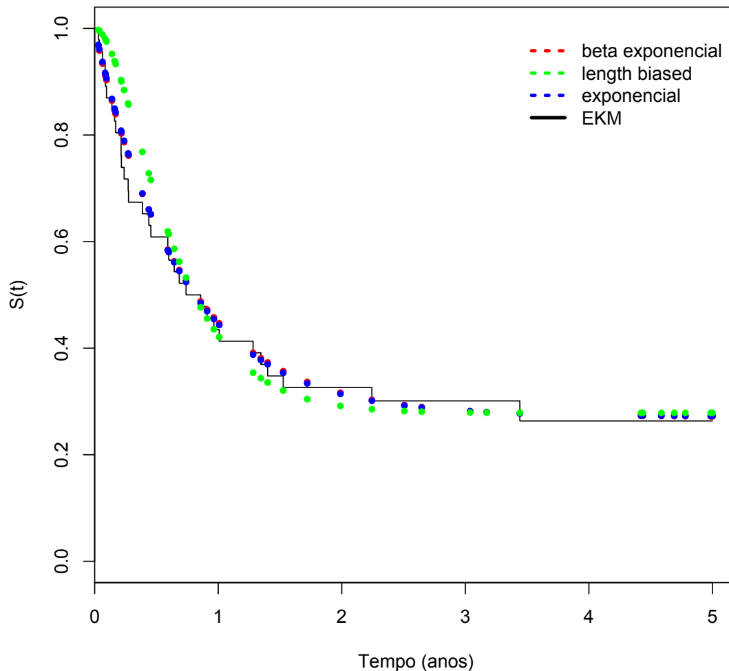
FIGURA 4.6: Curvas de sobrevivência previstas por cada um dos modelos para o grupo 1 e estimativa de Kaplan-Meier.
