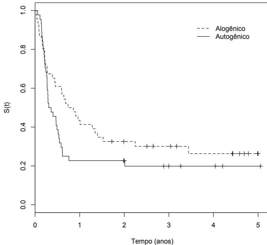
FIGURA 2.1: Estimativa de Kaplan-Meier de acordo com o tipo de transplante.
