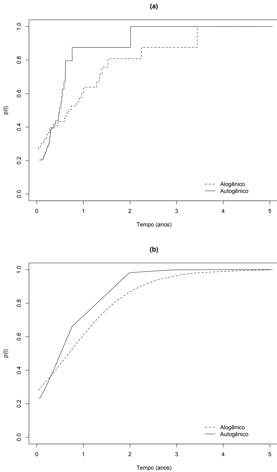
FIGURA 2.2: Funções probabilidade de imunes (a) estimativa não-paramétrica e (b) estimativa paramétrica
