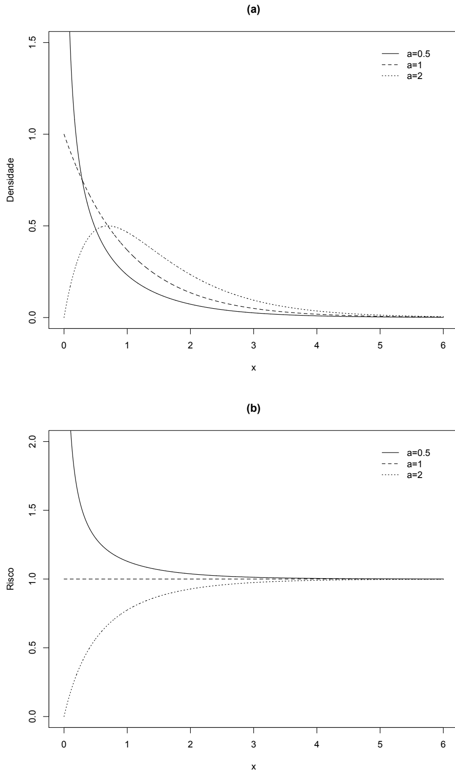
FIGURA 3.3: Função densidade(a) e risco (b) da distribuição beta exponencial para diferentes valores de a
