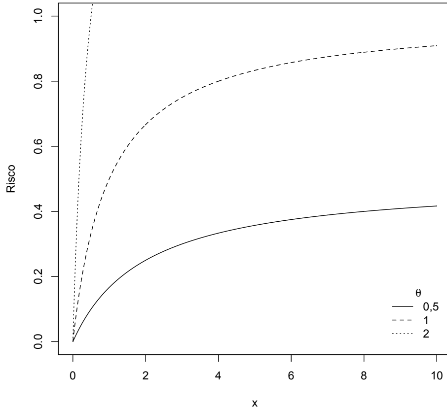
FIGURA 3.2: Função de risco da distribuição exponencial length biased para diferentes valores de \theta
