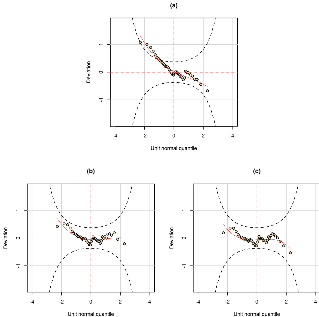
FIGURA 4.7: Gráficos wormplot : para o grupo 2 (a) exponencial (b) length biased e (c) beta exponencial
