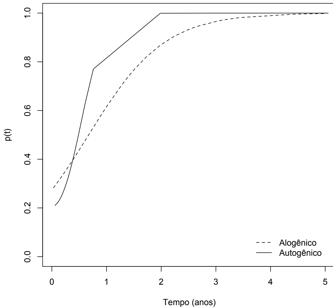
FIGURA 4.9: Função probabilidade de imunes do modelo beta exponencial para os dois grupos
