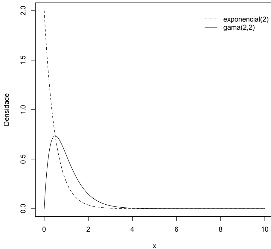
FIGURA 3.1: Comparação de uma distribuição exponencial com uma exponencial length biased
