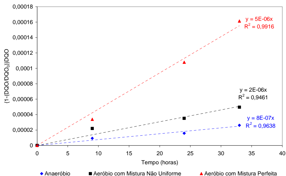
Figura 36: Ajuste linear de uma equação de segunda ordem para a cinética de degradação da Demanda Química de Oxigênio (DQO) do efluente, inoculado com a cepa específica de gorduraklin, nas primeiras horas de biodegradação, em diferentes condições operacionais, frente à disponibilidade de oxigênio e efeitos hidrodinâmicos.
