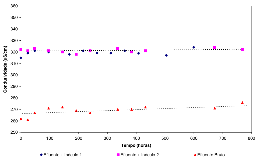
Figura 24: Variação da condutividade do efluente bruto e inoculado com esgoto doméstico, ao longo do processo de biodigestão anaeróbia.
