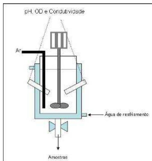
Figura 5: Esquema do reator biológico aeróbico.
