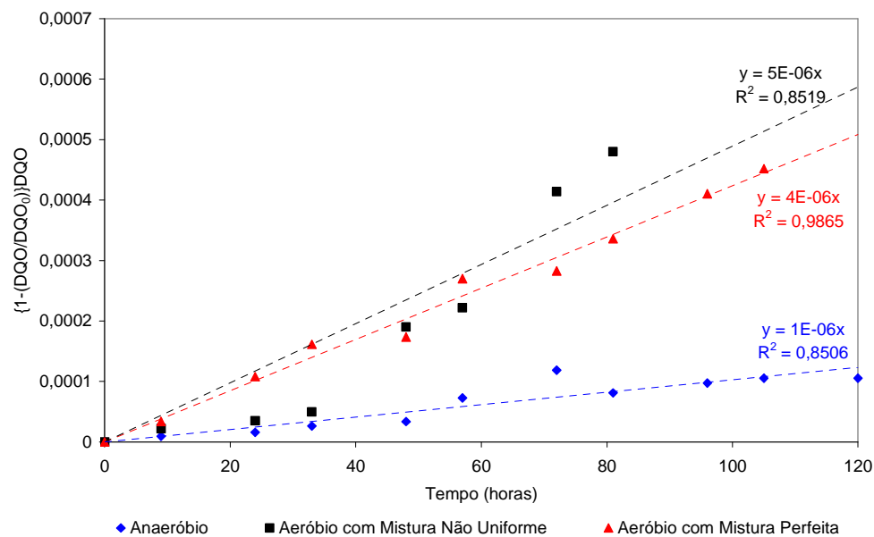
Figura 35: Ajuste linear de uma equação de segunda ordem para a cinética de degradação da Demanda Química de Oxigênio (DQO) do efluente, inoculado com a cepa específica de gorduraklin, ao longo do processo de biodegradação, em diferentes condições operacionais, frente à disponibilidade de oxigênio e efeitos hidrodinâmicos.
