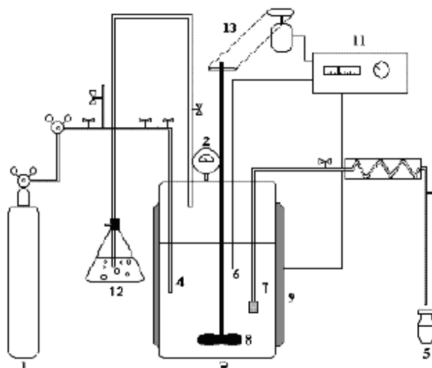
Figura 6: Módulo Experimental dos Ensaio de Oxidação Úmida Catalítica.
