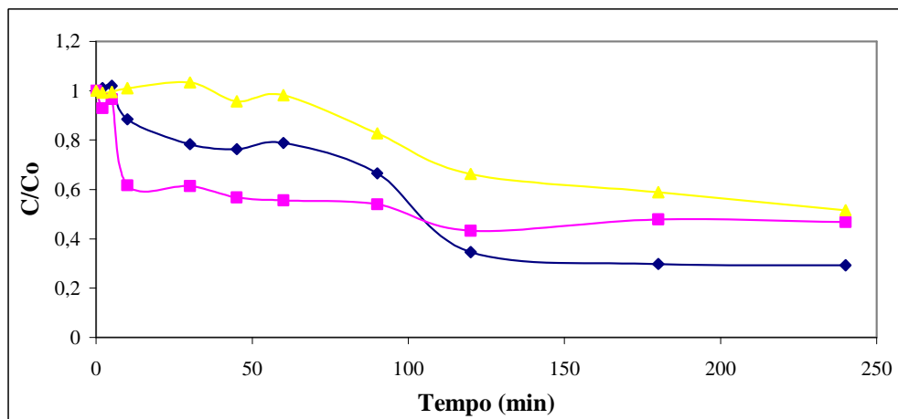
Figura 49: Frações residuais de LCC em foto-Fenton nos ensaios (♦) 1, (■) 3, (▲) 5, C_0 = 0,8\text{g/L} , de acordo com o planejamento da tabela 3.
