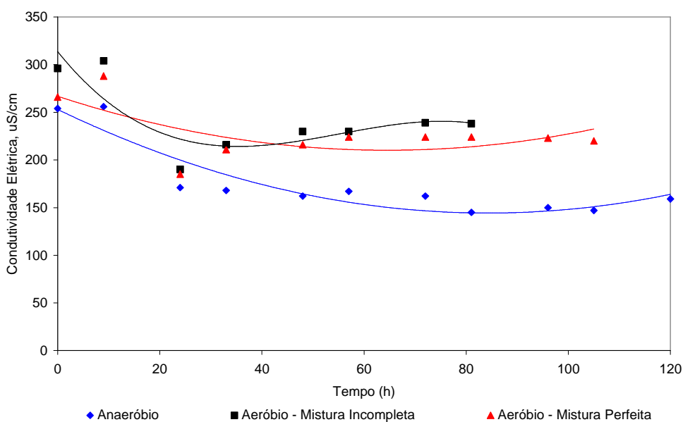
Figura 31: Variação da condutividade elétrica do efluente, inoculado com a cepa específica de gorduraklin, ao longo do processo de biodegradação, em diferentes condições operacionais, frente à disponibilidade de oxigênio e efeitos hidrodinâmicos.
