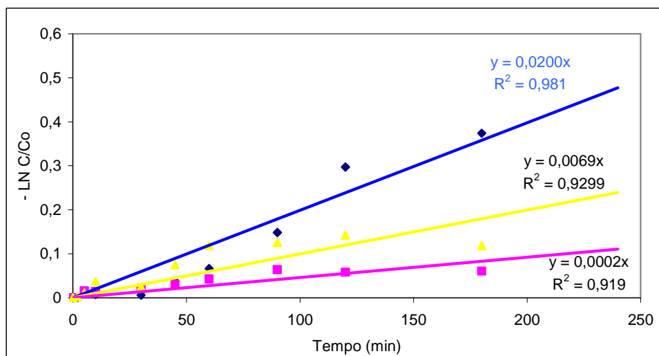
Figura 50: Frações residuais de LCC em UV-peróxido (◆), (▲) foto-Fenton e (■) Fenton, C_0=0,8 g/L, de acordo com o planejamento.
