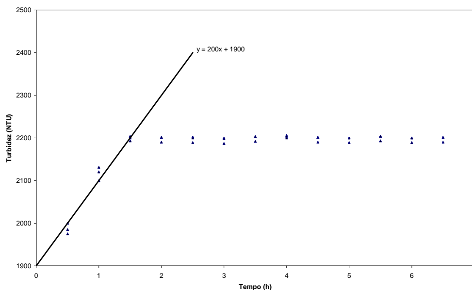
Figura 21: Perfil da turbidez ao longo da produção do efluente final.
