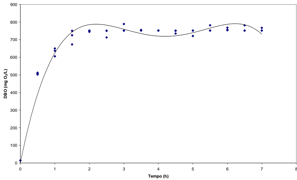
Figura 19: Cinética de contribuição da DBO nos efluentes formados.
