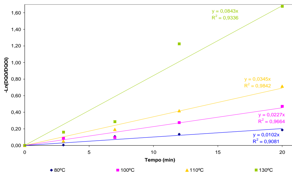
Figura 42: Ajuste linear de uma equação de pseudoprimera ordem para a cinética de degradação da Demanda Química de Oxigênio (DQO) do efluente em oxidação úmida catalítica em quatro diferentes níveis de temperatura.
