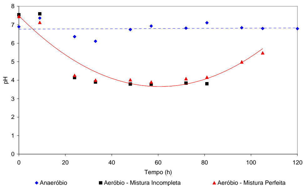
Figura 30: Variação do pH do efluente, inoculado com a cepa específica de gorduraklin, ao longo do processo de biodegradação, em diferentes condições operacionais, frente à disponibilidade de oxigênio e efeitos hidrodinâmicos.
