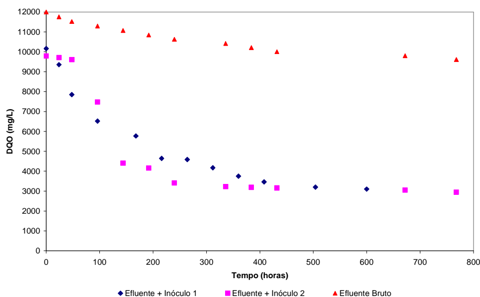
Figura 28: Variação da DQO remanescente no efluente bruto e inoculado com esgoto doméstico, ao longo do processo de biodigestão anaeróbia.
