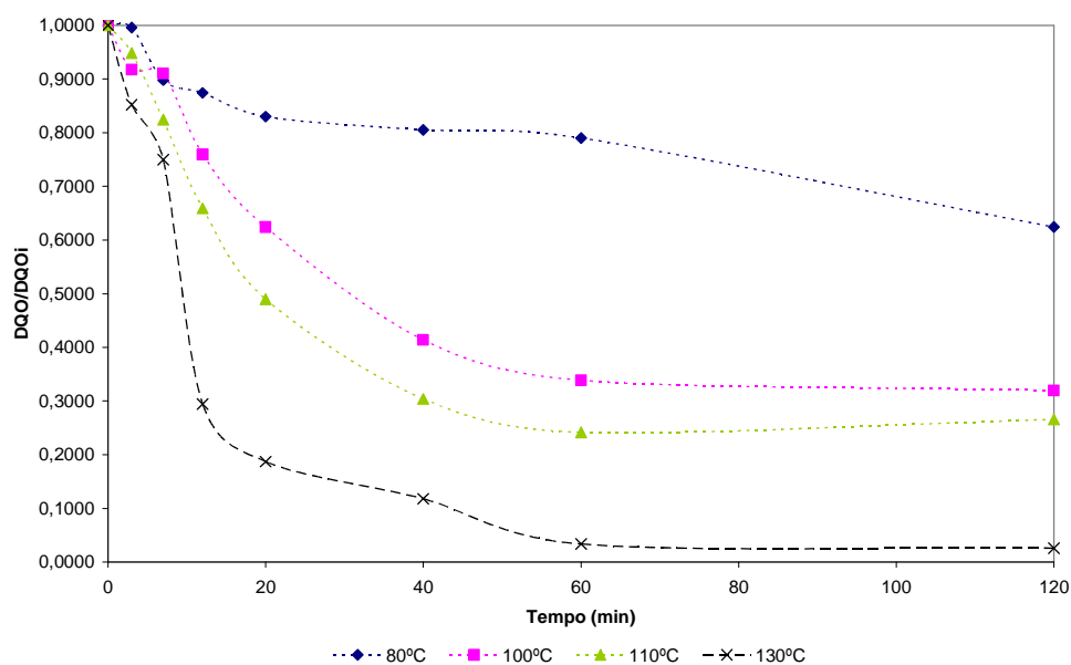
Figura 39: Frações residuais de LCC em oxidação catalisada por KMC a temperatura de (♦) 80 °C, (■) 100 °C, (▲) 110 °C, (X) 130 °C; C_i = 0,8 g/L, C_{\text{KMC}} = 5,0 g/L e P = 300 psi.
