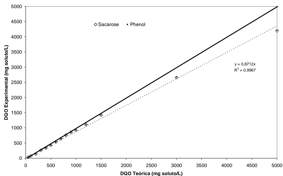
Figura 11: Comparação entre os valores experimentais e previstos para a DQO em efluentes sintéticos.
