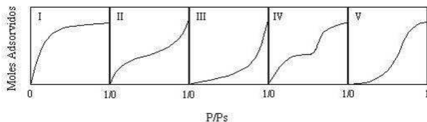
Figura 3: Classificação de Brunauer das Isotermas
