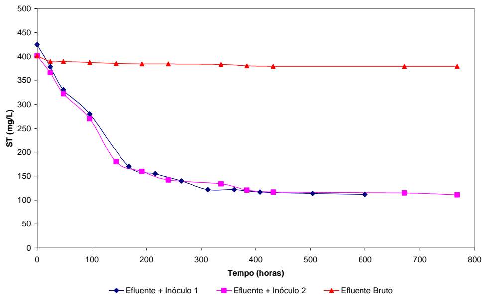
Figura 26: Variação dos sólidos totais do efluente bruto e inoculado com esgoto doméstico, ao longo do processo de biodigestão anaeróbia.
