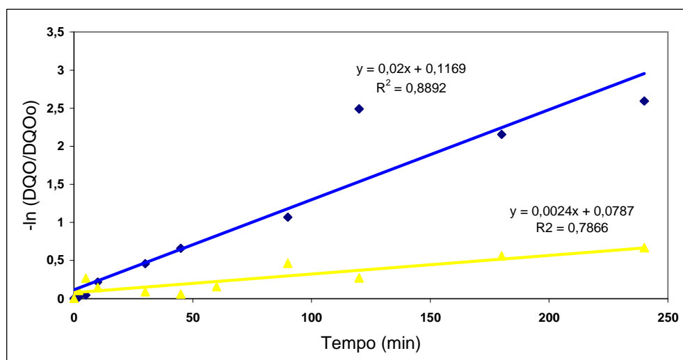
Figura 47: Frações residuais de LCC, ajustados a uma pseudo-primeira ordem, no tratamento UV-Peróxido nos ensaios (◆) 1, (▲) 3, C_0=0,8\text{g/L} , de acordo com o planejamento fatorial.
