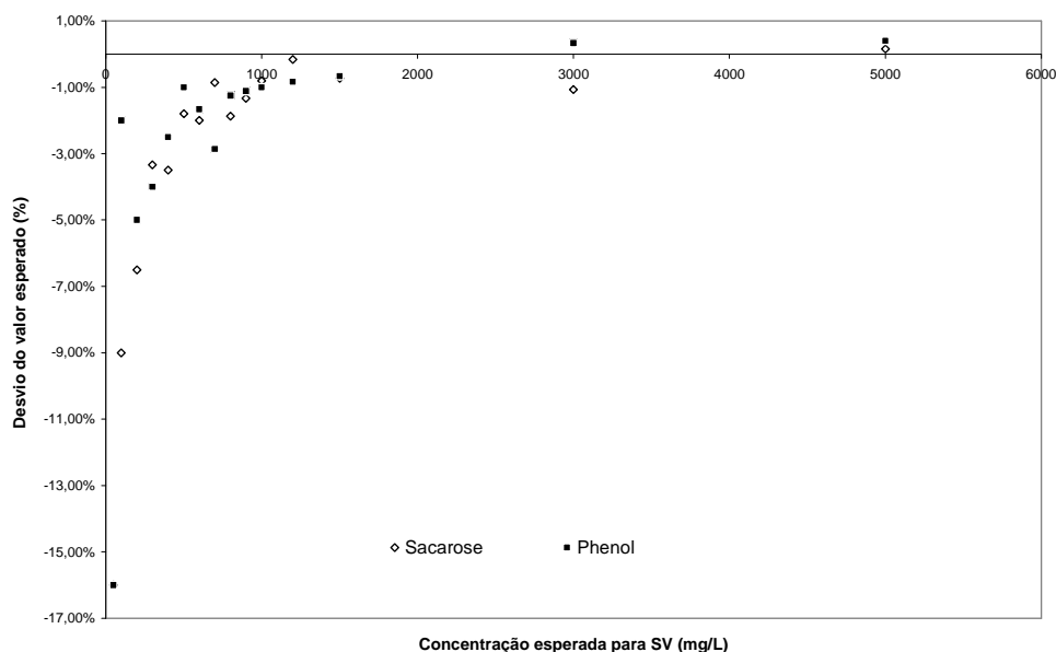
Figura 12: Comparação entre os valores experimentais e previstos para a SV em efluentes sintéticos.
