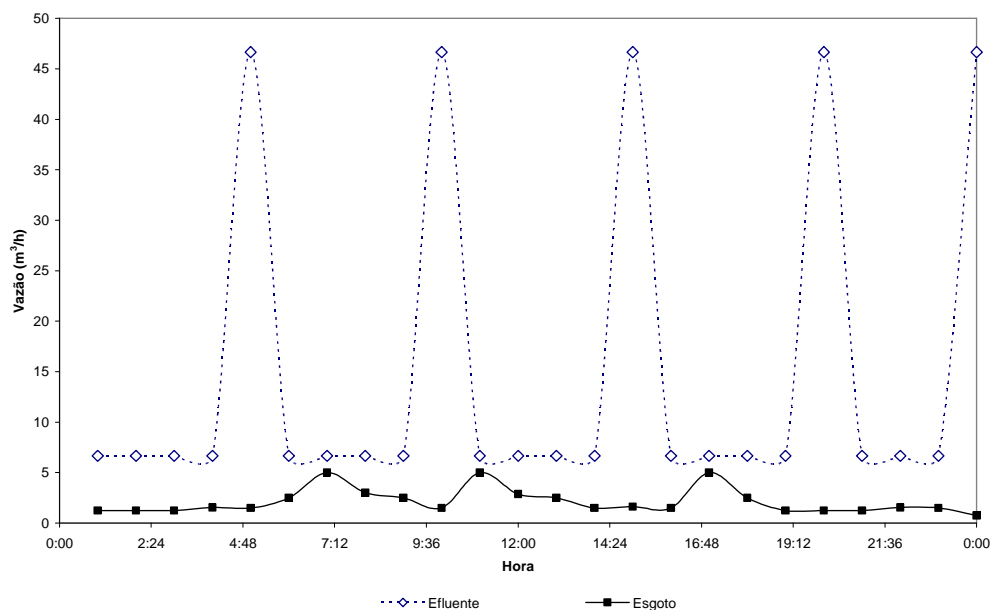
Figura 4: Vazões horárias dos efluentes industriais e esgotos sanitários da indústria de beneficiamento de castanha de caju utilizada para coleta de dados e efluentes.
