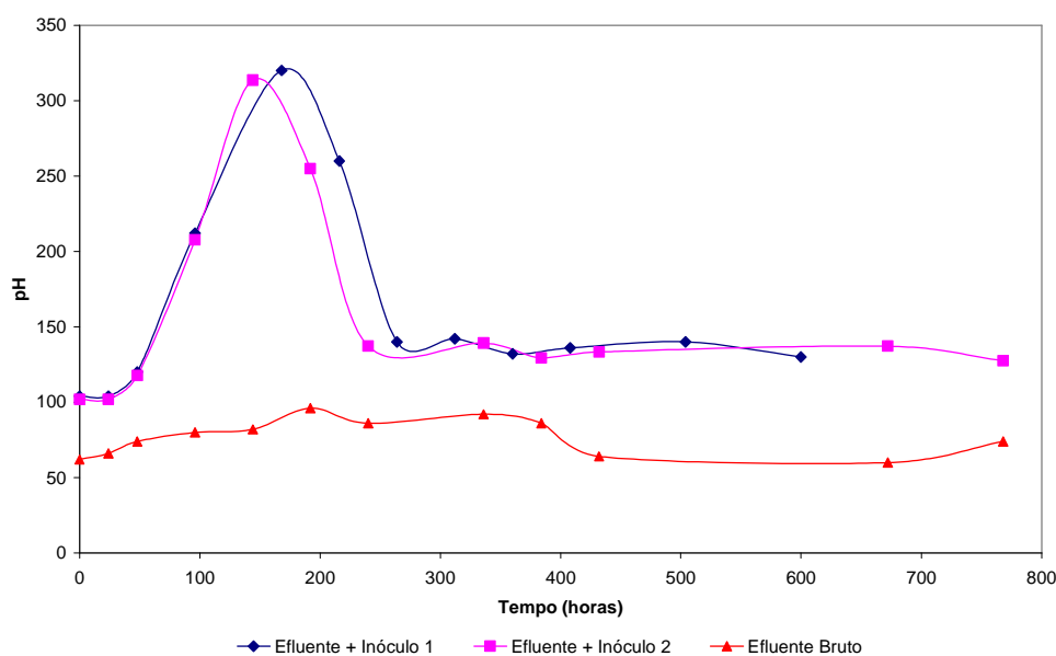
Figura 25: Variação de pH do meio do efluente bruto e inoculado com esgoto doméstico, ao longo do processo de biodigestão anaeróbia.
