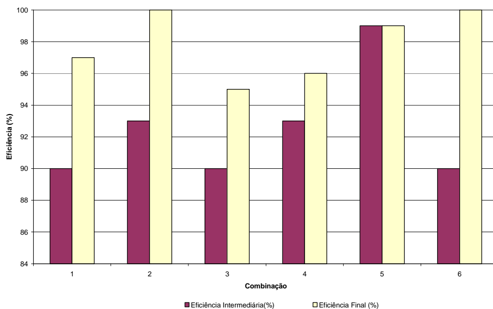
Figura 53: Resultados da eficiência de remoção da DQO nos ensaios combinados, nas condições experimentais otimizadas.
