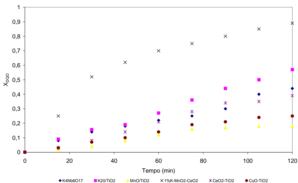
Figura 37: Conversão da DQO em função do tempo da reação.
