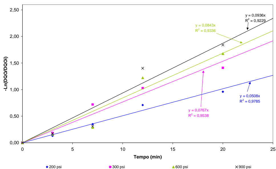
Figura 44: Ajuste linear de uma equação de primeira ordem para a cinética de degradação da Demanda Química de Oxigênio (DQO) do efluente em oxidação úmida catalítica em quatro diferentes níveis de pressão.
