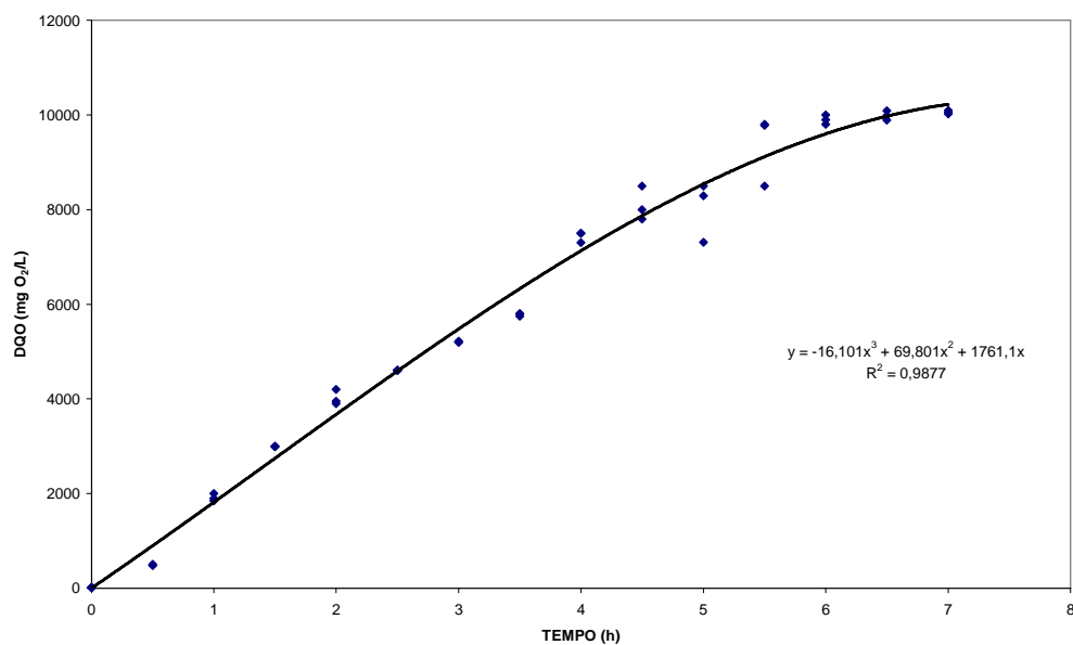
Figura 18: Perfil da concentração da DQO ao longo do processo de produção da batelada dos efluentes.
