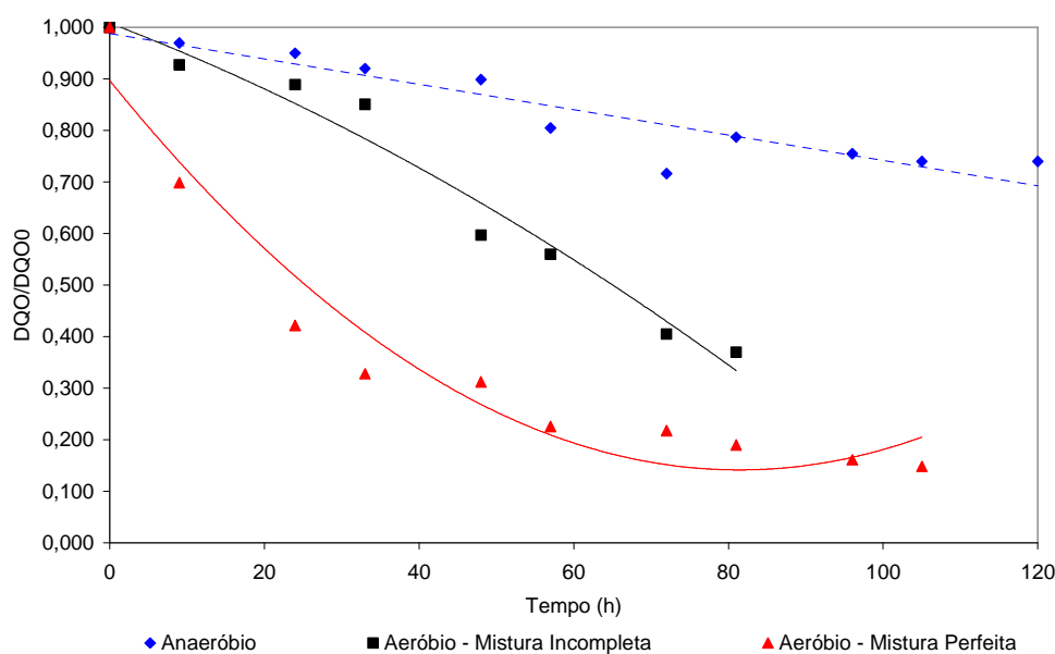
Figura 33: Variação do percentual de DQO remanescente do efluente, inoculado com a cepa específica de gorduraklin , ao longo do processo de biodegradação, em diferentes condições operacionais, frente à disponibilidade de oxigênio e efeitos hidrodinâmicos.
