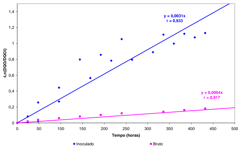
Figura 29: Ajuste linear de uma equação de primeira ordem para a cinética de degradação da Demanda Química de Oxigênio (DQO) do efluente bruto, e inoculado com esgoto doméstico, ao longo do processo de biodigestão anaeróbia.
