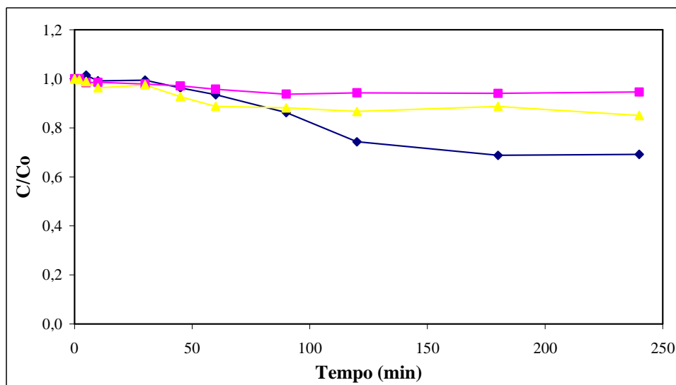
Figura 48: Frações residuais de LCC em Fenton nos ensaios (♦) 1, (▲) 3, (■) 5, C 0 = 0,8g/L, de acordo com o planejamento.
