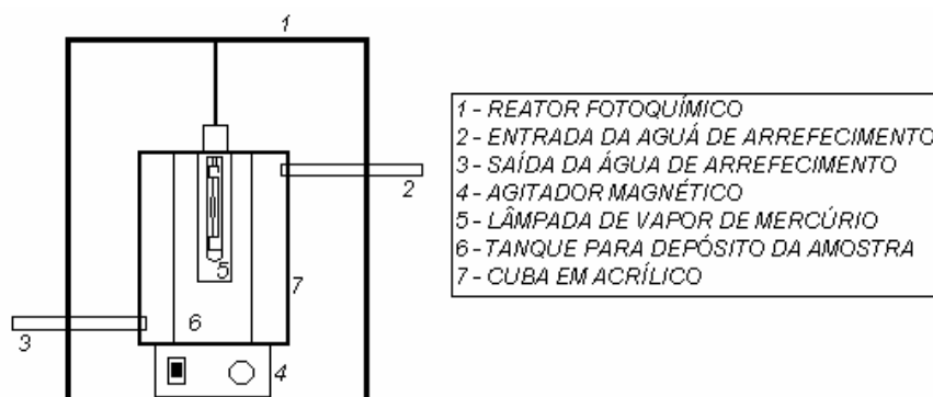
Figura 7: Equipamento utilizado para realizar os ensaios.
