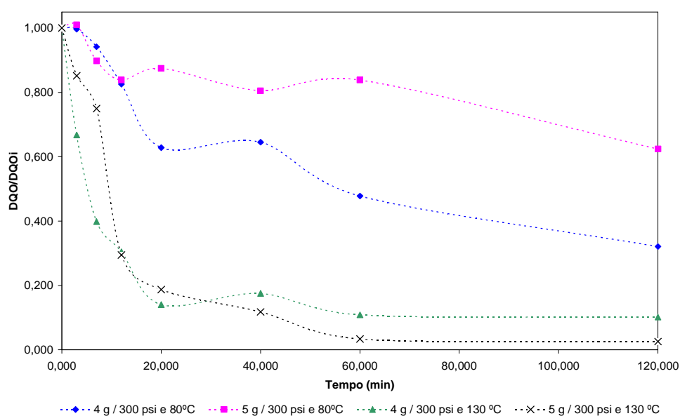
Figura 41: Frações residuais de LCC em quatro experimentos catalisados por K-MnO 2 /CeO 2 a concentrações de (♦) 4,0 g/L, (■) 5,0 g/L; Ci = 0,8 g/L, T = 80 °C e 130 °C e P = 300 psi.
