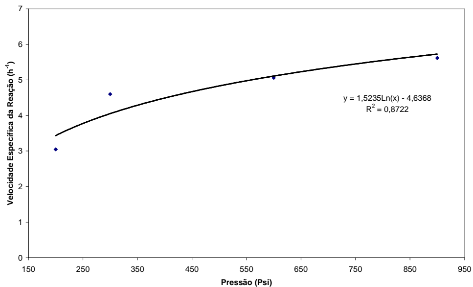
Figura 45: Velocidade Específica de Reação para a degradação da Demanda Química de Oxigênio (DQO) do efluente em oxidação úmida catalítica em função da pressão.
