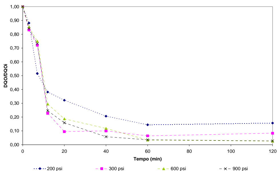
Figura 40: Frações residuais de LCC em oxidação catalisada por KMC a pressão de (◆) 200 psi, (◆) 300 psi, (▲) 600 psi e (X) 900 psi; C_i = 0,8 g/L, T = 130 °C e C_{KMC} = 5,0 g/L.
