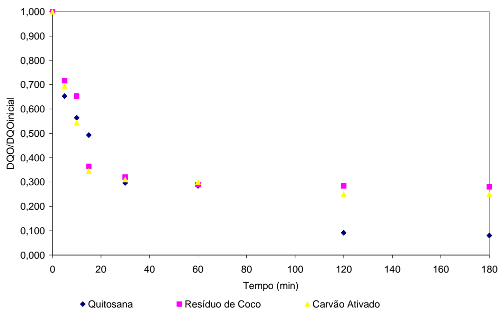
Figura 51: Avaliação dos diferentes adsorventes frente a cinética de remoção de DQO dos efluentes.
