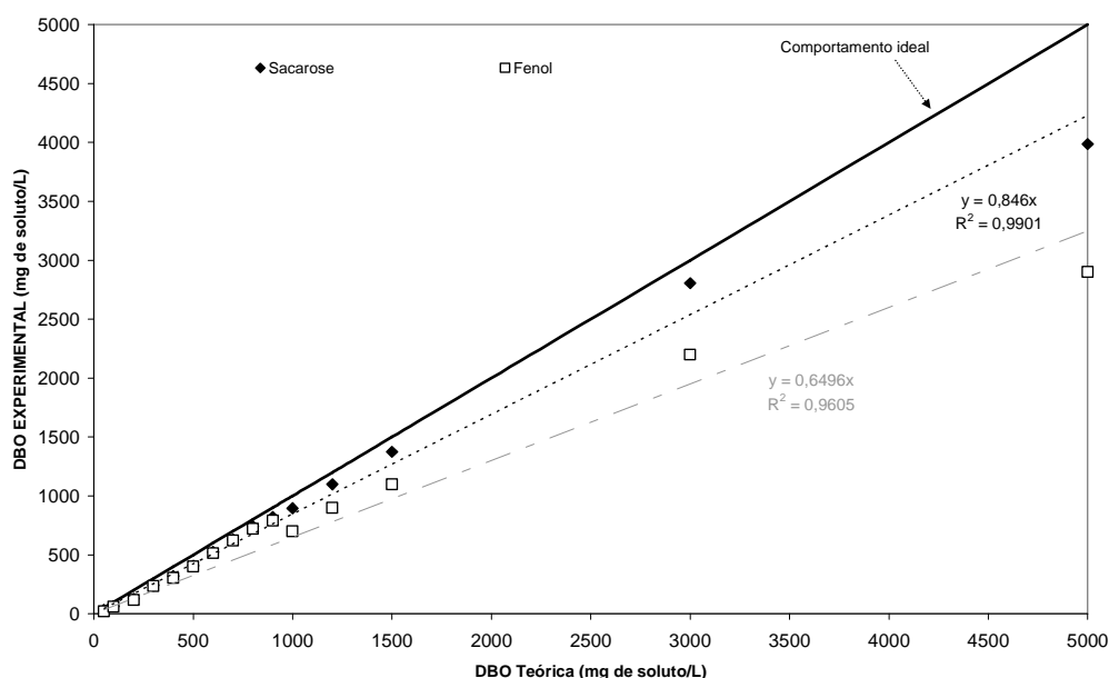
Figura 10: Comparação entre os valores experimentais e previstos para a DBO em efluentes sintéticos.
