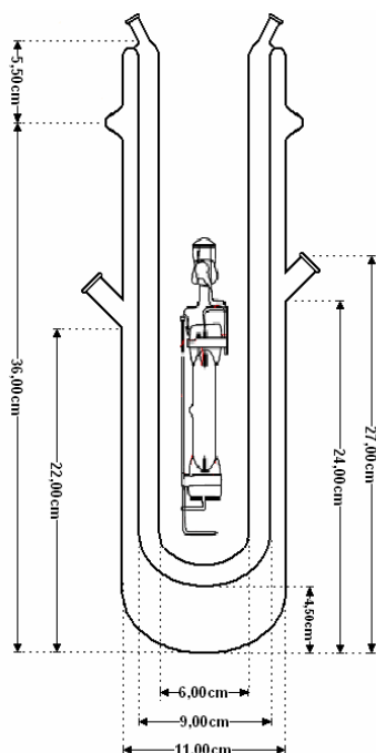
Figura 8: Esquema do reator fotoquímico anular nacional
