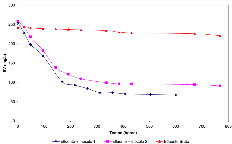
Figura 27: Variação dos sólidos voláteis do efluente bruto e inoculado com esgoto doméstico, ao longo do processo de biodigestão anaeróbia.
