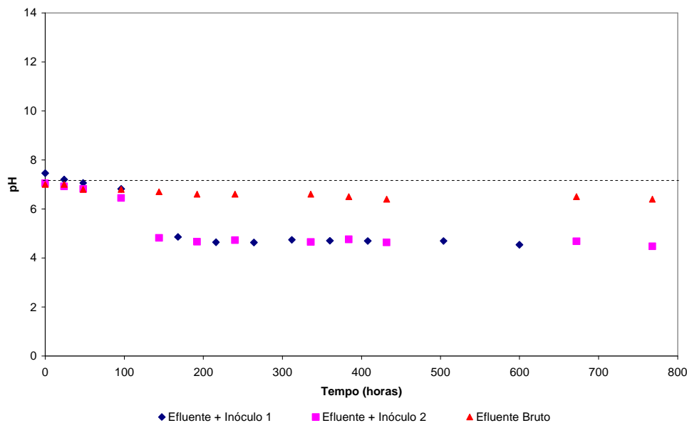
Figura 23: Variação do pH do efluente bruto e inoculado com esgoto doméstico, ao longo do processo de biodigestão anaeróbia.
