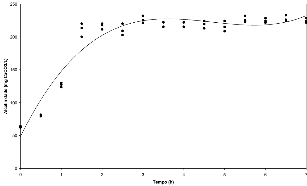
Figura 17: Perfil da alcalinidade ao longo do processo de geração dos efluentes.
