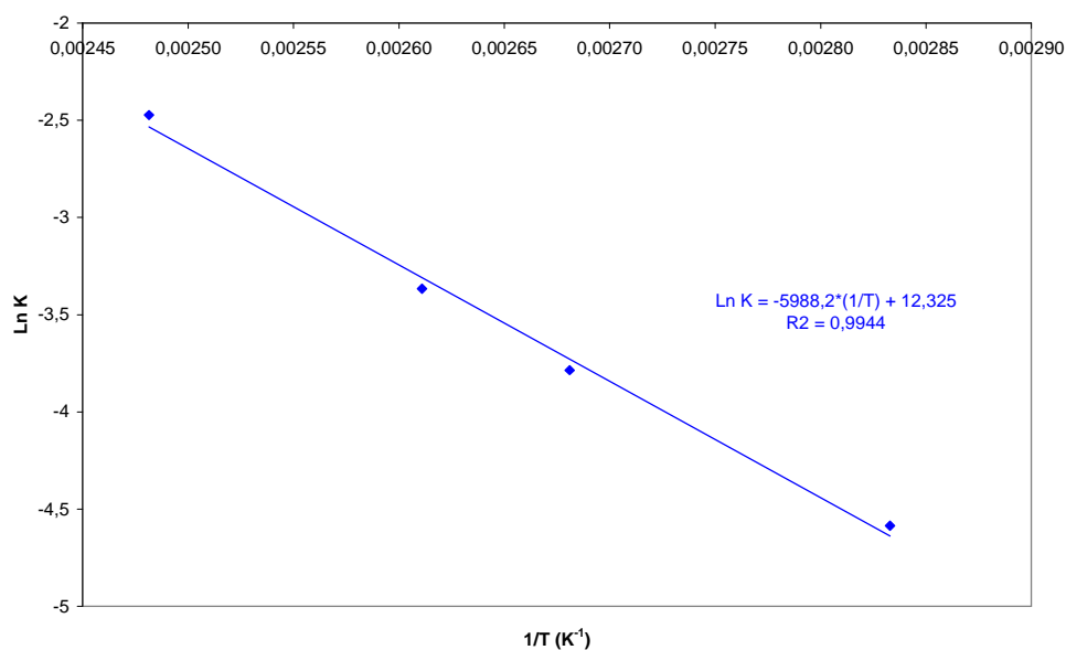
Figura 43: Representação dos parâmetros obtidos na forma de logaritmo natural da constante de velocidade da reação em função do inverso da temperatura.
