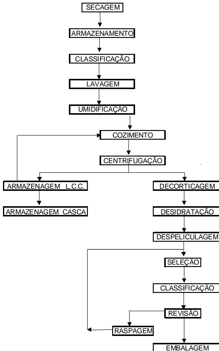
Figura 1: Fluxograma do processo produtivo de beneficiamento da castanha de caju.
