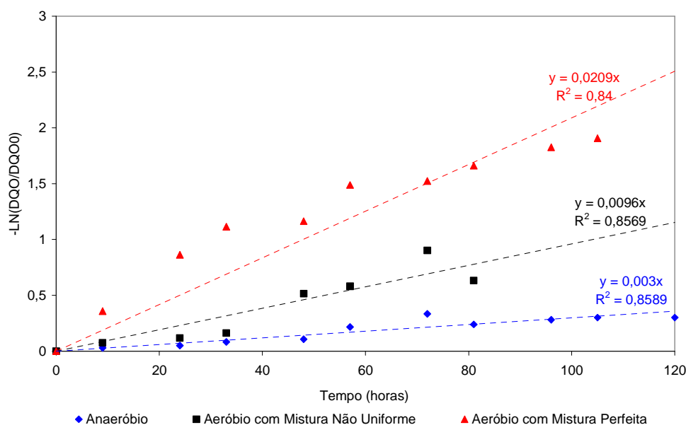
Figura 34: Ajuste linear de uma equação de primeira ordem para a cinética de degradação da Demanda Química de Oxigênio (DQO) do efluente, inoculado com a cepa específica de gorduraklin, ao longo do processo de biodegradação, em diferentes condições operacionais, frente à disponibilidade de oxigênio e efeitos hidrodinâmicos.
