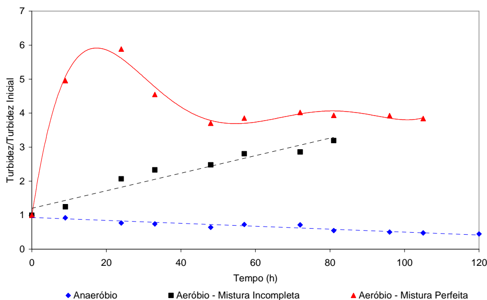
Figura 32: Variação da Turbidez do efluente, inoculado com a cepa específica de ( Gorduraklin® ), ao longo do processo de biodegradação, em diferentes condições operacionais, frente à disponibilidade de oxigênio e efeitos hidrodinâmicos.
