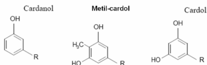
Figura 2: Estrutura química dos principais componentes do LCC.
