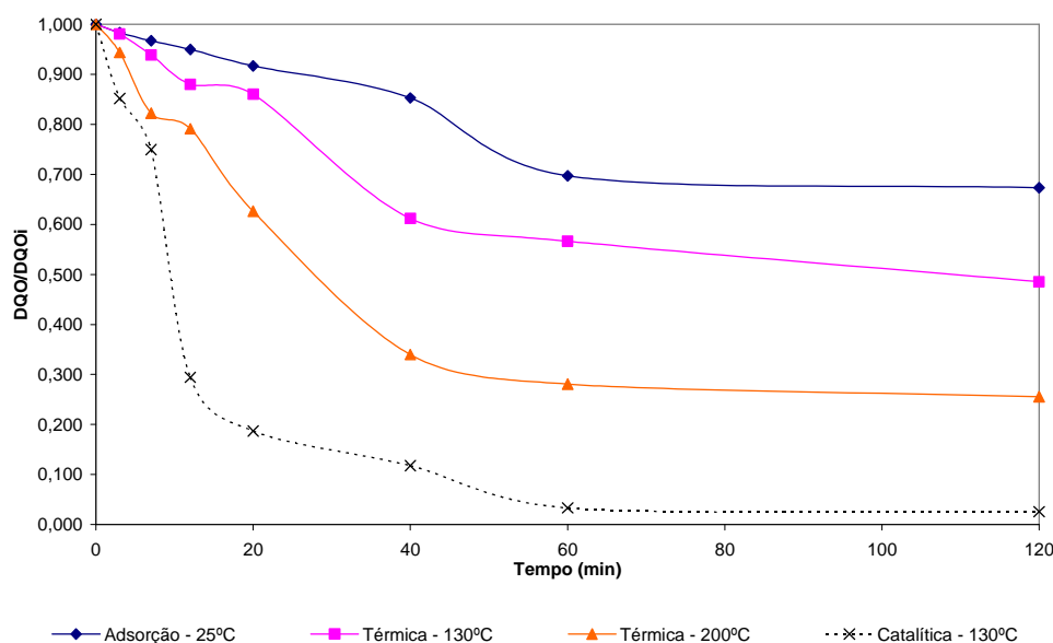
Figura 46: Resultados comparativos das frações residuais de LCC nos processos de adsorção a 25 °C, degradação térmica a 130 e 200 °C e no processo de oxidação catalítica a 130°C.
