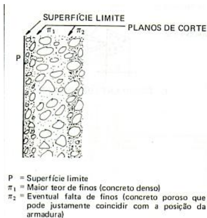
Figura 24 - Efeito parede
