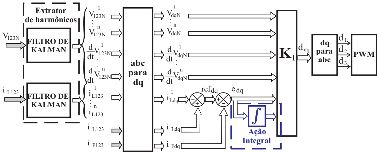
Figura 47: Estrutura do processo de controle LQRNI proposto
