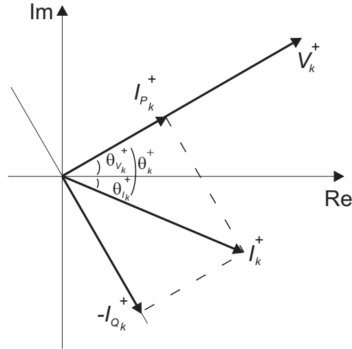
Figura 104: Relações para se obter a corrente fundamental de sequência positiva
