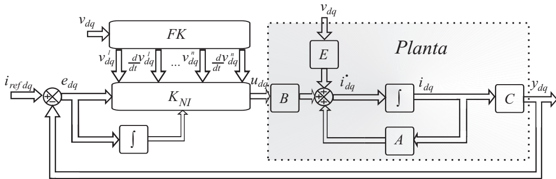
Figura 46: Estrutura do servossistema LQRNI proposto.
