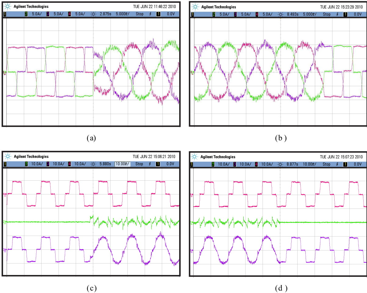
Figura 39: Compensação de harmônicos (a) Correntes trifásicas compensadas (b) Correntes trifásicas compensadas (c) Corrente compensada na fase 1 (d) Corrente compensada na fase 3.
