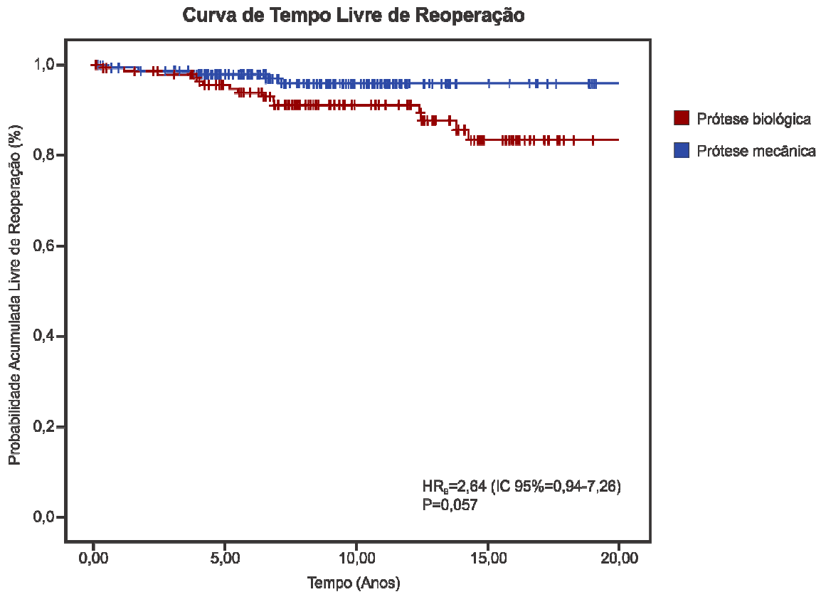
Figura 2 - Curva de Kaplan-Meier para avaliar tempo livre de reoperação.
