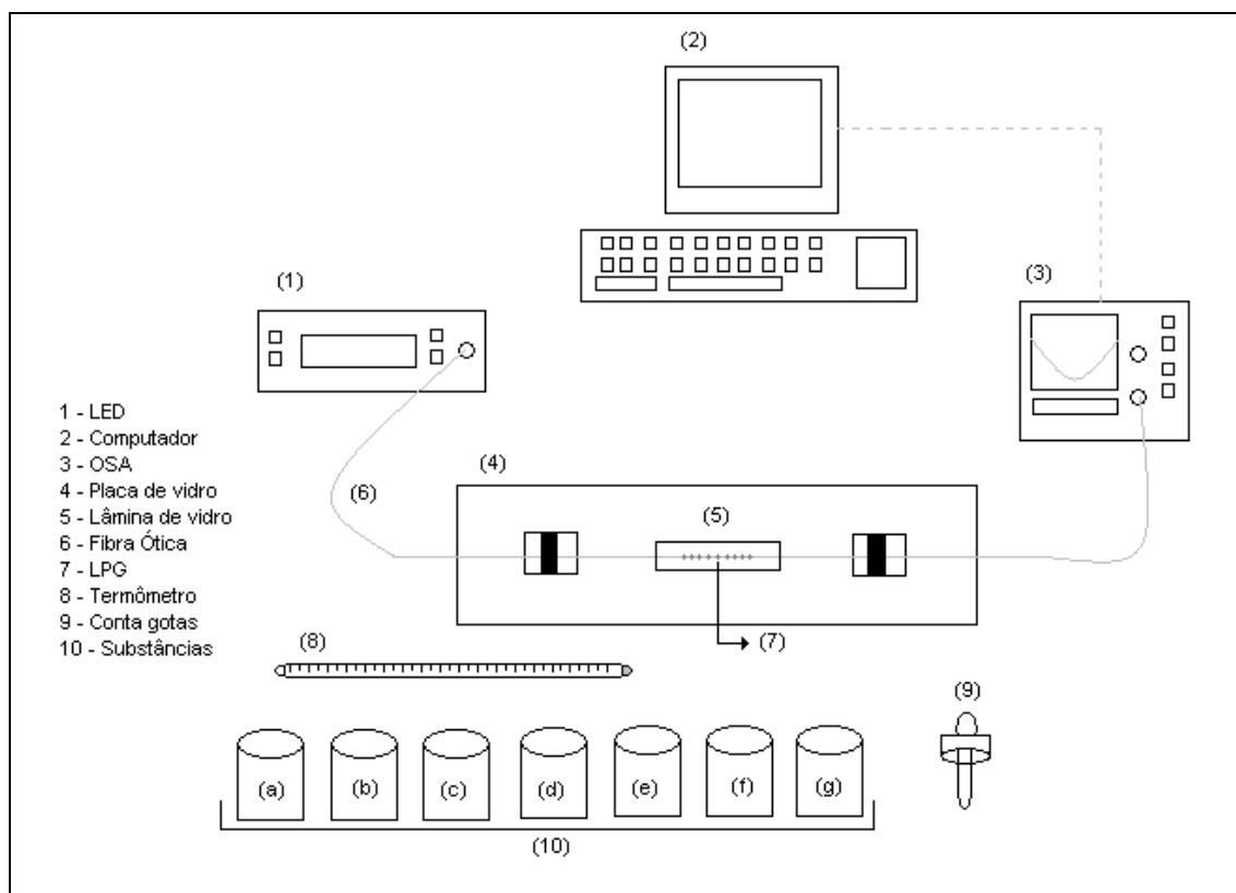
Figura 9 – Diagrama esquemático do sistema e dos materiais utilizados para o processo de caracterização das LPG.
