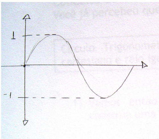
Figura 18: Esboço do Gráfico das Funções Seno e Cosseno
