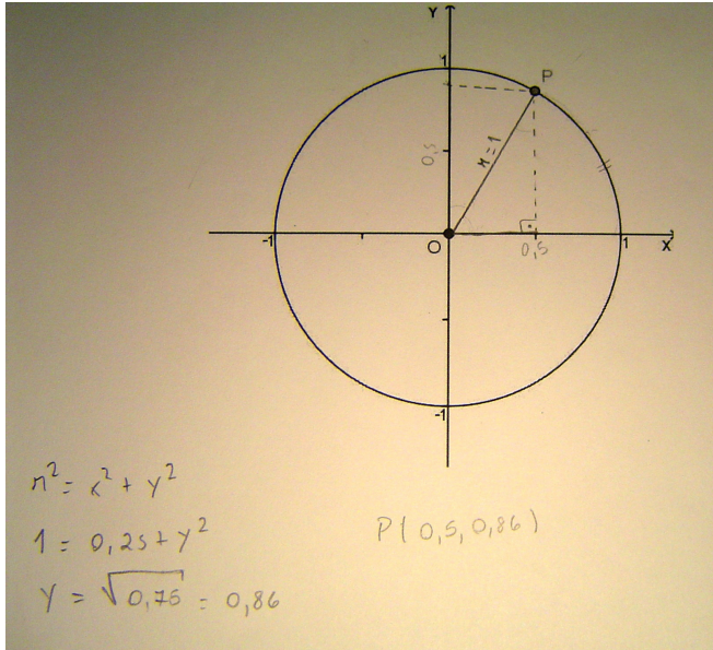
Figura 15: Círculo Trigonométrico - Segundo Encontro
