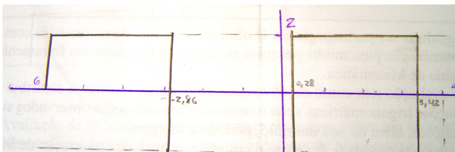
Figura 20: Gráfico da Função 2
