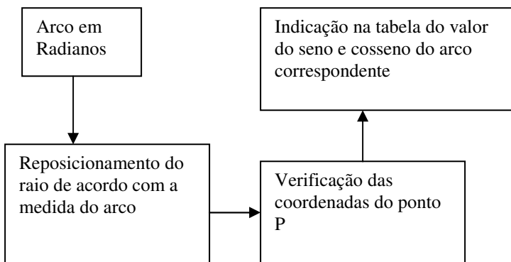
Figura 12: Mudanças de registro no círculo trigonométrico
