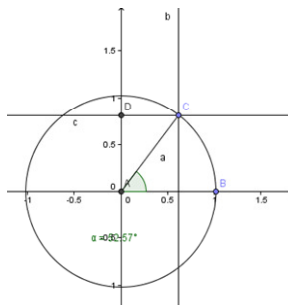
Figura 5: Alguns registros da Função f(x)=\cos(x)
