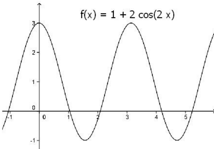
Figura 9: Registro gráfico e algébrico da função
