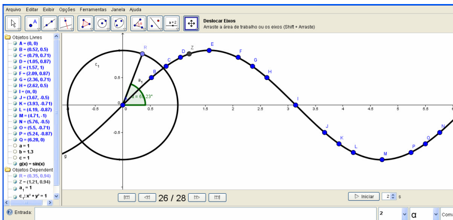
Figura 17: Círculo Trigonométrico
