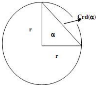
Figura 3: A função “ \text{crd}(x) ”
