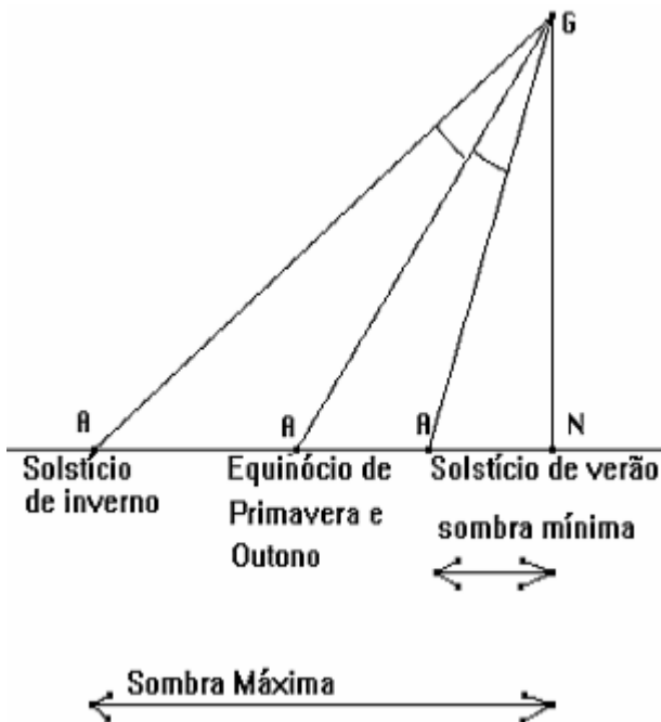
Figura 2: Representação do relógio de sol (gnômon)
