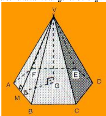
Figura 1: Pirâmide Regular e a relação seqt
