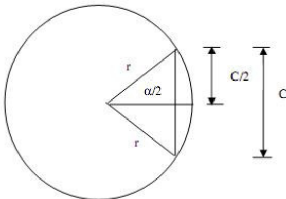
Figura 4: A relação jiva sobre a circunferência
