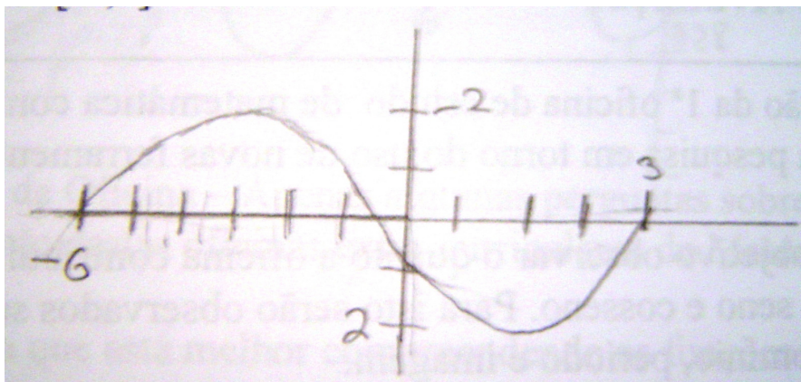
Figura 19: Gráfico da Função
