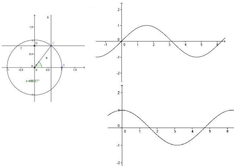
Figura 8: Círculo trigonométrico e o gráfico das funções seno e cosseno
