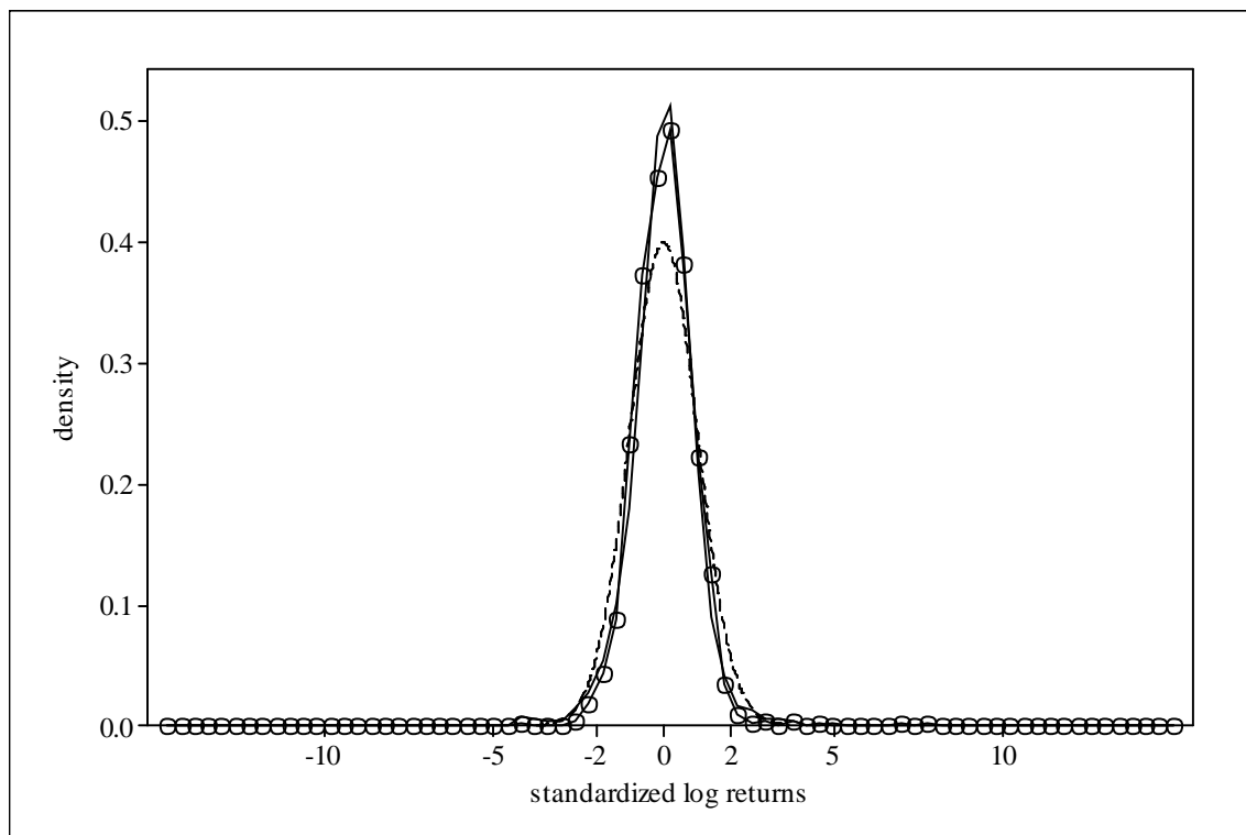
Figura 7. Funções densidade de probabilidade da série de retornos do índice Bovespa (linha contínua) e da série de retornos gerada pelo modelo (círculos abertos) com \lambda = 1 , \kappa = 9 , e \mu = 2 \times 10^{10} . A natureza leptocúrtica da série empírica é replicada pelo modelo. Uma f.d.p. Gaussiana (linha tracejada) é apresentada no gráfico para comparação
