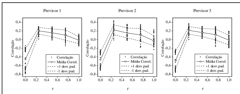
Figura 5 – Relação entre o parâmetro \tau e o desempenho em termos de convergência do SC-AG.
