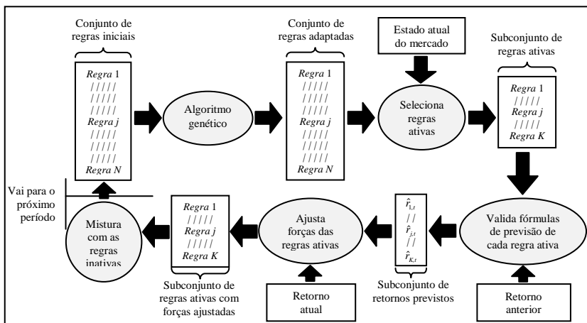
Figura 1 – Ilustração do processo de previsão do SC-AG.
