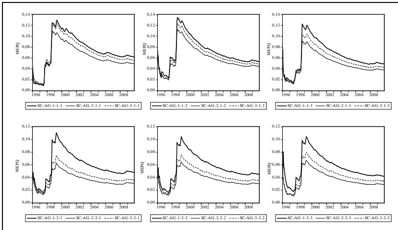
Figura 11 – Comparativo das médias recursivas acumuladas dos erros de previsão ao quadrado, por predictor do SC-AG.
