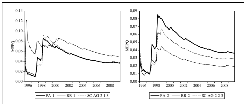
Figura 13 – Comparativo das médias recursivas acumuladas dos erros de previsão ao quadrado, por algoritmo preditivo.
