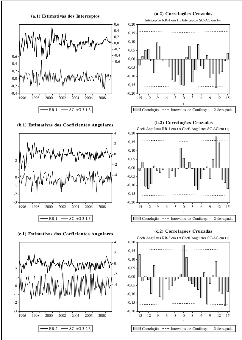
Figura 7 – Comparativo dos parâmetros de previsão estimados recursivamente pelos modelos de regressões recursivas e SC-AG.
