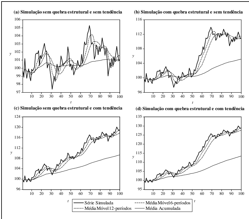
Figura 3 – Ilustração dos indicadores de médias móveis a partir de séries temporais simuladas.
