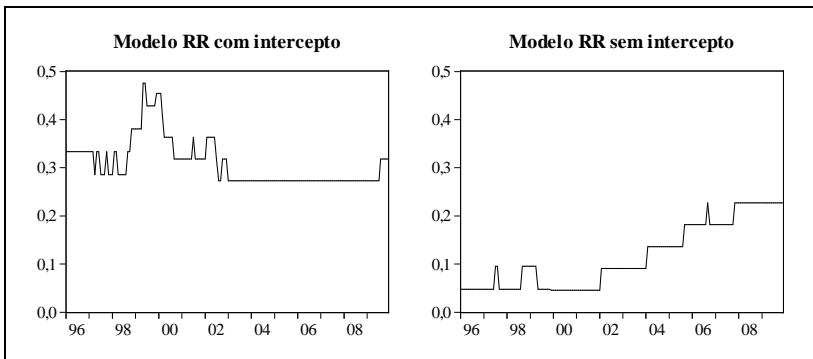
Figura 10 – Evolução do percentual de bits estatisticamente significantes ao nível de 10% nas estimativas dos modelos RR.
