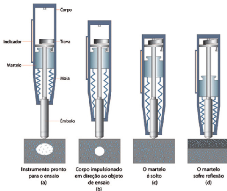
Figura 2-9 Diagrama de operação do esclerômetro de reflexão (Mehta & Monteiro, 2008)
