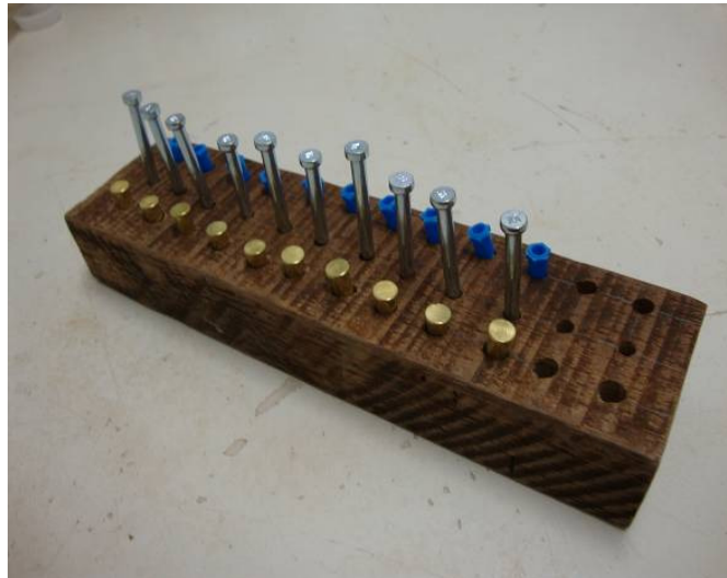
Figura 3-23 – Gabarito para pinos e cartuchos
