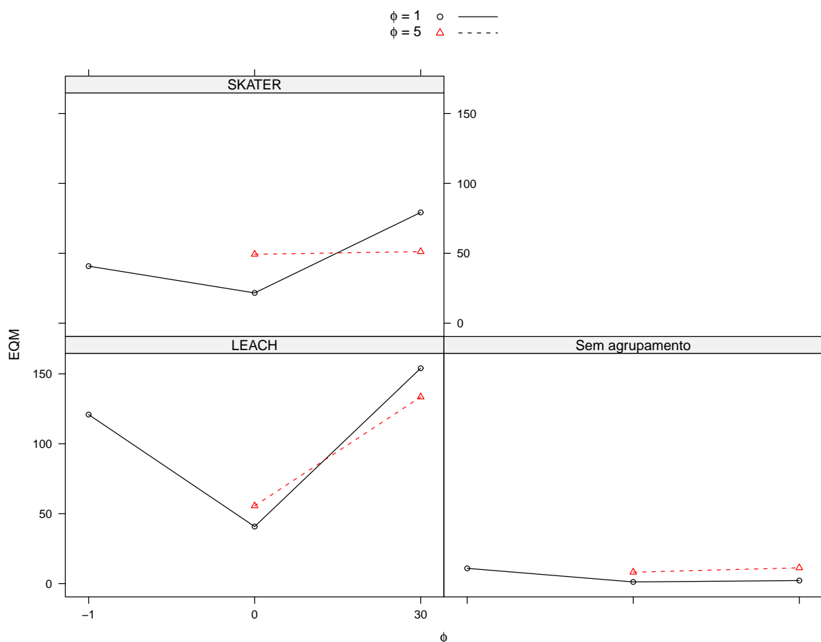
Figura 4.1: Erro quadrático médio do estimador de \phi pelo kriging simples
