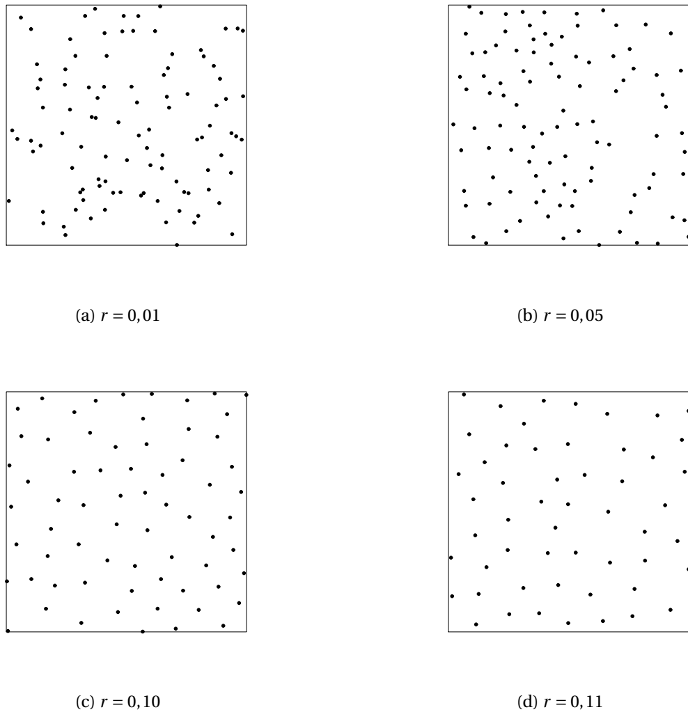
Figura 3.5: Exemplos de um processo pontual de SSI com n = 100 e T = 1.000
