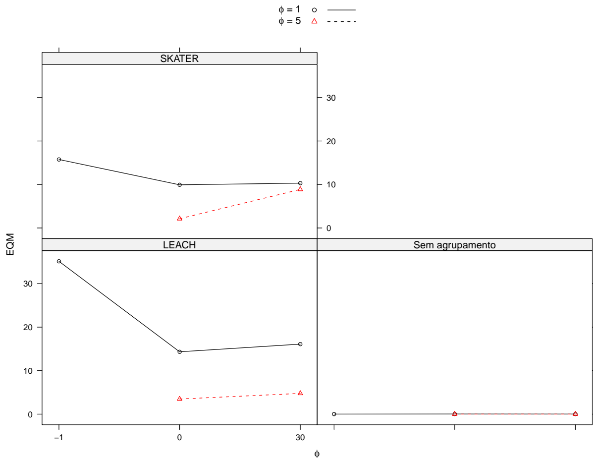
Figura 4.3: Erro quadrático médio do estimador de \phi pelo kriging bayesiano
