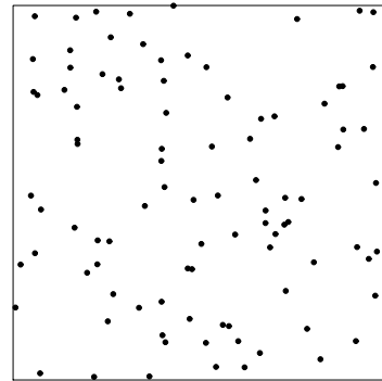
(b) n = 95 pontos
