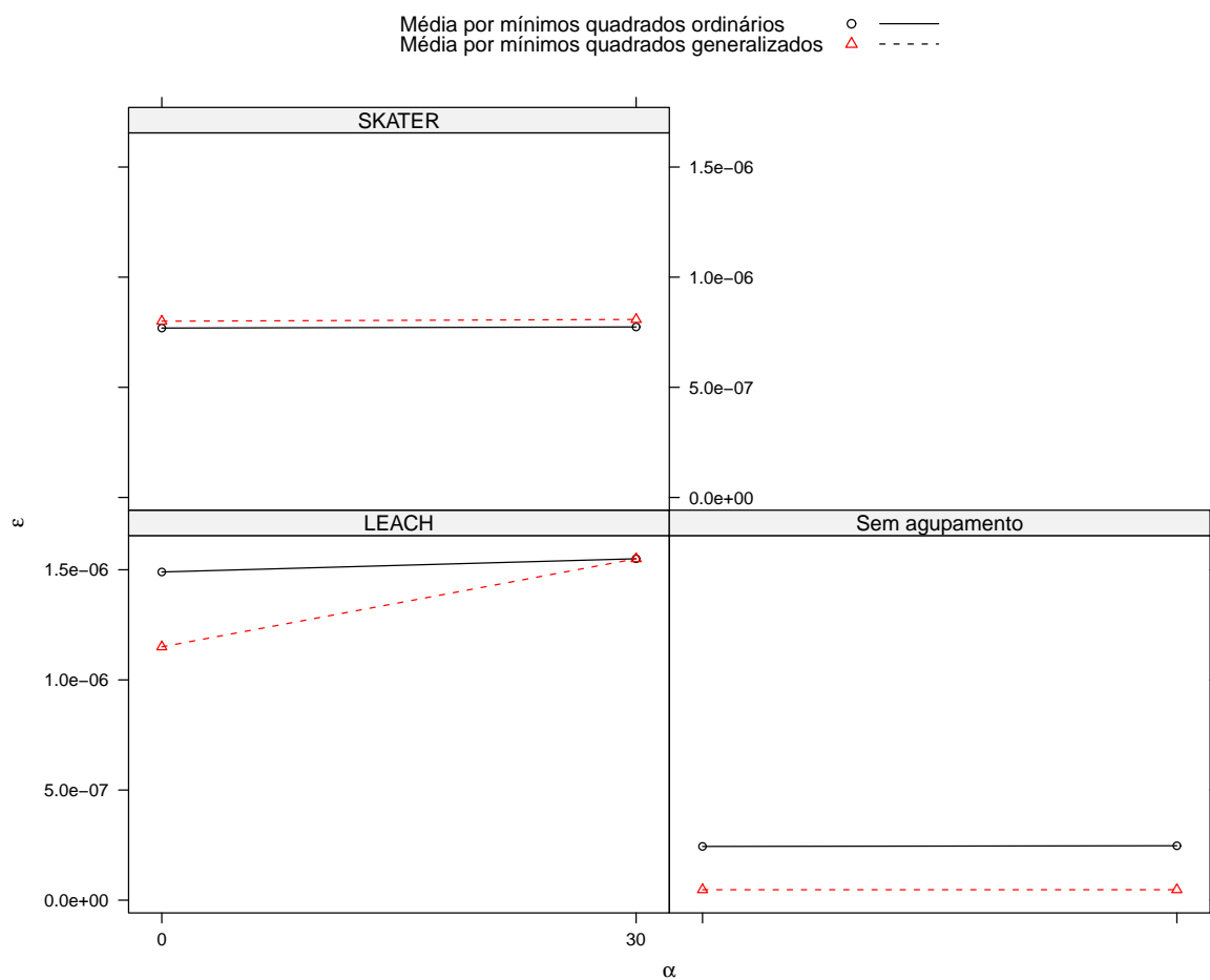
Figura 4.17: Erro de reconstrução por kriging simples pelos parâmetros considerando a média para \phi = 5
