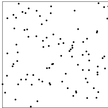
(a) n = 94 pontos
