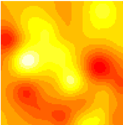
(b) Reconstrução por kriging simples
