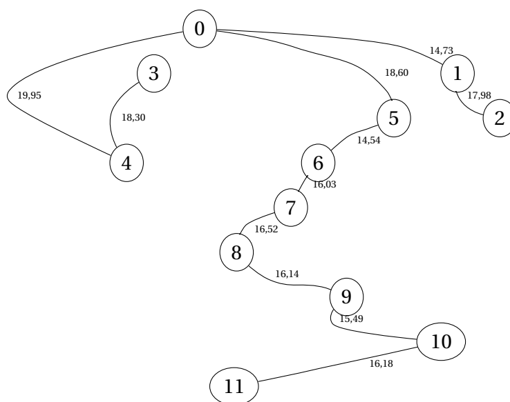
Figura 2.13: Árvore Geradora Mínima do grafo de sensores da figura 2.12
