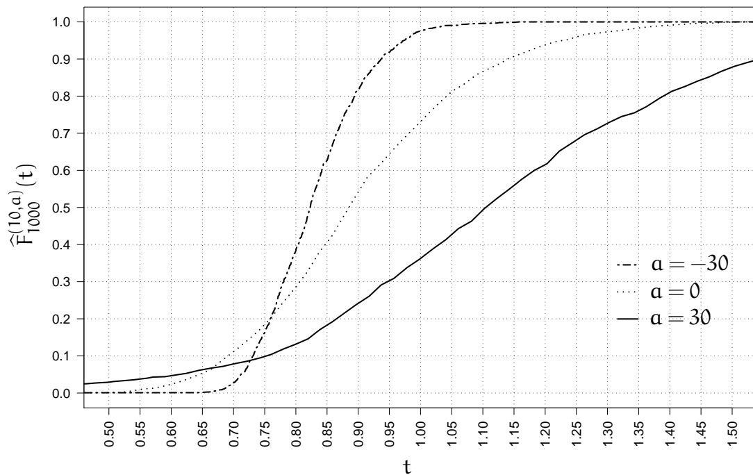
Figura 4.15: Função empírica das variáveis \chi^{(10,a)}
