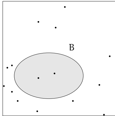
Figura 2.7: Região de contagem N(B) = 2
