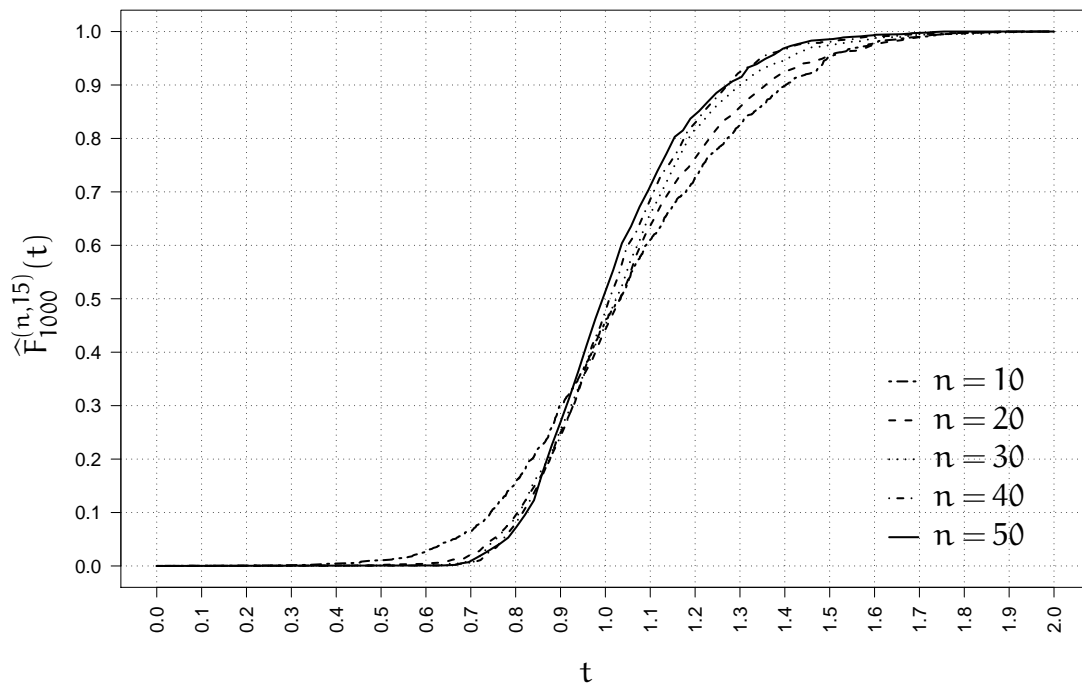
Figura 4.12: Função empírica das variáveis X^{(n,15)}
