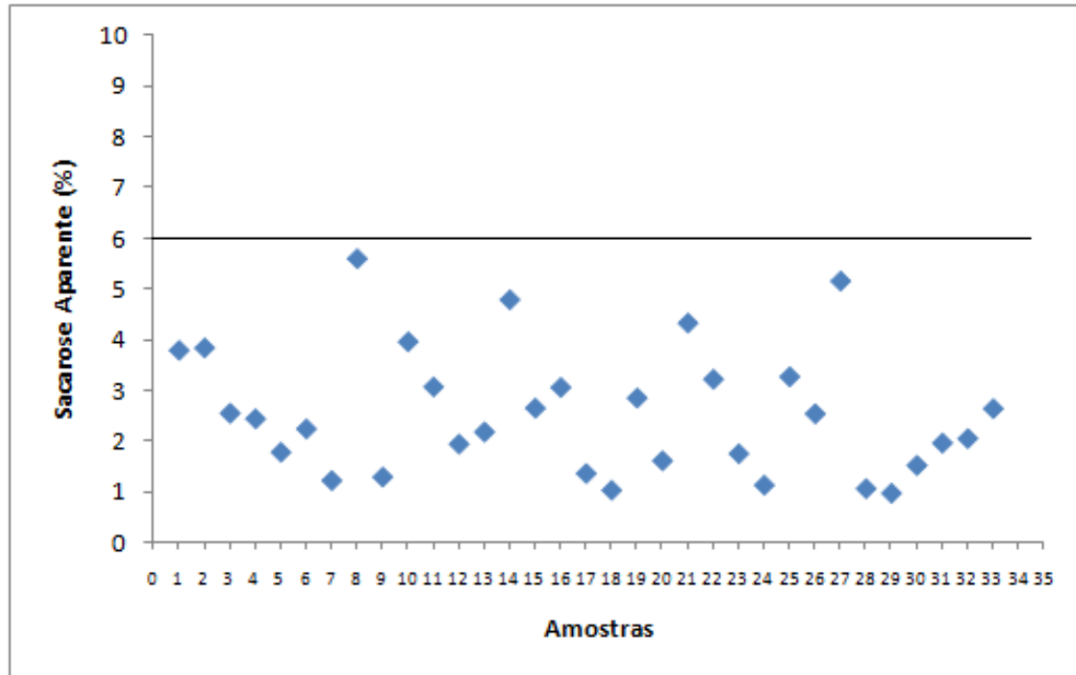
Figura 14. Valores de sacarose aparente em amostras mel de abelhas Apis melliferas L. da microrregião de Pires do Rio/GO, e o limite de 6 % estabelecido pela Instrução Normativa nº 11 (BRASIL, 2000)
