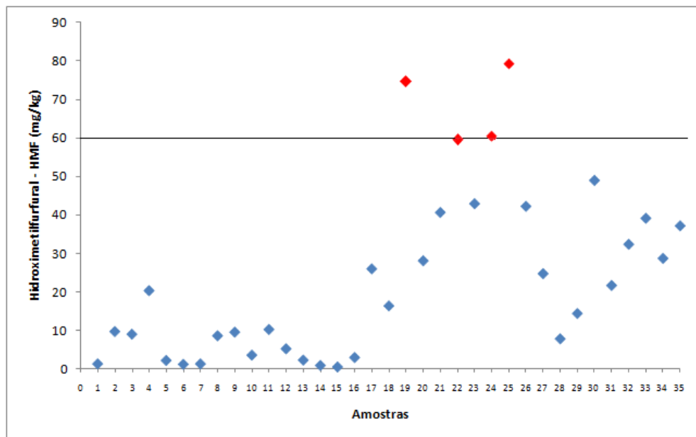
Figura 11. Valores de hidroximetilfurfural em amostras mel de abelhas Apis melliferas L. da microrregião de Pires do Rio/GO, e o limite de 60 mg/kg estabelecido pela Instrução Normativa nº 11 (BRASIL, 2000)
