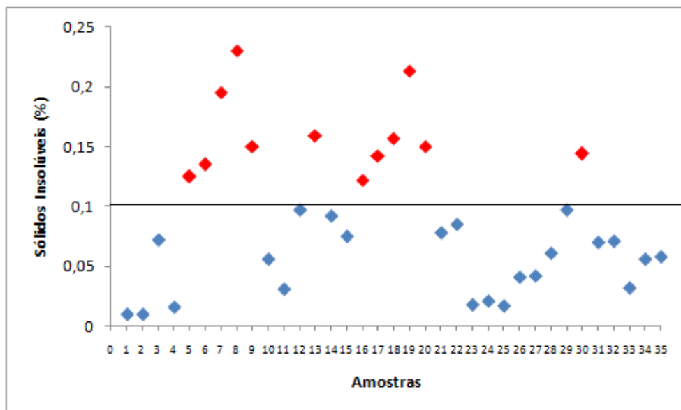
Figura 16. Valores de sólidos insolúveis em amostras mel de abelhas Apis melliferas L. da microrregião de Pires do Rio/GO, e o limite de 0,1% estabelecido pela Instrução Normativa nº 11 (BRASIL, 2000)
