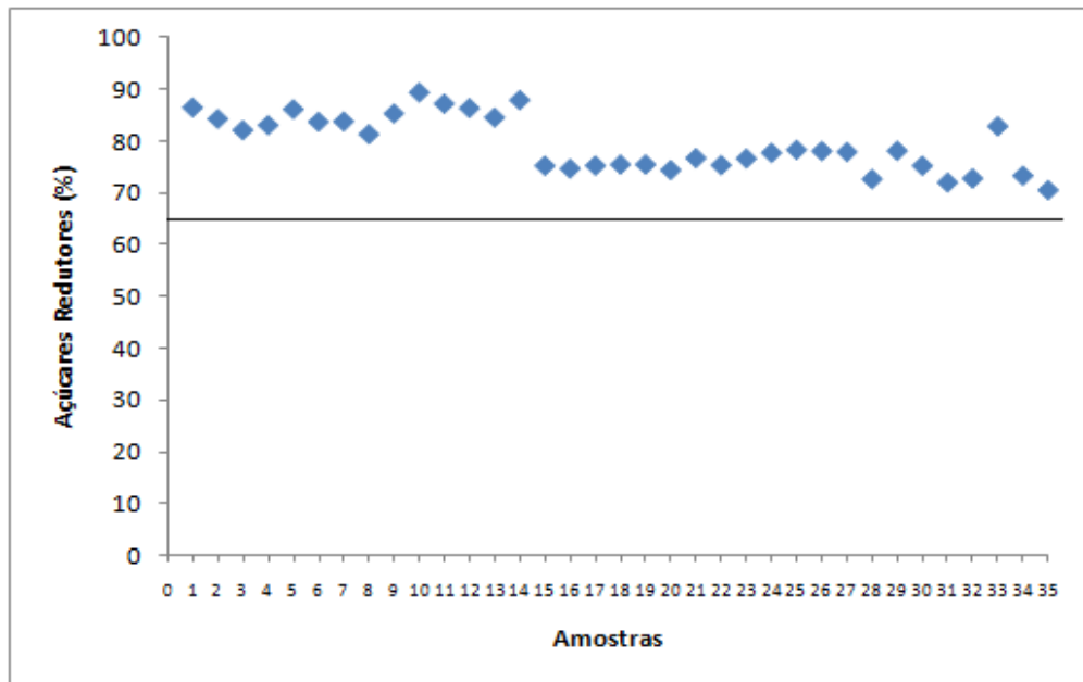
Figura 13. Valores de açúcares redutores em amostras mel de abelhas Apis mellifera L. da microrregião de Pires do Rio/GO, e o limite mínimo de 65% estabelecido pela Instrução Normativa nº 11 (BRASIL, 2000)
