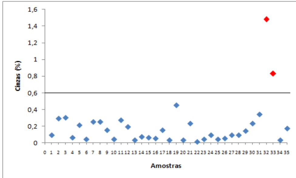
Figura 15. Valores de cinzas em amostras mel de abelhas Apis melliferas L. da microrregião de Pires do Rio/GO, e o limite de 0,6 % estabelecido pela Instrução Normativa nº 11 (BRASIL, 2000)
