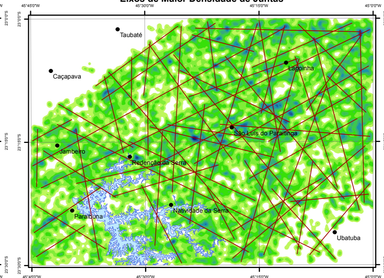
Figura 18 - Mapa de Densidade de Cruzamentos de Lineamentos Estruturais e Densidade de Juntas e respectivos eixos de maior densidade.
