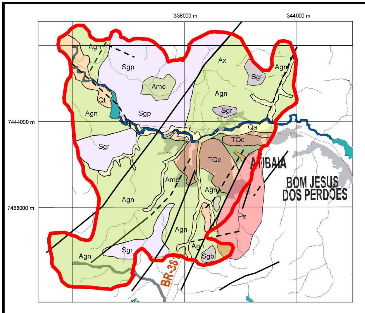
Figura 4.3a: Mapa geológico da região do município de Atibaia (OLIVEIRA et al. 1985 e SILVA, 2007).
