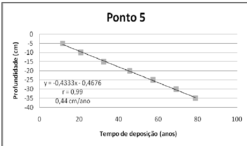
Figura 7.23: Relação entre a profundidade da coluna sedimentar e o tempo de deposição dos sedimentos para o ponto 5
