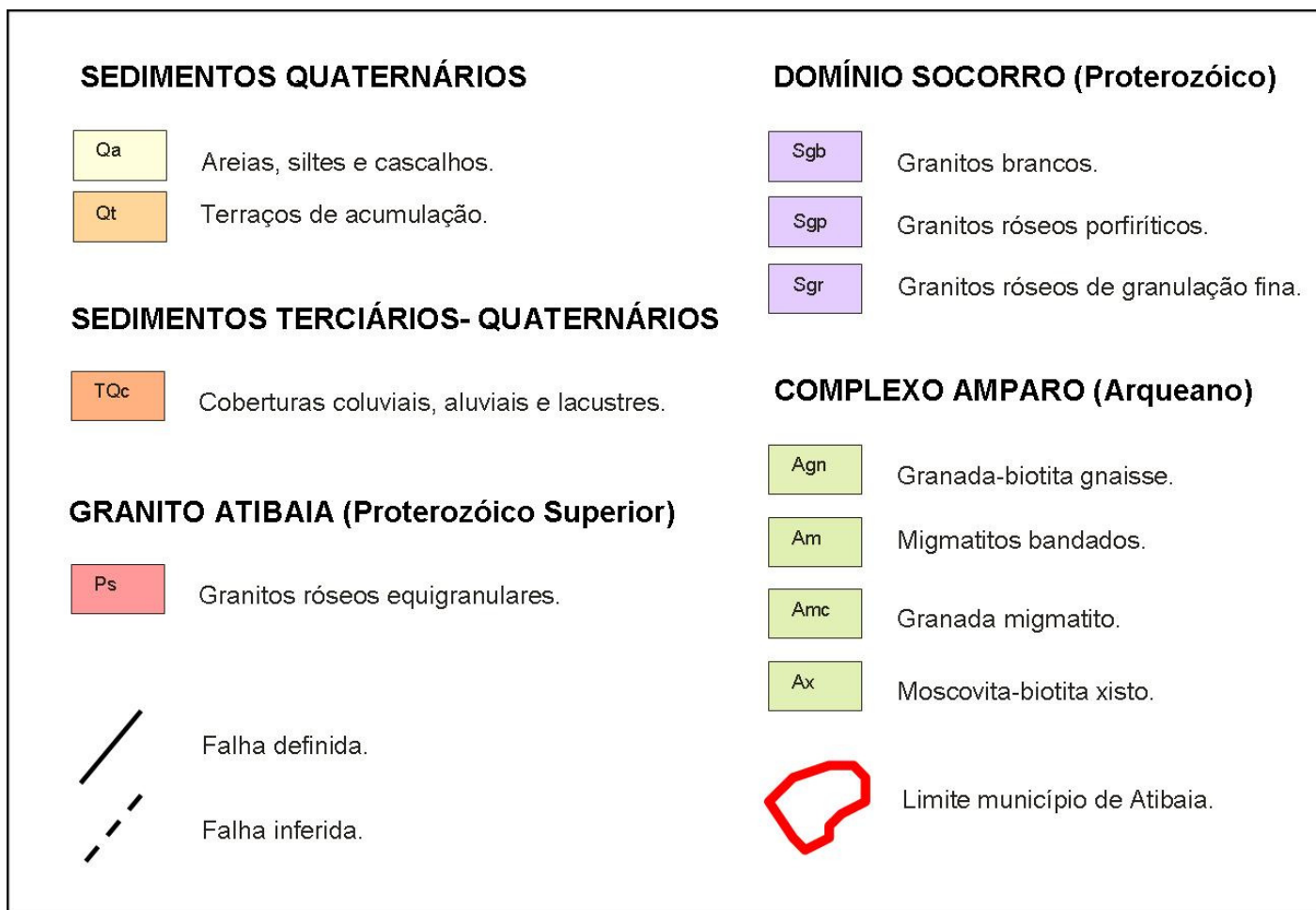
Figura 4.3b: Legenda do mapa geológico da região do município de Atibaia (OLIVEIRA et al. 1985 e SILVA, 2007).
