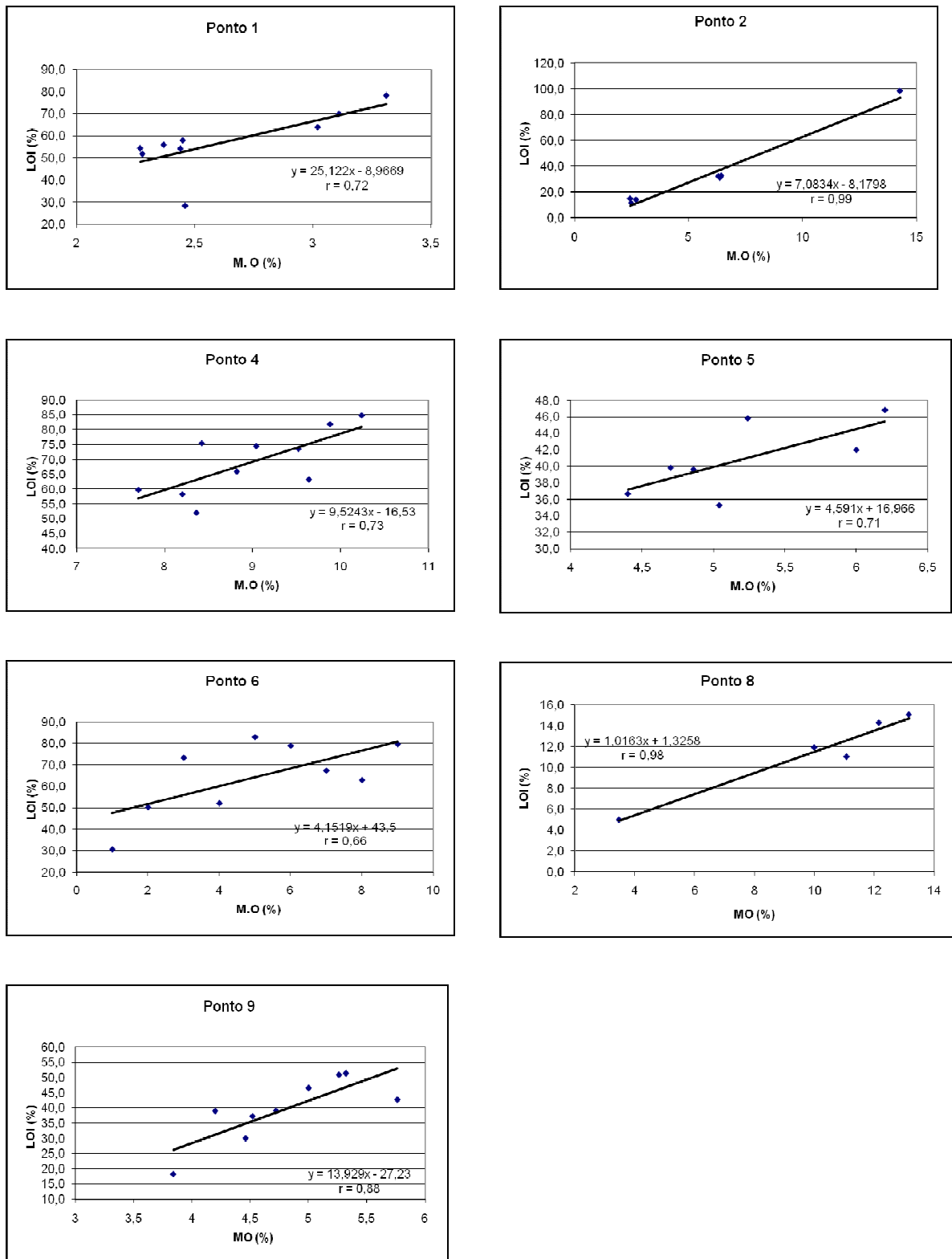
Figura: 6.5: Relação entre LOI e Matéria Orgânica em % nos sedimentos dos testemunhos.
