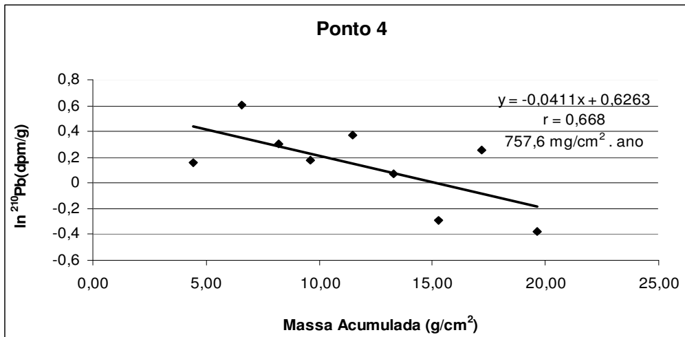
Figura 7.13: Variação da atividade do ^{210}\text{Pb} “não produzido” em função da massa seca acumulada por unidade de área do perfil 4.
