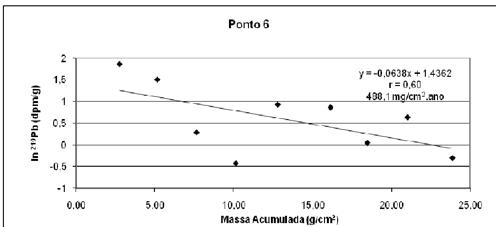
Figura 7.15: Variação da atividade do ^{210}\text{Pb} “não produzido” em função da massa seca acumulada por unidade de área do perfil 6.
