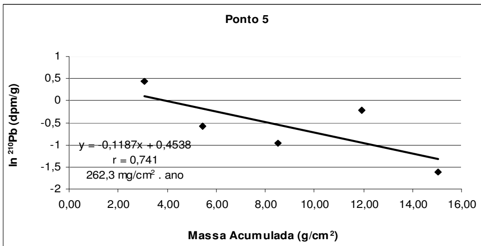
Figura 7.14: Variação da atividade do ^{210}\text{Pb} “não produzido” em função da massa seca acumulada por unidade de área do perfil 5.
