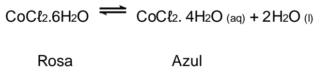
Figura 2: Deslocamento do equilíbrio químico \text{CoCl}_2 \cdot 6\text{H}_2\text{O} / \text{CoCl}_2 \cdot 4\text{H}_2\text{O} : (a) sob hidratação, maior concentração de \text{CoCl}_2 \cdot 6\text{H}_2\text{O} ; (b) após secagem, maior concentração de \text{CoCl}_2 \cdot 4\text{H}_2\text{O} (< www.scielo.br/img/revistas/qn/v27n6/22294f4.jpg >).
